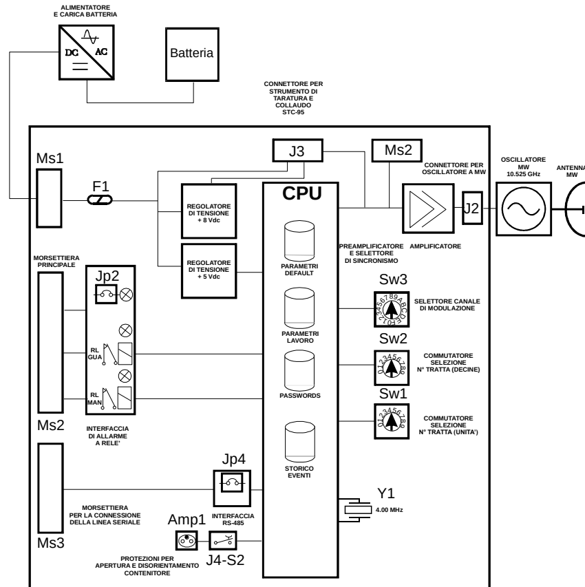
Schema a blocchi Coral Plus Trasmettitore
