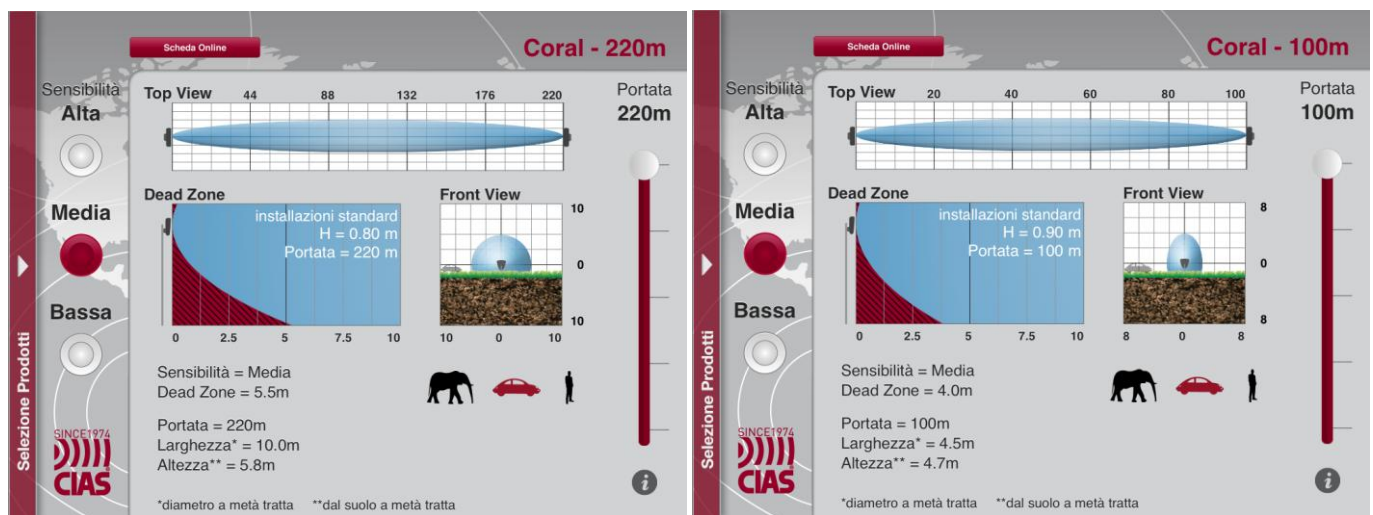
Dimensione del fascio e zone d'ombra usando antenna parabolica di serie
