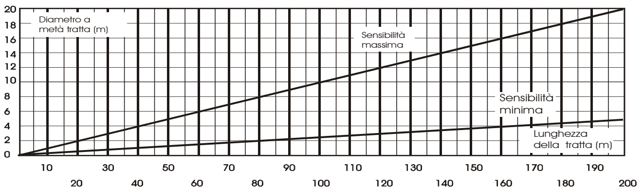
Figura 4 Diametro della zona sensibile a metà tratta per ERMox 482/ 80-120-200
