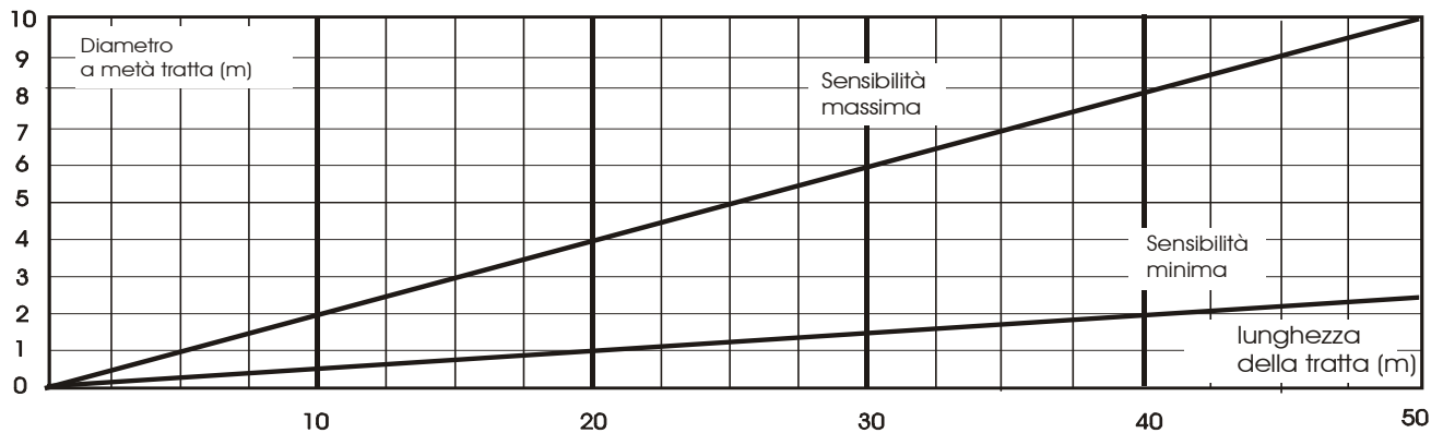
Figura 3 Diametro della zona sensibile a metà tratta per ERMox 482/ 50
