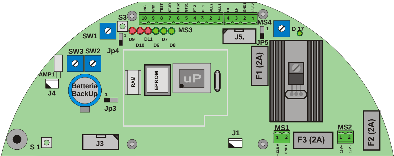
Figura 9 Disposizione topografica dei componenti nel circuito Rx
