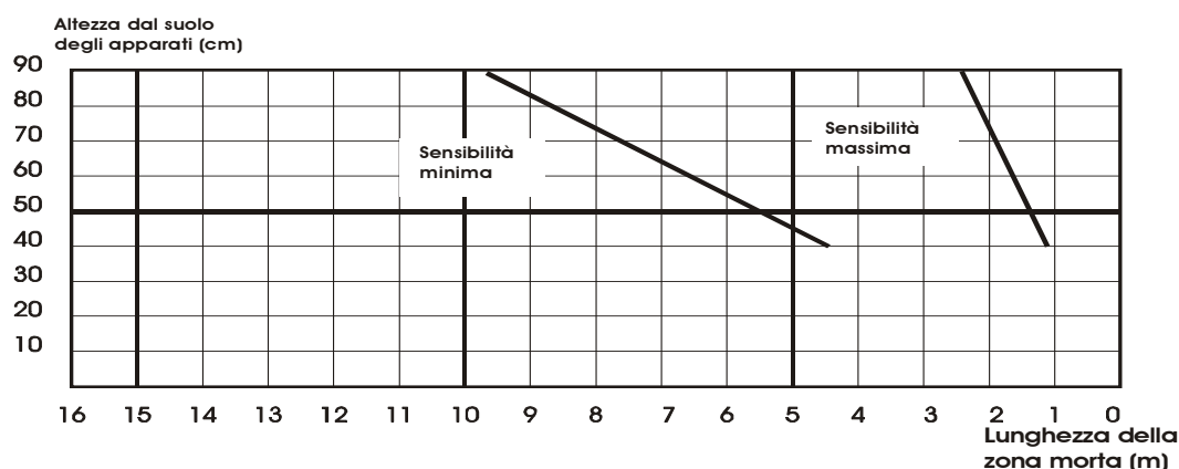
Figura 6 Lunghezza della zona morta in prossimità degli apparati in funzione dell'altezza dal centro degli stessi al suolo per ERMO 482X PRO. 80-120-200
