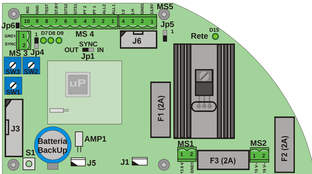
Figura 8 Disposizione topografica dei componenti nel circuito Tx
