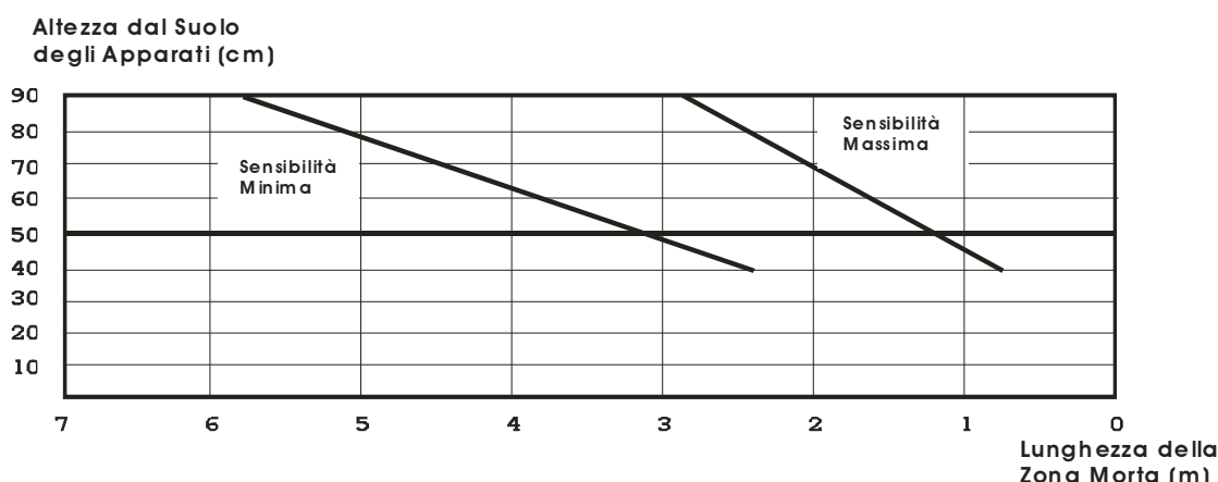
Figura 5 Lunghezza della zona morta in prossimità degli apparati in funzione dell'altezza dal centro degli stessi al suolo per ERMO 482X PRO. 50
