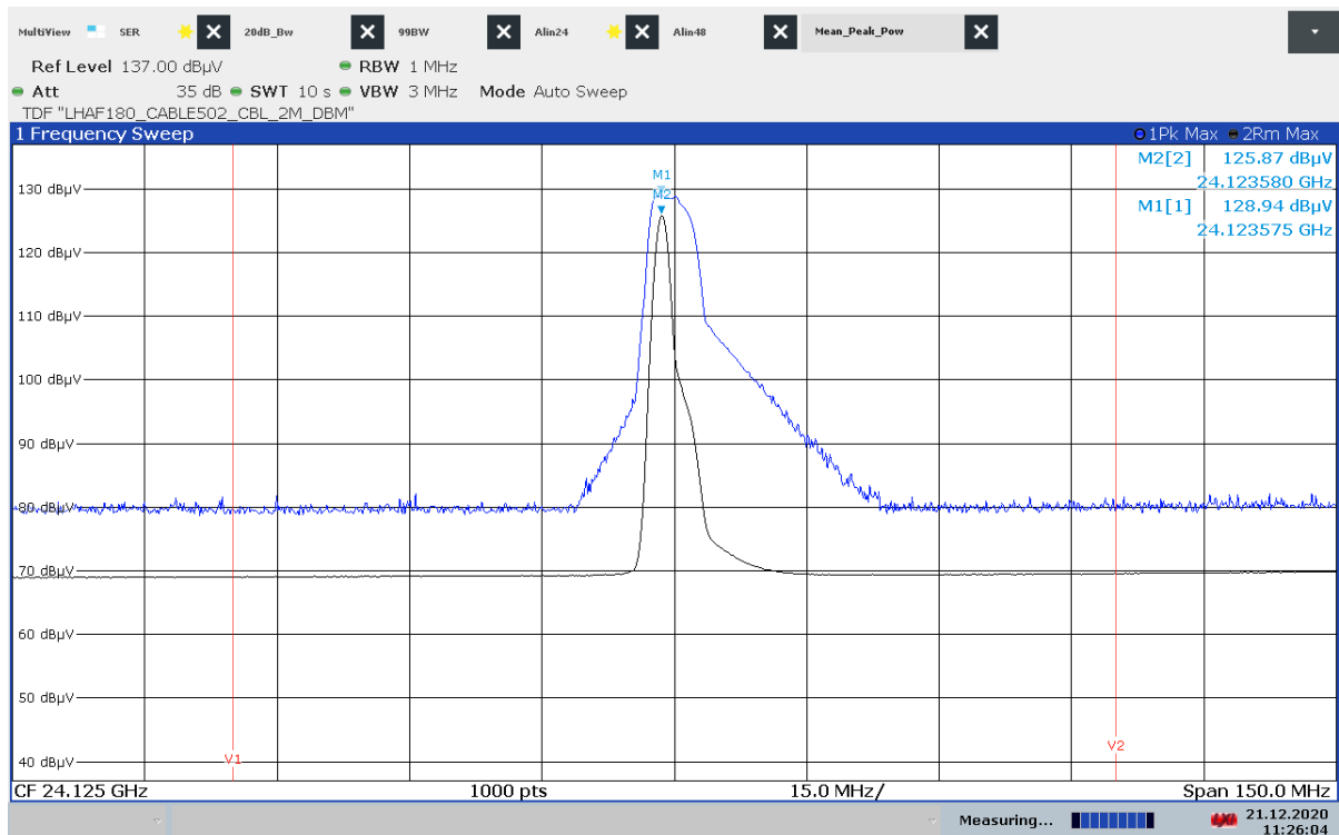
Plot 25: +30 °C, V_{\text{nom}}
