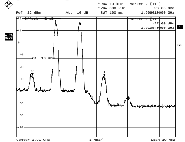
EDGE Upper Bandedge - Uplink
