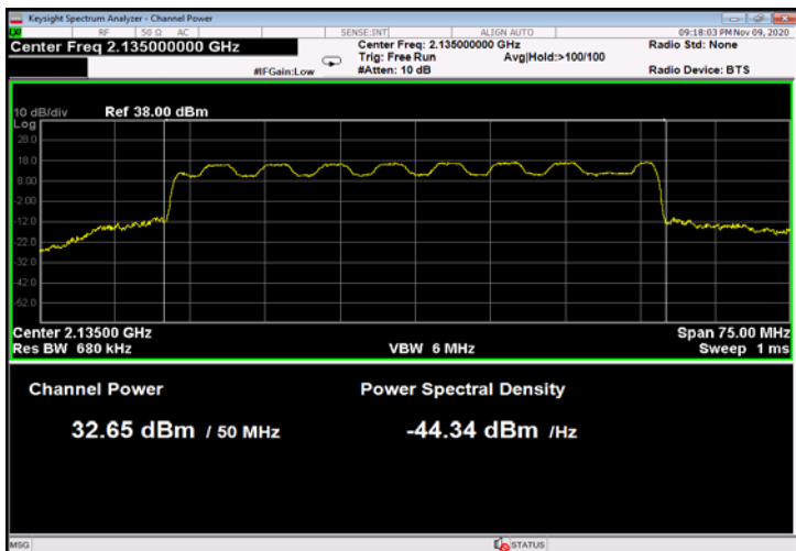
Figure 61: 16QAM 50MHz B.W.; 2135.0MHz, 30kHz
