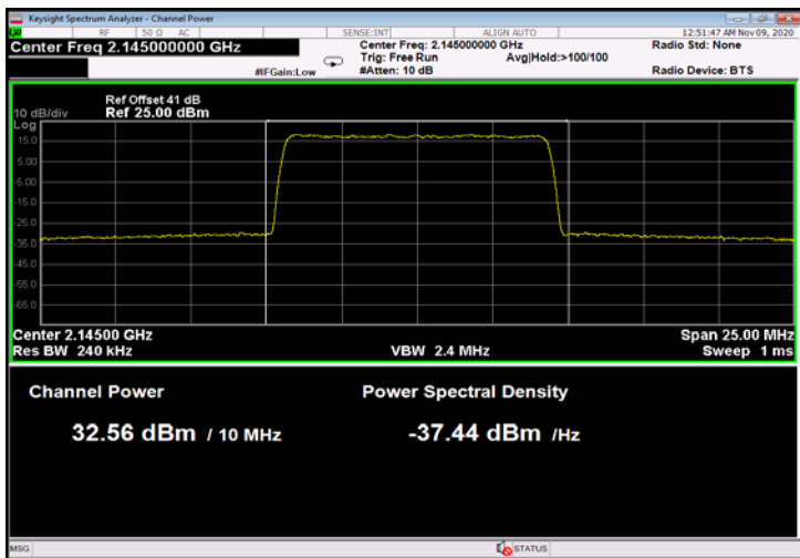
Figure 85: 64QAM 10MHz B.W.; 2145MHz, 30kHz
