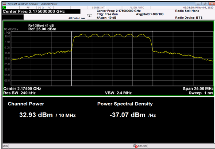
Figure 21: 16QAM 10MHz B.W.; 2175.0MHz, 15kHz
