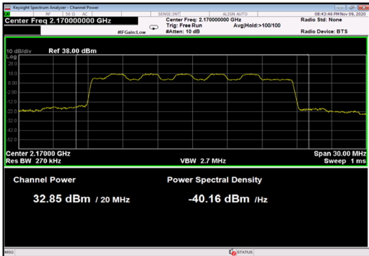
Figure 41: 16QAM 20MHz B.W.; 2170.0MHz, 60kHz
