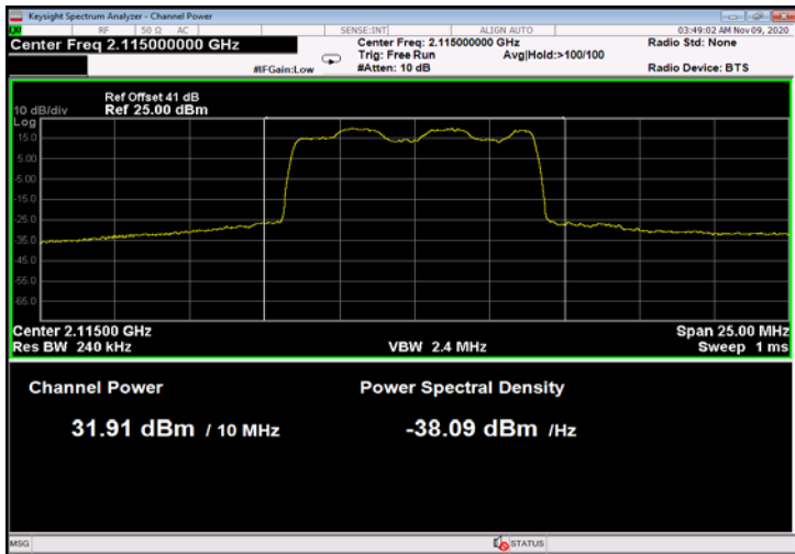
Figure 17: 16QAM 10MHz B.W.; 2115.0MHz, 60kHz
