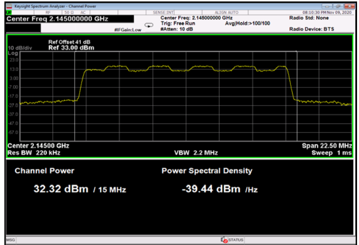
Figure 28: 16QAM 15MHz B.W.; 2145.0MHz, 30kHz
