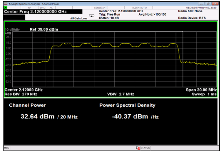
Figure 34: 16QAM 20MHz B.W.; 2120.0MHz, 30kHz
