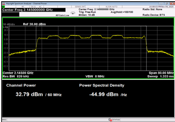
Figure 71: 16QAM 60MHz B.W.; 2145.0MHz, 30kHz
