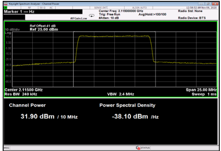
Figure 82: 64QAM 10MHz B.W.; 2115.0MHz, 30kHz
