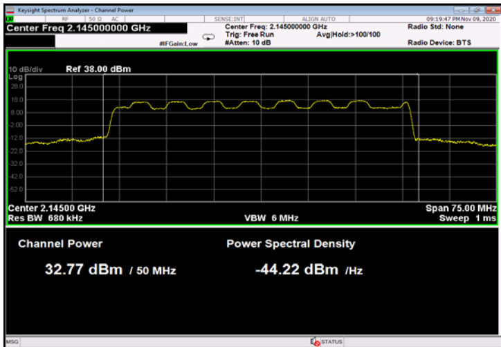
Figure 65: 16QAM 50MHz B.W.; 2145.0MHz, 60kHz
