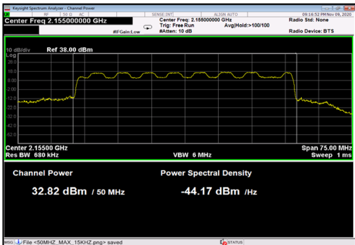
Figure 67: 16QAM 50MHz B.W.; 2155.0MHz, 30kHz
