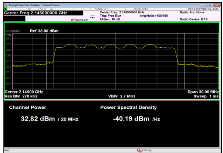
Figure 38: 16QAM 20MHz B.W.; 2145.0MHz, 60kHz
