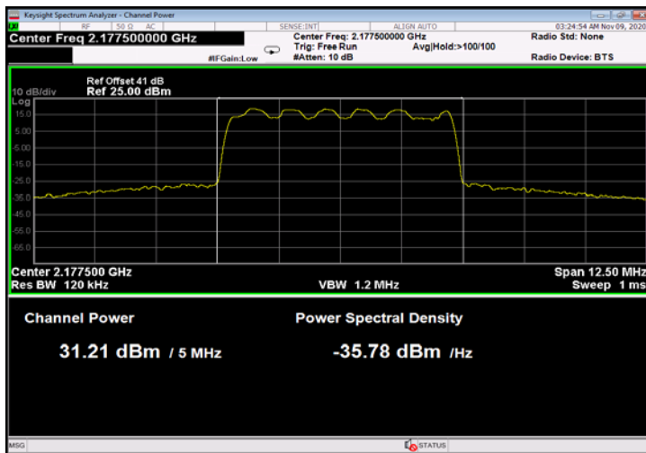
Figure 13: 16QAM 5MHz B.W.; 2177.5MHz, 15kHz
