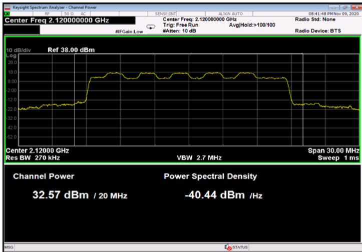
Figure 35: 16QAM 20MHz B.W.; 2120.0MHz, 60kHz
