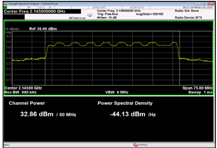
Figure 64: 16QAM 50MHz B.W.; 2145.0MHz, 30kHz
