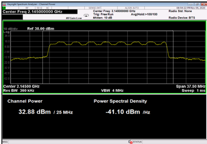
Figure 47: 16QAM 25MHz B.W.; 2145.0MHz, 60kHz
