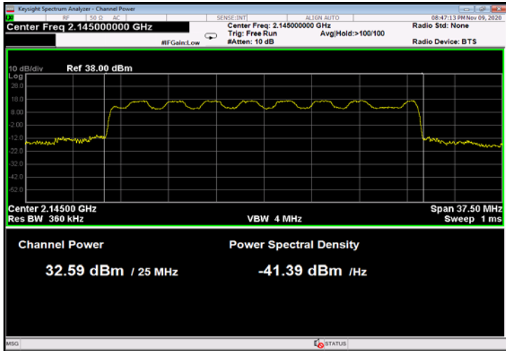
Figure 45: 16QAM 25MHz B.W.; 2145.0MHz, 15kHz
