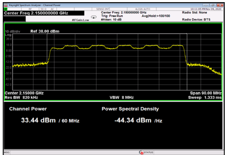
Figure 74: 16QAM 60MHz B.W.; 2150.0MHz, 60kHz
