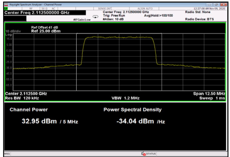
Figure 76: 64QAM 5MHz B.W.; 2112.5MHz, 30kHz
