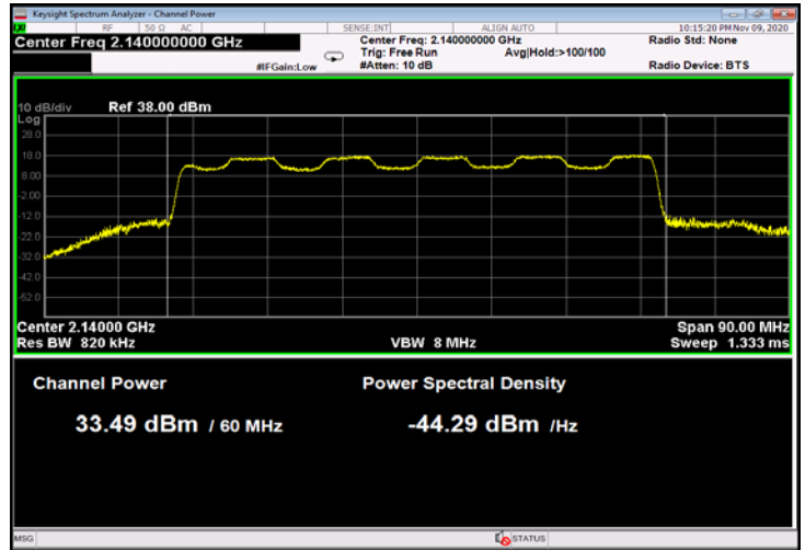
Figure 70: 16QAM 60MHz B.W.; 2140.0MHz, 60kHz
