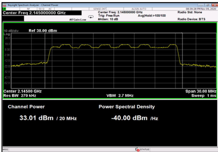
Figure 37: 16QAM 20MHz B.W.; 2145.0MHz, 30kHz
