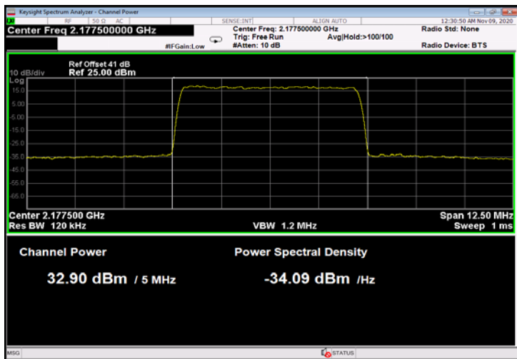
Figure 79: 64QAM 5MHz B.W.; 2177.5MHz, 15kHz
