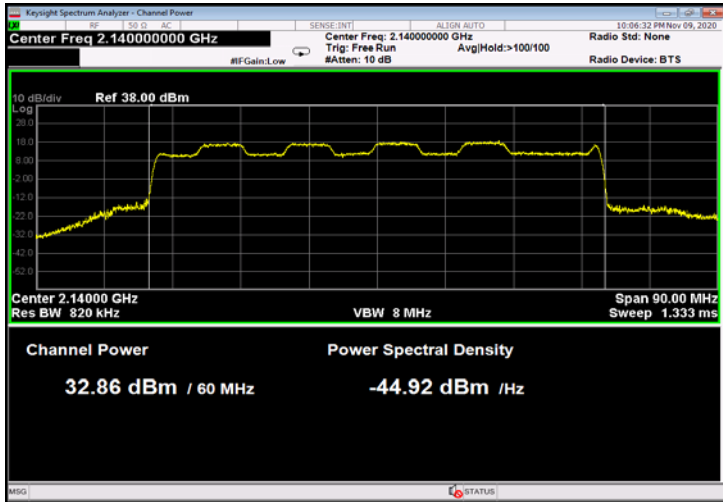
Figure 69: 16QAM 60MHz B.W.; 2140.0MHz, 30kHz
