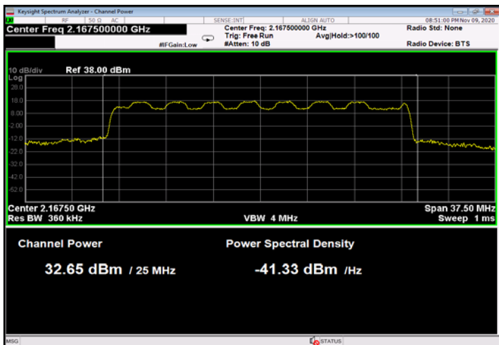
Figure 49: 16QAM 25MHz B.W.; 2167.5MHz, 30kHz
