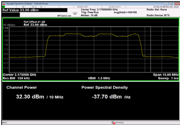
Figure 23: 16QAM 10MHz B.W.; 2175.0MHz, 60kHz
