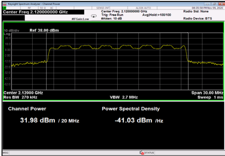
Figure 33: 16QAM 20MHz B.W.; 2120.0MHz, 15kHz
