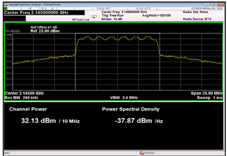
Figure 18: 16QAM 10MHz B.W.; 2145.0MHz, 15kHz
