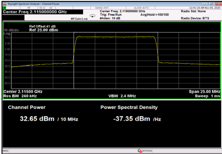
Figure 81: 64QAM 10MHz B.W.;2115.0MHz, 15kHz
