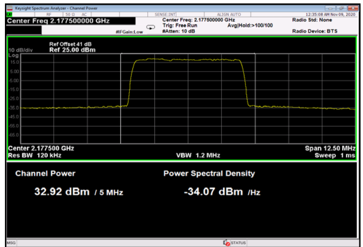
Figure 80: 64QAM 5MHz C.S.; 2177.5MHz, 30kHz
