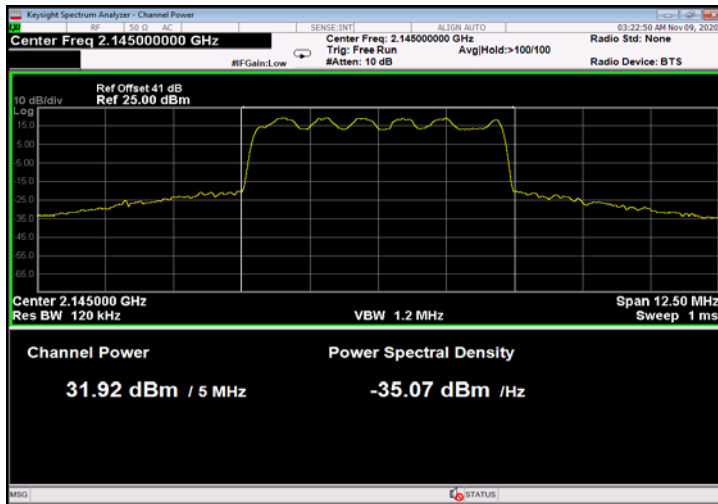
Figure 11: 16QAM 5MHz B.W.; 2145.0MHz, 15kHz
