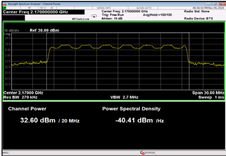
Figure 39: 16QAM 20MHz B.W.; 2170.0MHz, 15kHz
