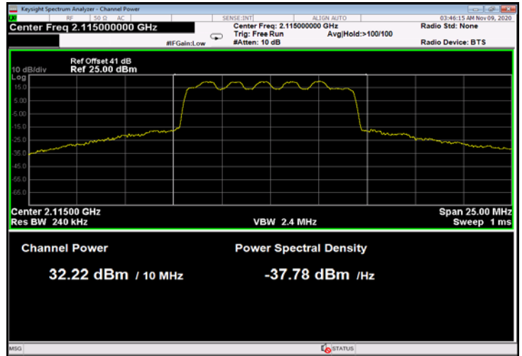
Figure 16: 16QAM 10MHz B.W.; 2115.0MHz, 30kHz
