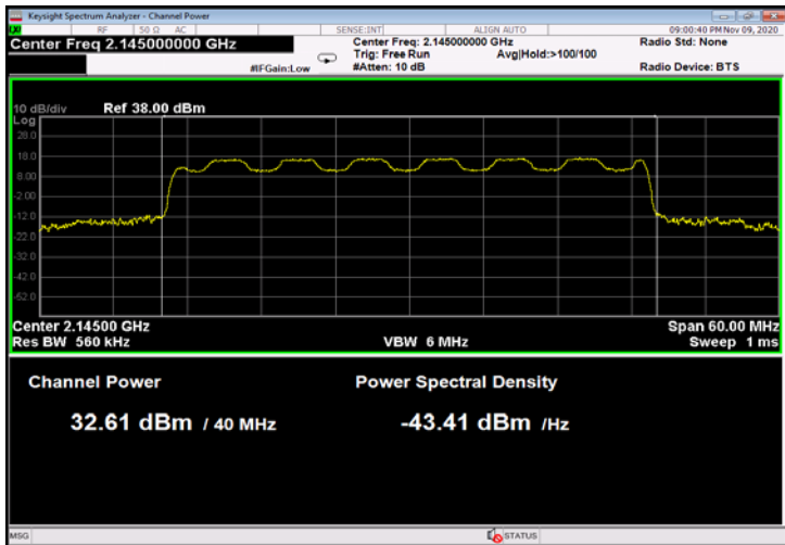
Figure 55: 16QAM 40MHz B.W.; 2145.0MHz, 30kHz
