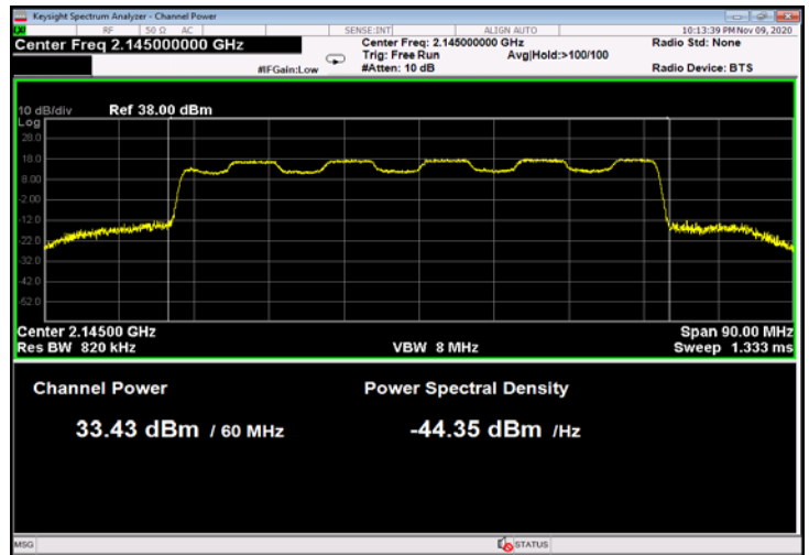
Figure 72: 16QAM 60MHz B.W.; 2145.0MHz, 60kHz
