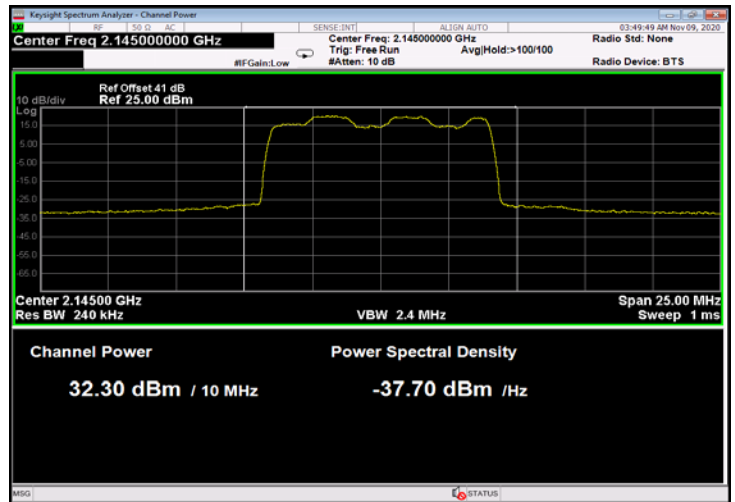
Figure 20: 16QAM 10MHz B.W.; 2145.0MHz, 60kHz
