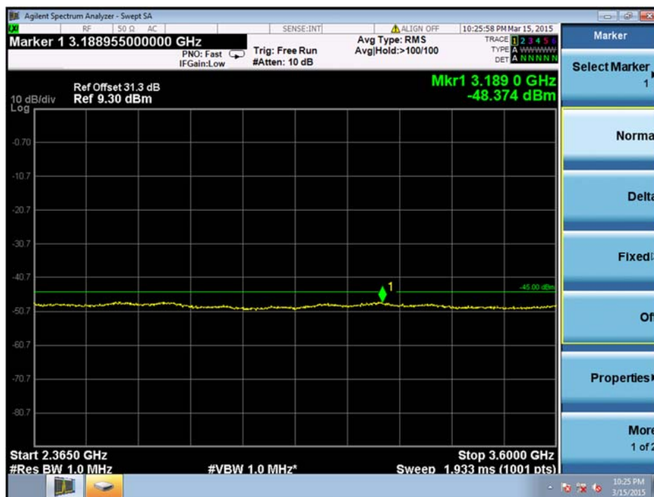
Figure 73.—2365 MHz-3600MHz – W-CDMA
