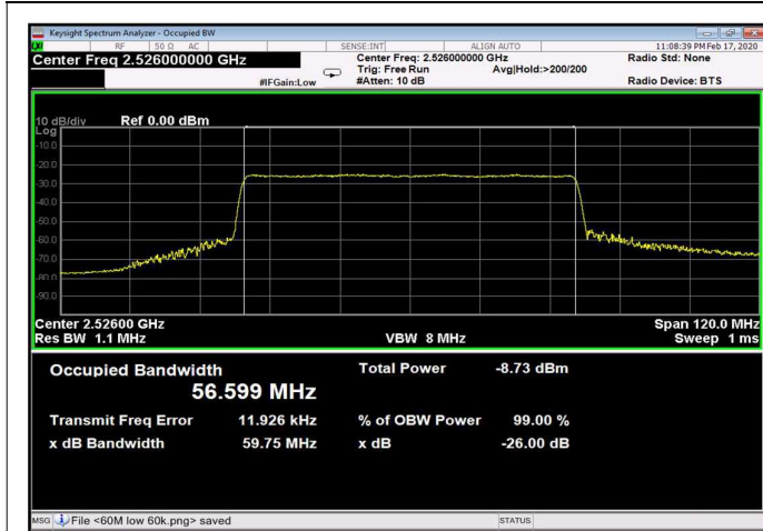
Figure 434: 256QAM 60MHz B.W.; 2526.0MHz, 30kHz Output
