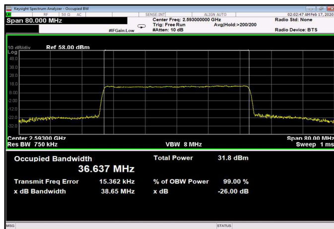
Figure 430: 256QAM 40MHz B.W.; 2593.0MHz, 60kHz Output
