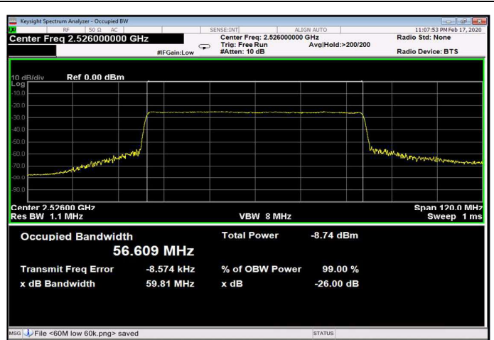
Figure 435: 256QAM 60MHz B.W.; 2526.0MHz, 60kHz Output
