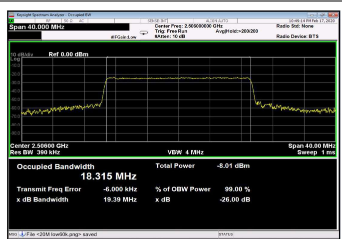
Figure 417: 256QAM 20MHz B.W.; 2506.0MHz, 30kHz Output
