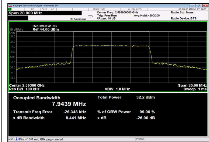
Figure 402: 256QAM 10MHz B.W.; 2593.0MHz, 30kHz Output
