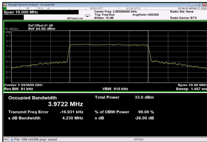
Figure 394: 256QAM 5MHz B.W.; 2593.0MHz, 15kHz Output
