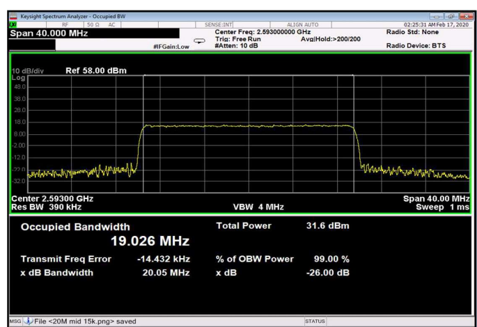
Figure 419: 256QAM 20MHz B.W.; 2593.0MHz, 15kHz Output
