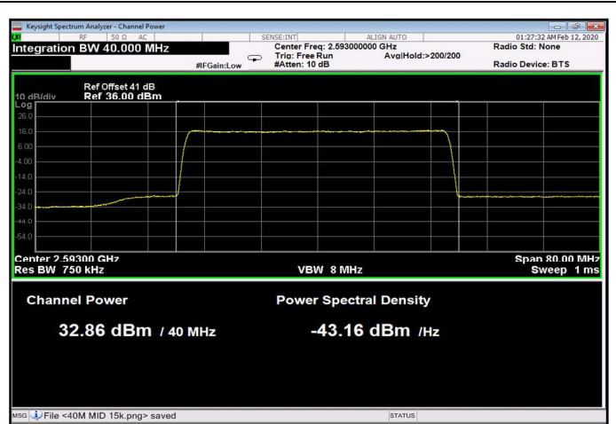
Figure 93: 64QAM 40MHz B.W.; 2593.0MHz, 30kHz
