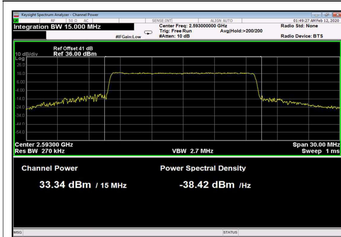
Figure 74: 64QAM 15MHz B.W.; 2593.0MHz, 15kHz
