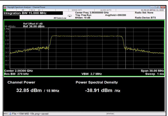
Figure 75: 64QAM 15MHz B.W.; 2593.0MHz, 30kHz
