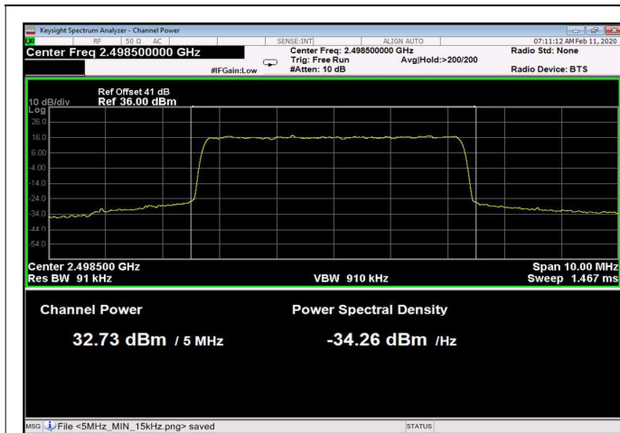
Figure 104: 256QAM 5MHz B.W.; 2498.5MHz, 15kHz
