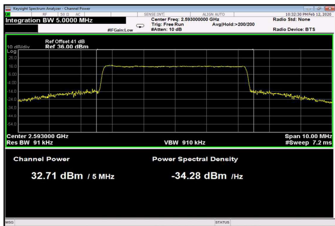
Figure 106: 256QAM 5MHz B.W.; 2593.0MHz, 30kHz
