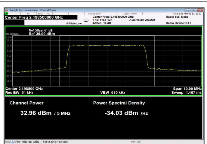
Figure 105: 256QAM 5MHz B.W.; 2498.5MHz, 30kHz
