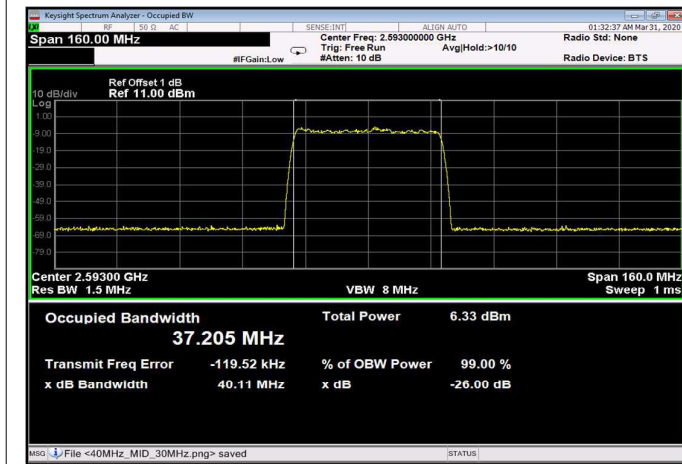
Figure 238: 64QAM 40MHz B.W.; 2593.0MHz, 60kHz Input
