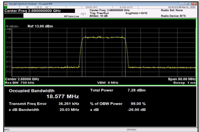
Figure 279: 256QAM 20MHz B.W.; 2680.0MHz, 30kHz Input
