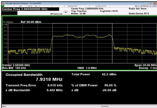
Figure 310: 16QAM 10MHz B.W.; 2685.0MHz, 60kHz Output
