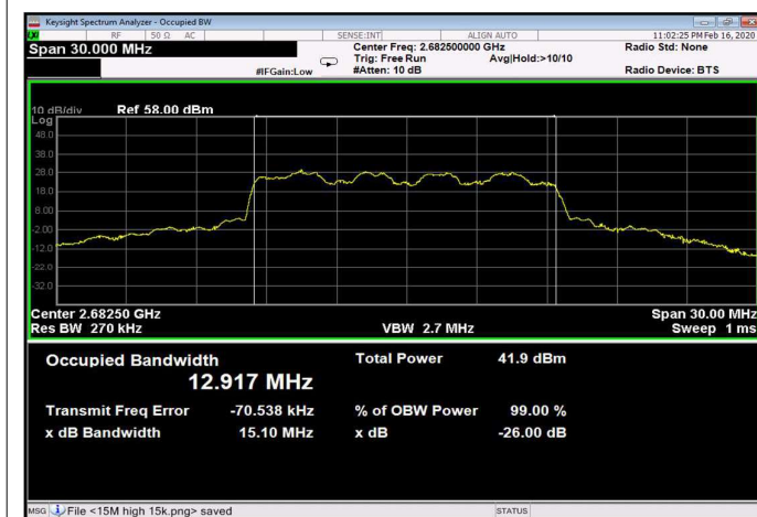
Figure 318: 16QAM 15MHz B.W.; 2682.5MHz, 30kHz Output
