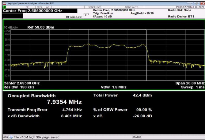
Figure 308: 16QAM 10MHz B.W.; 2685.0MHz, 15kHz Output
