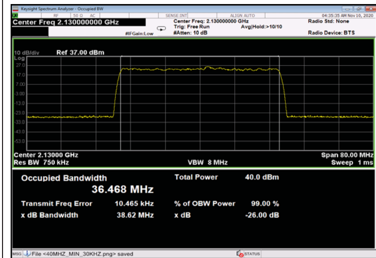
Figure 383: 64QAM 40MHz B.W.; 2130.0MHz, 60kHz - Input
