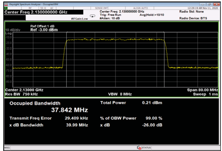
Figure 448: 256QAM 40MHz B.W.; 2130.0MHz, 30kHz - Input
