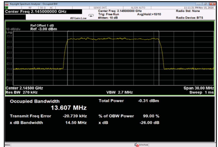
Figure 424: 256QAM 15MHz B.W.; 2145.0MHz, 30kHz - Input
