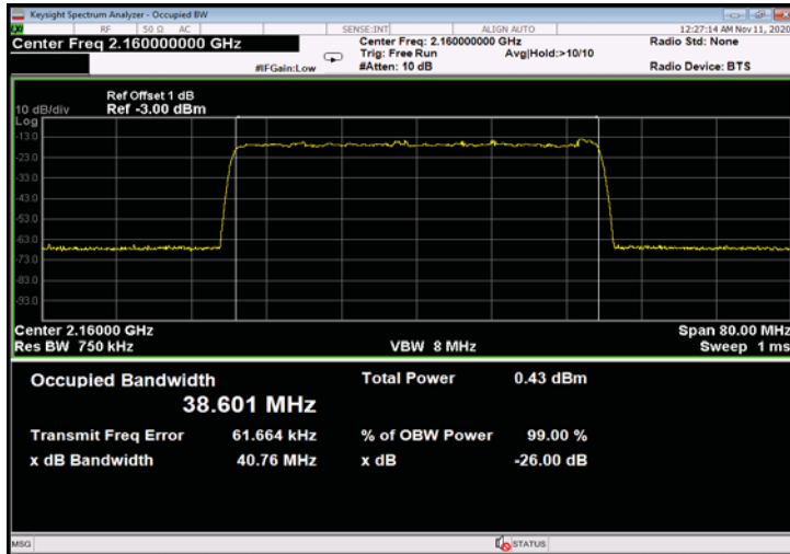
Figure 453: 256QAM 40MHz B.W.; 2160.0MHz, 15kHz - Input
