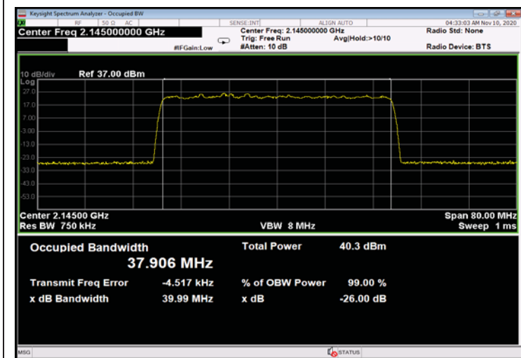
Figure 385: 64QAM 40MHz B.W.; 2145.0MHz, 30kHz - Input
