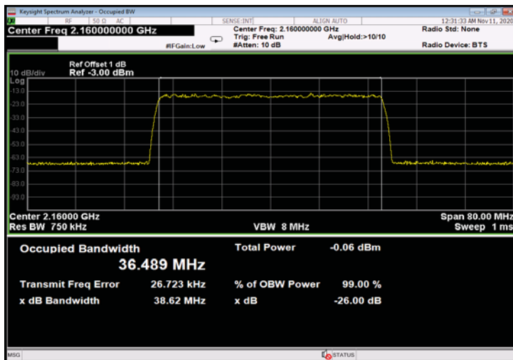
Figure 455: 256QAM 40MHz B.W.; 2160.0MHz, 60kHz - Input
