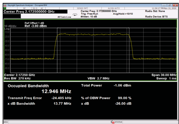
Figure 428: 256QAM 15MHz B.W.; 2172.5MHz, 60kHz - Input
