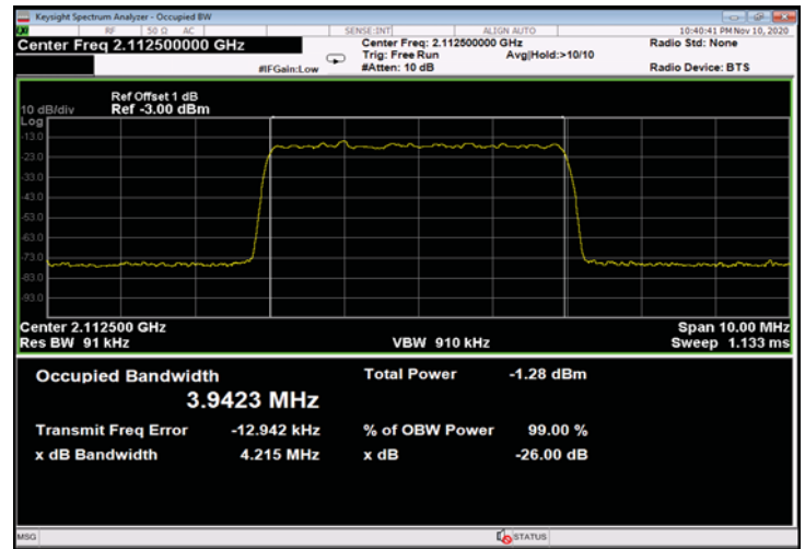
Figure 406: 256QAM 5MHz B.W.; 2112.5MHz, 30kHz - Input
