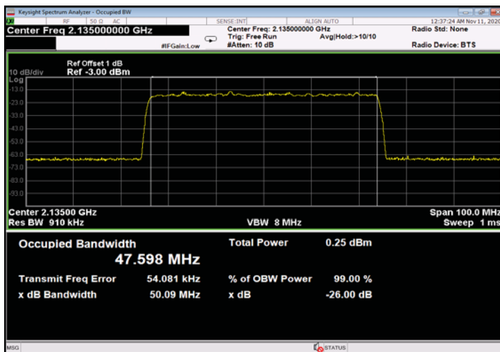
Figure 457: 256QAM 50MHz B.W.; 2135.0MHz, 30kHz - Input
