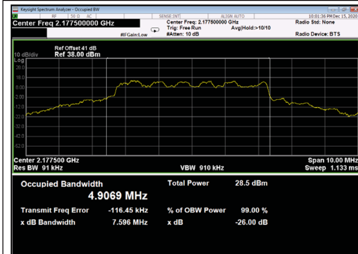
Figure 541: 16QAM 5MHz B.W.; 2177.5MHz, 15kHz - Output
