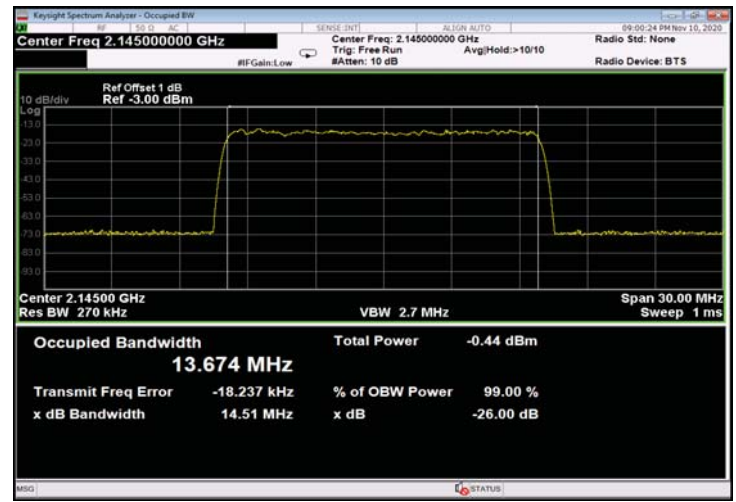
Figure 490: QPSK 15MHz B.W.; 2145.0MHz, 30kHz - Input
