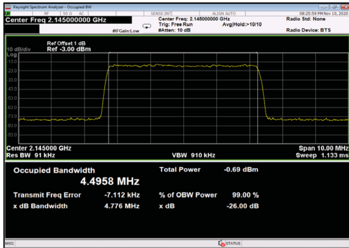
Figure 473: QPSK 5MHz B.W.; 2145.0MHz, 15kHz - Input
