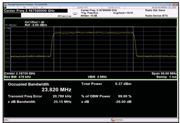
Figure 510: QPSK 25MHz B.W.; 2167.5MHz, 15kHz - Input
