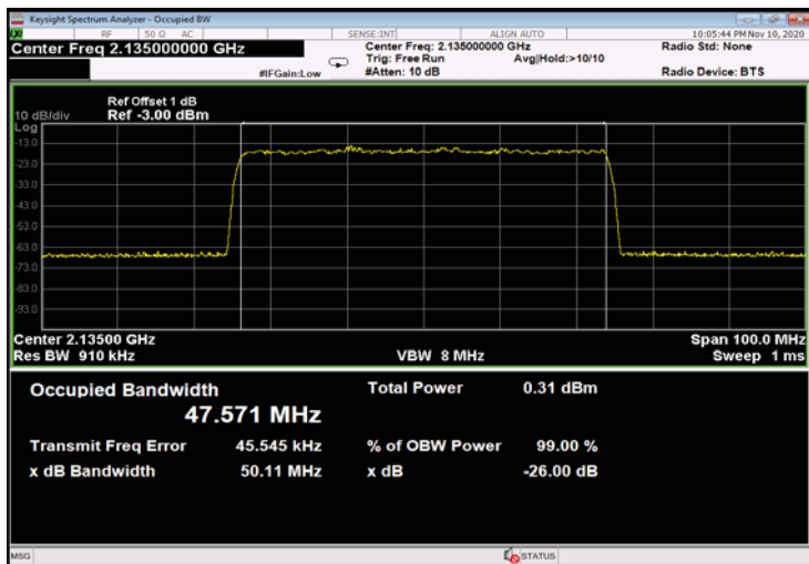
Figure 523: QPSK 50MHz B.W.; 2135.0MHz, 30kHz - Input
