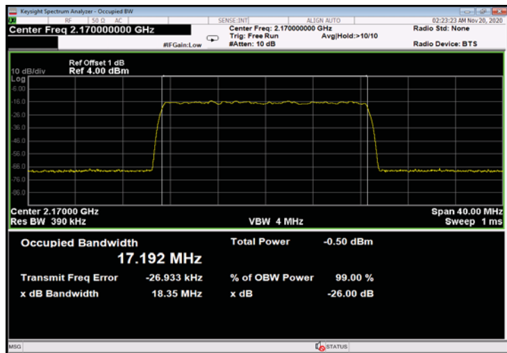
Figure 503: QPSK 20MHz B.W.; 2170.0MHz, 60kHz - Input
