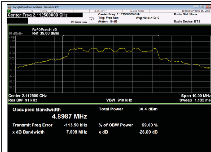
Figure 537: 16QAM 5MHz B.W.; 2112.5MHz, 15kHz - Output
