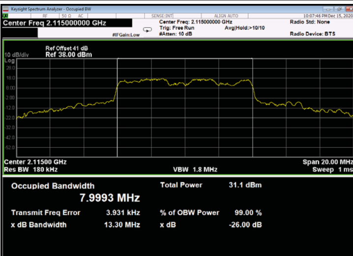
Figure 545: 16QAM 10MHz B.W.; 2115.0MHz, 60kHz - Output
