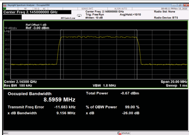
Figure 481: QPSK 10MHz B.W.; 2145.0MHz, 30kHz - Input
