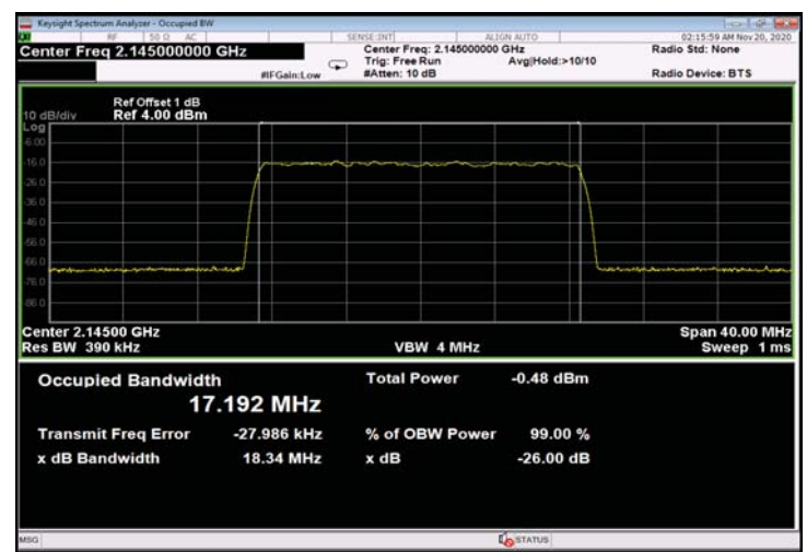
Figure 500: QPSK 20MHz B.W.; 2145.0MHz, 60kHz - Input
