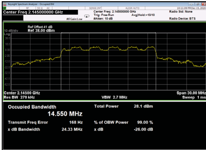
Figure 555: 16QAM 15MHz B.W.; 2145.0MHz, 15kHz - Output
