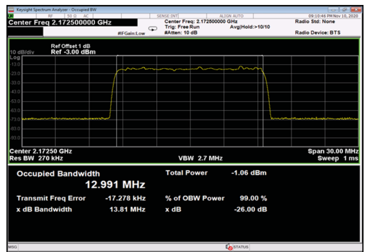
Figure 494: QPSK 15MHz B.W.; 2172.5MHz, 60kHz - Input
