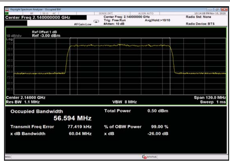
Figure 532: QPSK 60MHz B.W.; 2140.0MHz, 60kHz - Input
