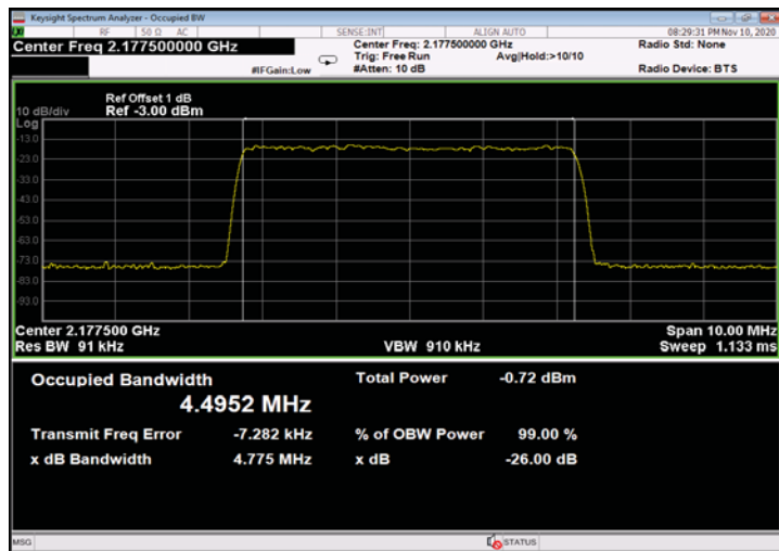
Figure 475: QPSK 5MHz B.W.; 2177.5MHz, 15kHz - Input
