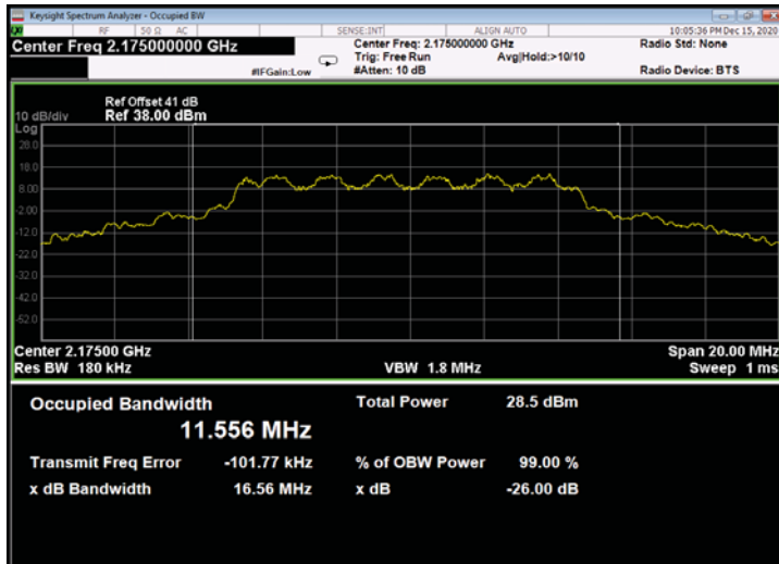
Figure 549: 16QAM 10MHz B.W.; 2175.0MHz, 15kHz - Output
