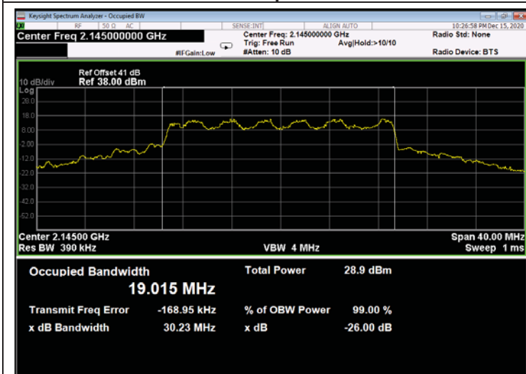
Figure 565: 16QAM 20MHz B.W.; 2145.0MHz, 30kHz - Output
