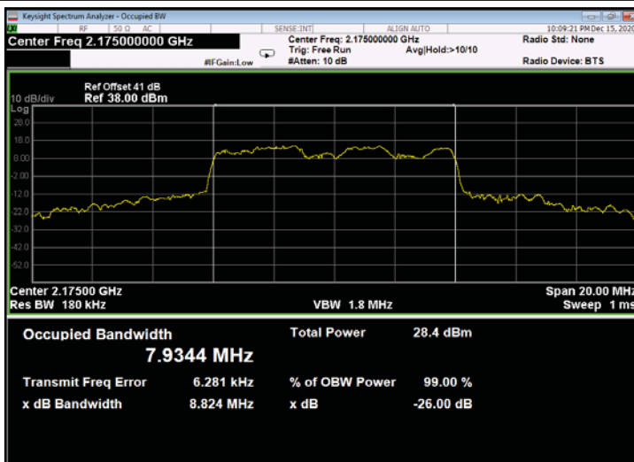
Figure 551: 16QAM 10MHz B.W.; 2175.0MHz, 60kHz - Output
