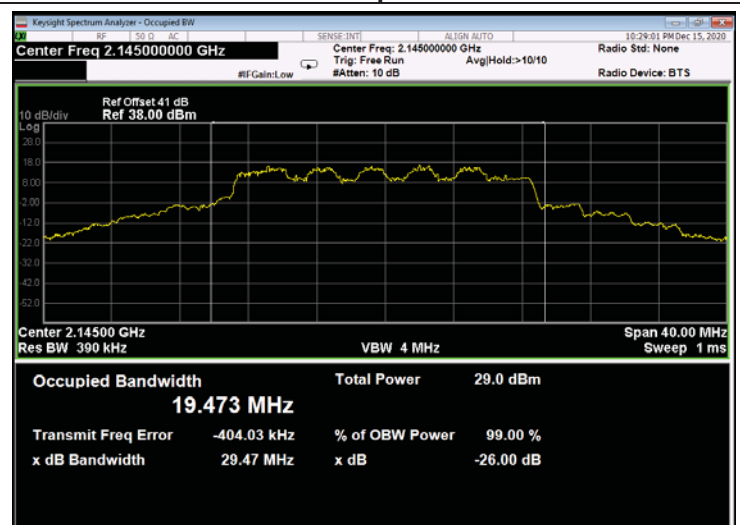
Figure 566: 16QAM 20MHz B.W.; 2145.0MHz, 60kHz - Output
