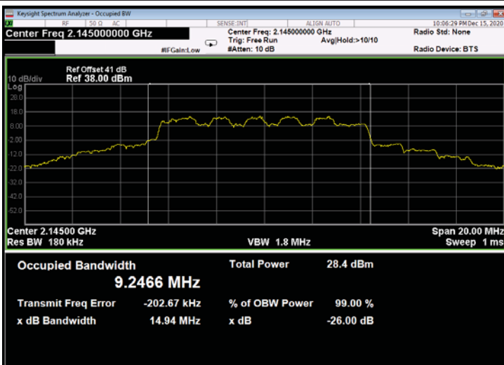
Figure 547: 16QAM 10MHz B.W.; 2145.0MHz, 30kHz - Output
