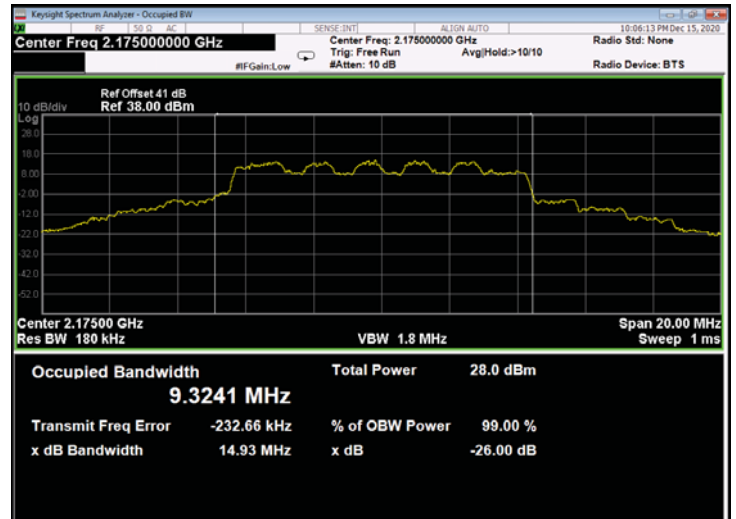
Figure 550: 16QAM 10MHz B.W.; 2175.0MHz, 30kHz - Output
