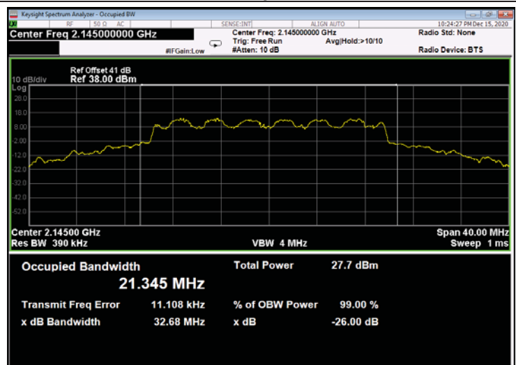
Figure 564: 16QAM 20MHz B.W.; 2145.0MHz, 15kHz - Output
