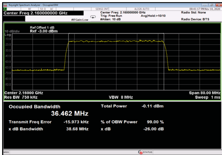
Figure 521: QPSK 40MHz B.W.; 2160.0MHz, 60kHz - Input
