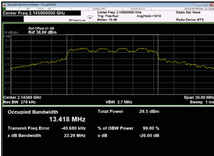
Figure 557: 16QAM 15MHz B.W.; 2145.0MHz, 60kHz - Output
