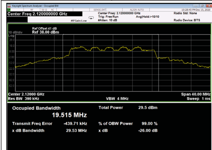
Figure 563: 16QAM 20MHz B.W.; 2120.0MHz, 60kHz - Output
