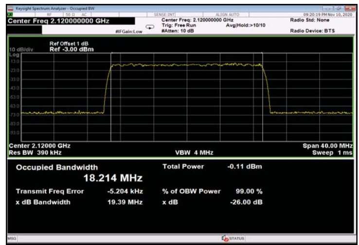
Figure 496: QPSK 20MHz B.W.; 2120.0MHz, 30kHz - Input
