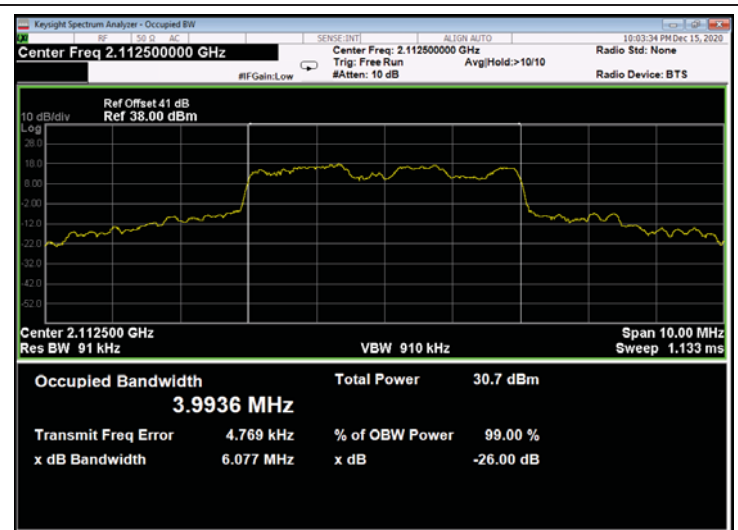
Figure 538: 16QAM 5MHz B.W.; 2112.5MHz, 30kHz - Output
