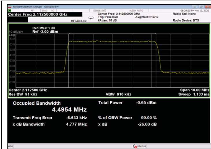
Figure 471: QPSK 5MHz B.W.; 2112.5MHz, 15kHz - Input
