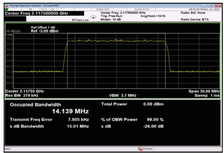
Figure 486: QPSK 15MHz B.W.; 2117.5MHz, 15kHz - Input
