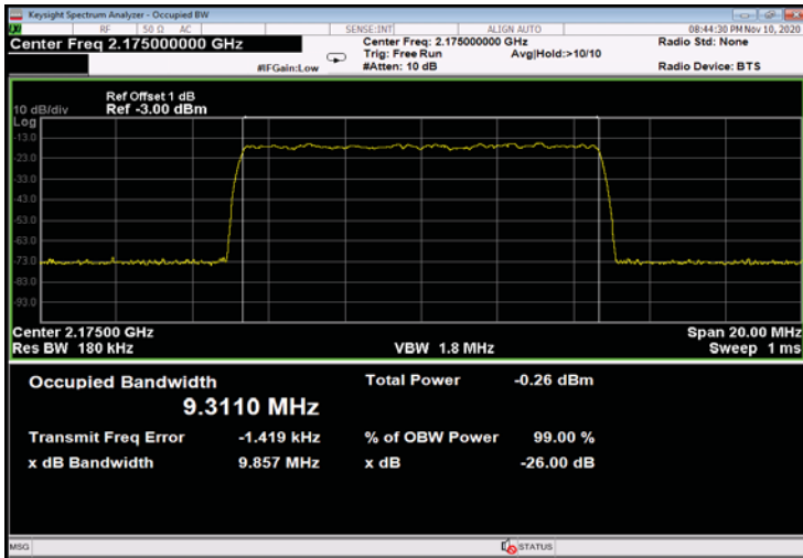
Figure 483: QPSK 10MHz B.W.; 2175.0MHz, 15kHz - Input
