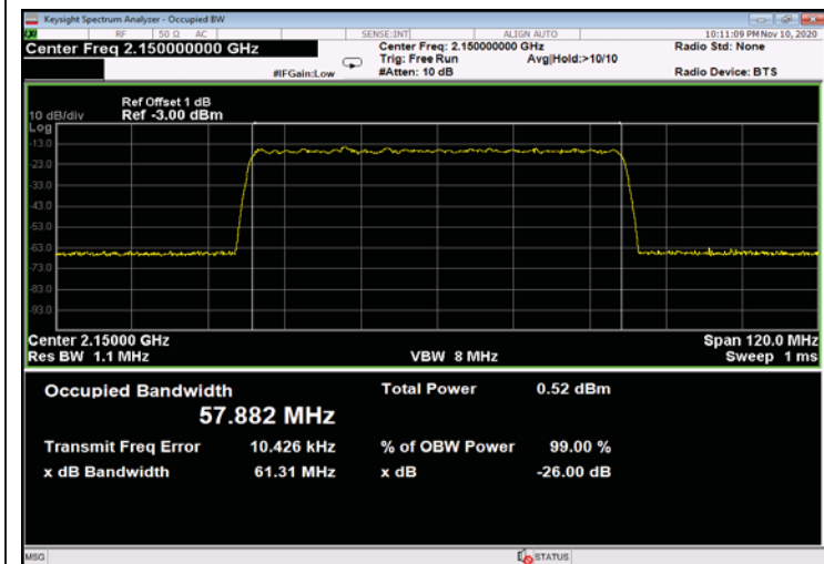
Figure 535: QPSK 60MHz B.W.; 2150.0MHz, 30kHz - Input
