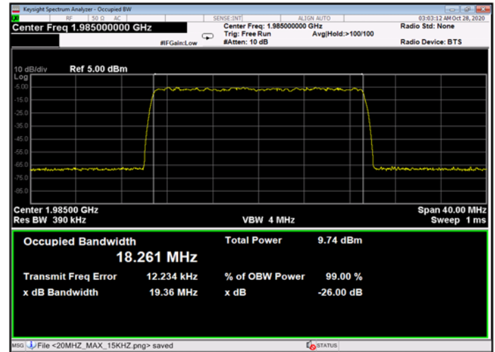
Figure 436: 256QAM 20MHz B.W.; 1985.0MHz, 30kHz - Input
