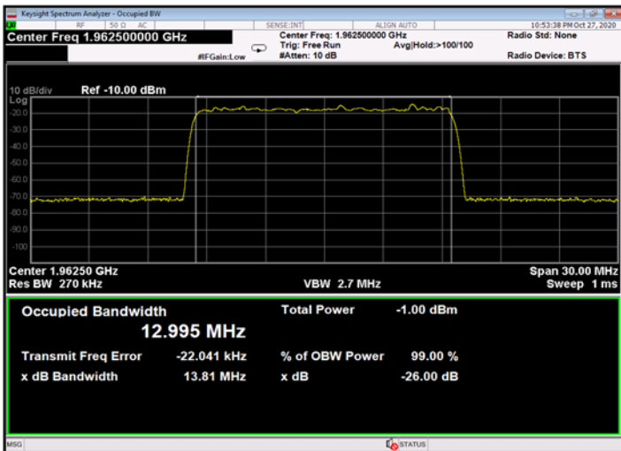
Figure 491: QPSK 15MHz B.W.; 1962.5MHz, 60kHz - Input
