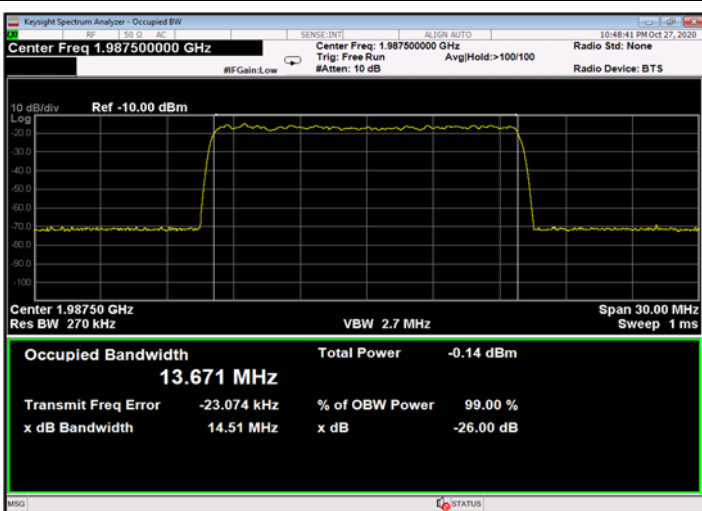
Figure 493: QPSK 15MHz B.W.; 1987.5MHz, 30kHz - Input
