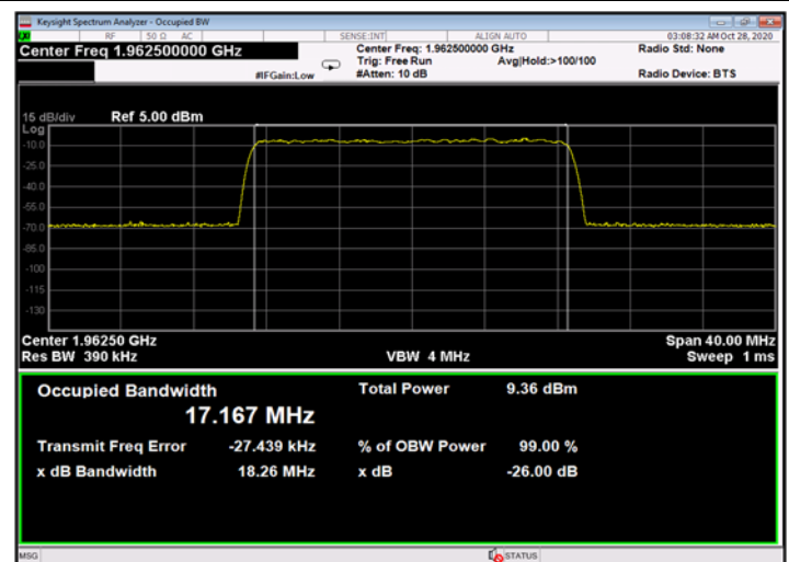
Figure 434: 256QAM 20MHz B.W.; 1962.5MHz, 60kHz - Input
