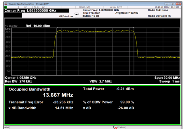
Figure 490: QPSK 15MHz B.W.; 1962.5MHz, 30kHz - Input
