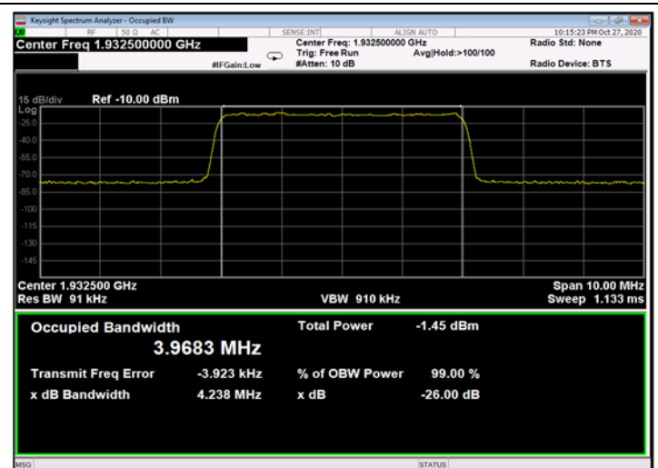
Figure 472: QPSK 5MHz B.W.; 1932.5MHz, 30kHz - Input
