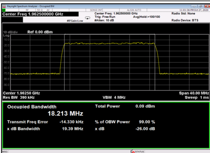
Figure 499: QPSK 20MHz B.W.; 1962.5MHz, 30kHz - Input
