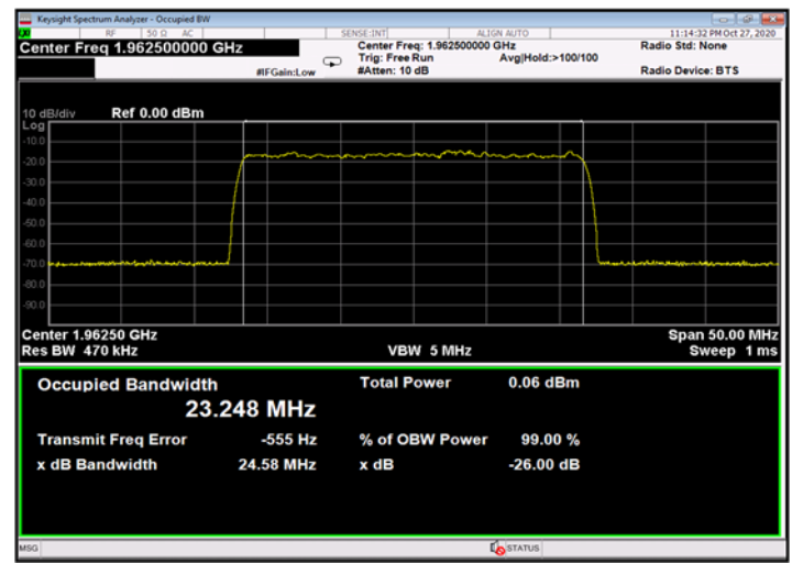
Figure 508: QPSK 25MHz B.W.; 1962.5MHz, 30kHz - Input
