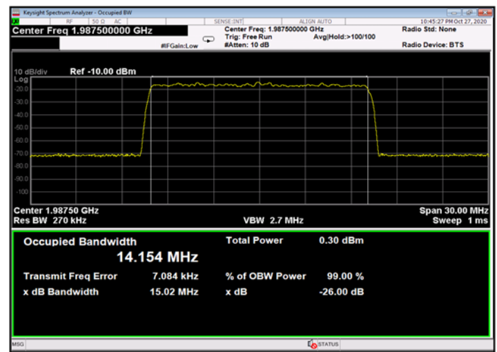
Figure 492: QPSK 15MHz B.W.; 1987.5MHz, 15kHz - Input
