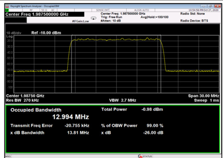
Figure 494: QPSK 15MHz B.W.; 1987.5MHz, 60kHz - Input
