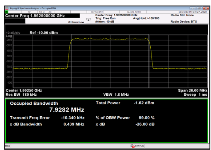
Figure 482: QPSK 10MHz B.W.; 1962.5MHz, 60kHz - Input
