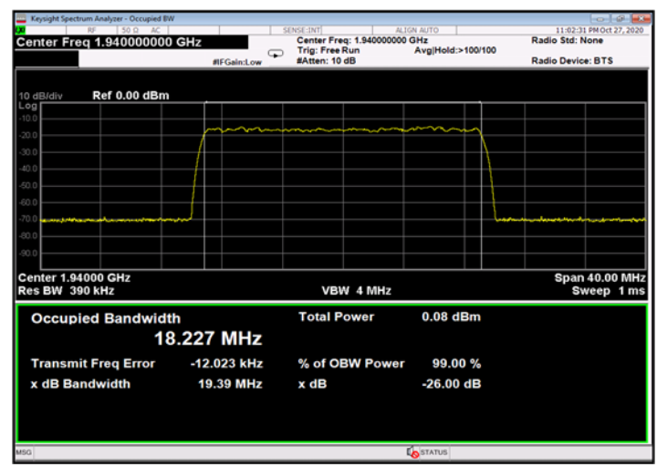
Figure 496: QPSK 20MHz B.W.; 1940.0MHz, 30kHz - Input
