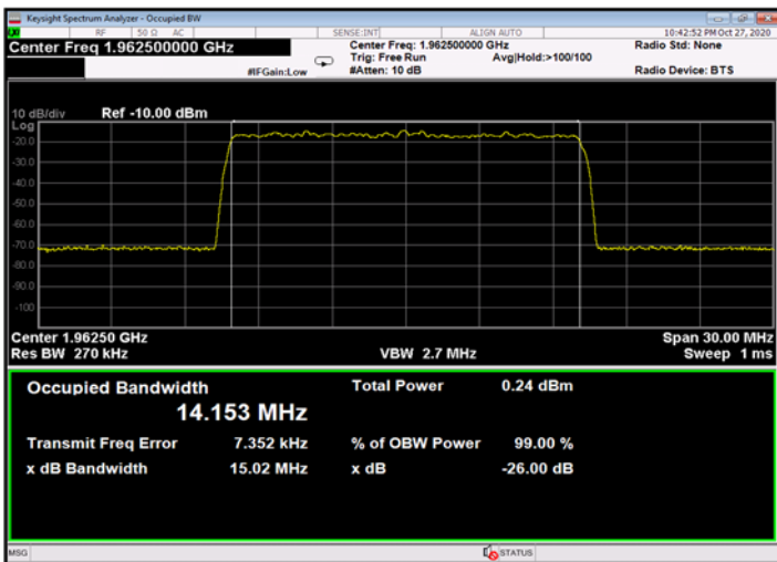
Figure 489: QPSK 15MHz B.W.; 1962.5MHz, 15kHz - Input
