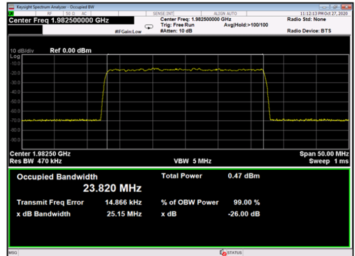
Figure 510: QPSK 25MHz B.W.; 1982.5MHz, 15kHz - Input
