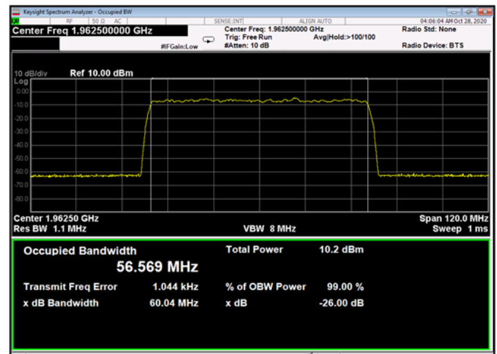
Figure 468: 256QAM 60MHz B.W.; 1962.5MHz, 60kHz - Input
