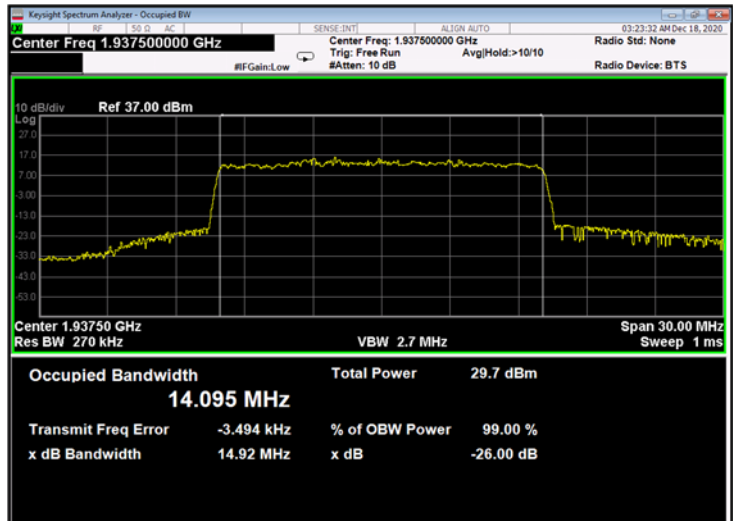
Figure 618: 64QAM 15MHz B.W.; 1937.5MHz, 15kHz - Output
