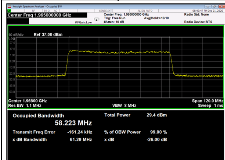
Figure 667: 64QAM 60MHz B.W.; 1965.0MHz, 30kHz - Output
