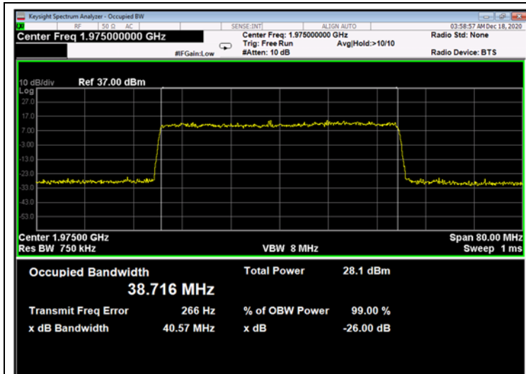
Figure 651: 64QAM 40MHz B.W.; 1975.0MHz, 15kHz - Output
