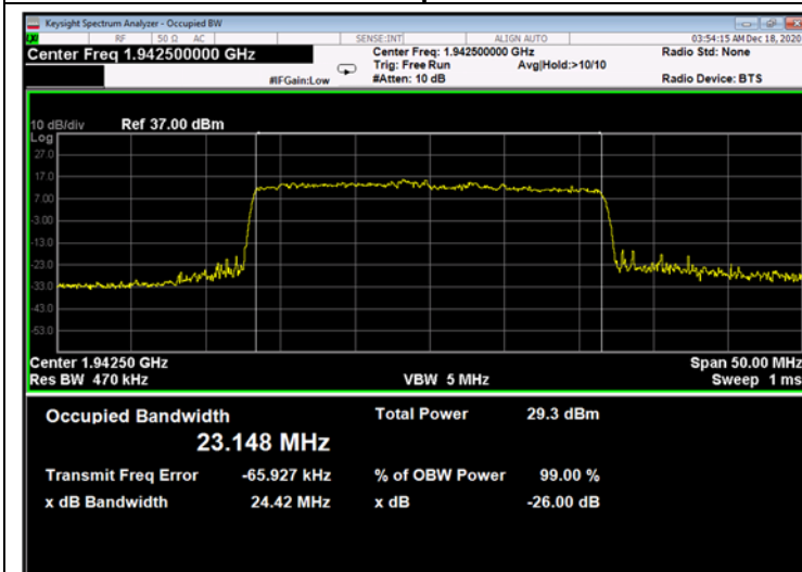
Figure 637: 64QAM 25MHz B.W.; 1942.5MHz, 30kHz - Output
