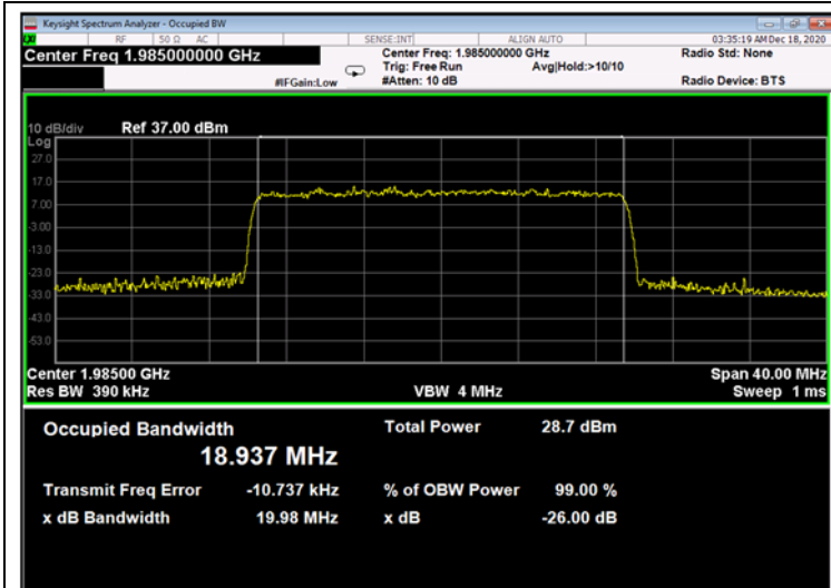
Figure 633: 64QAM 20MHz B.W.; 1985.0MHz, 15kHz - Output
