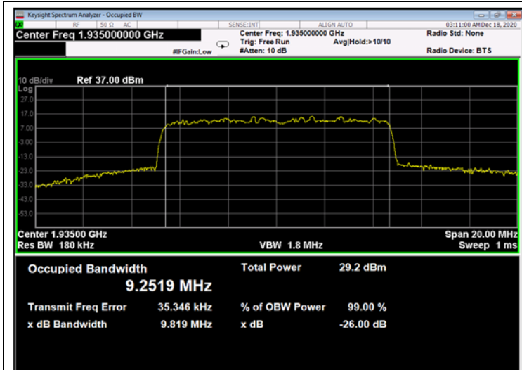
Figure 609: 64QAM 10MHz B.W.; 1935.00MHz, 15kHz - Output
