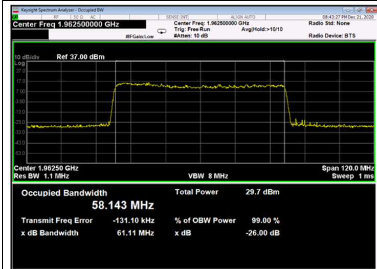
Figure 665: 64QAM 60MHz B.W.; 1962.5MHz, 30kHz - Output
