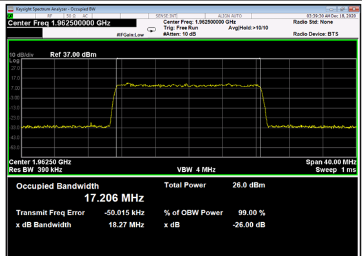
Figure 632: 64QAM 20MHz B.W.; 1962.5MHz, 60kHz - Output
