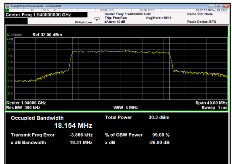
Figure 628: 64QAM 20MHz B.W.; 1940.0MHz, 30kHz - Output
