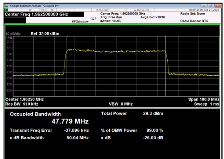
Figure 658: 64QAM 50MHz B.W.; 1962.5MHz, 30kHz - Output
