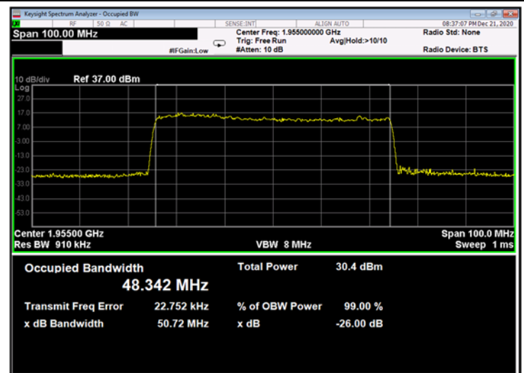
Figure 654: 64QAM 50MHz B.W.; 1955.0MHz, 15kHz - Output
