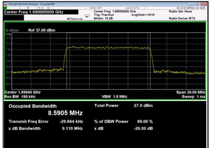
Figure 616: 64QAM 10MHz B.W.; 1990.0MHz, 30kHz - Output
