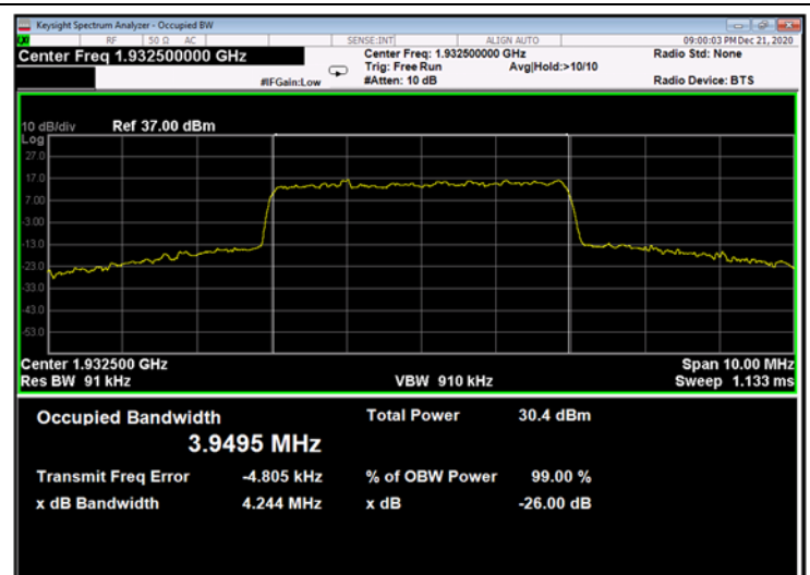
Figure 670: 256QAM 5MHz B.W.; 1932.5MHz, 30kHz - Output
