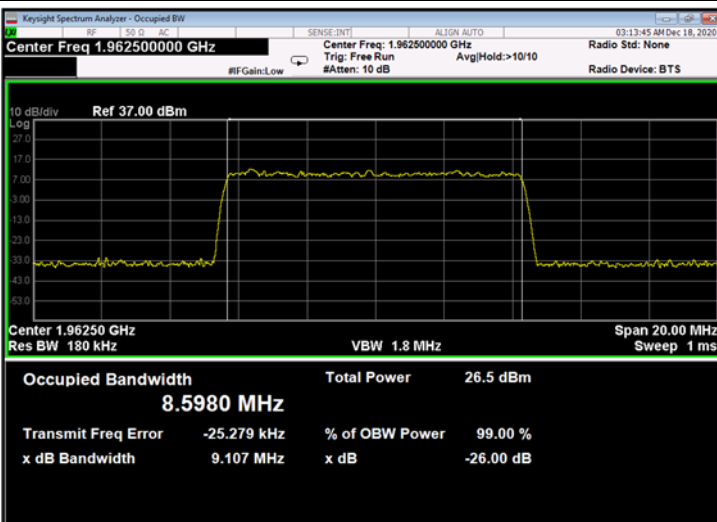
Figure 613: 64QAM 10MHz B.W.; 1962.5MHz, 30kHz - Output
