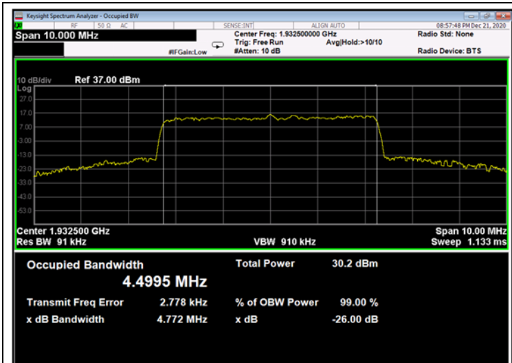
Figure 669: 256QAM 5MHz B.W.; 1932.5MHz, 15kHz - Output
