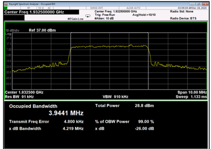
Figure 604: 64QAM 5MHz B.W.; 1932.5MHz, 30kHz - Output
