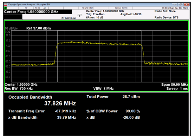
Figure 646: 64QAM 40MHz B.W.; 1950.0MHz, 30kHz - Output
