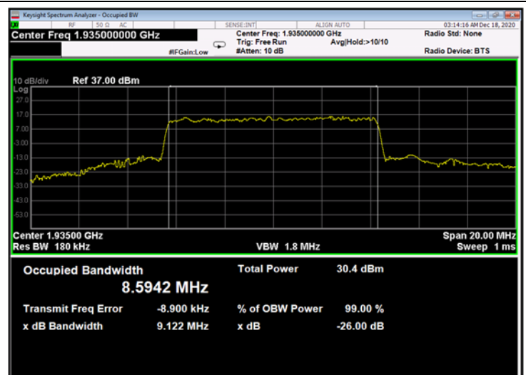
Figure 610: 64QAM 10MHz B.W.; 1935.0MHz, 30kHz - Output
