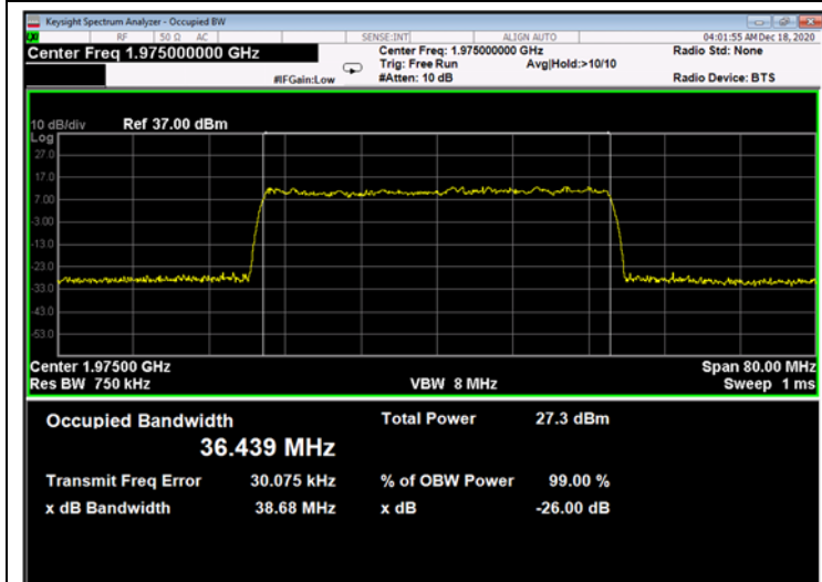
Figure 653: 64QAM 40MHz B.W.; 1975.0MHz, 60kHz - Output
