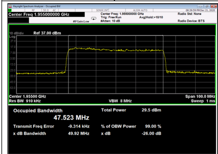
Figure 655: 64QAM 50MHz B.W.; 1955.0MHz, 30kHz - Output
