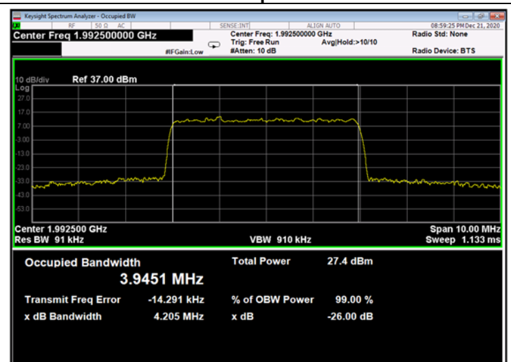
Figure 674: 256QAM 5MHz C.S.; 1992.5MHz, 30kHz - Output
