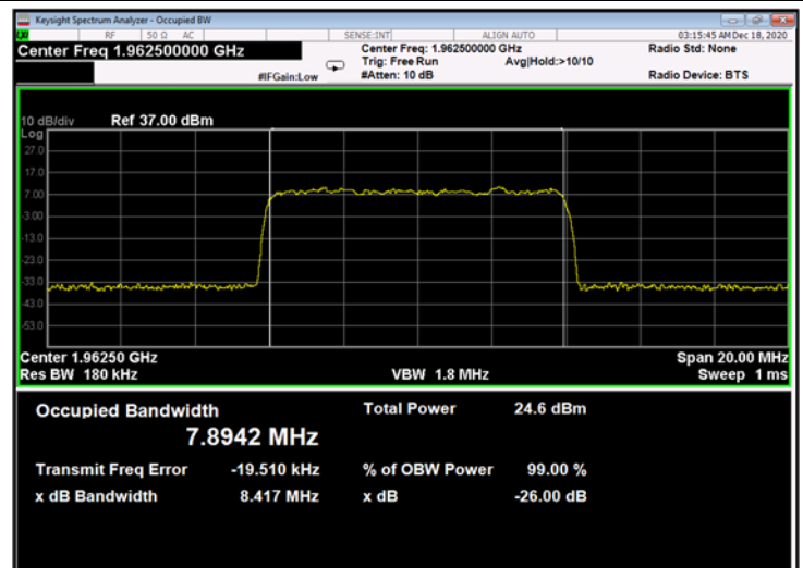
Figure 614: 64QAM 10MHz B.W.; 1962.5MHz, 60kHz - Output
