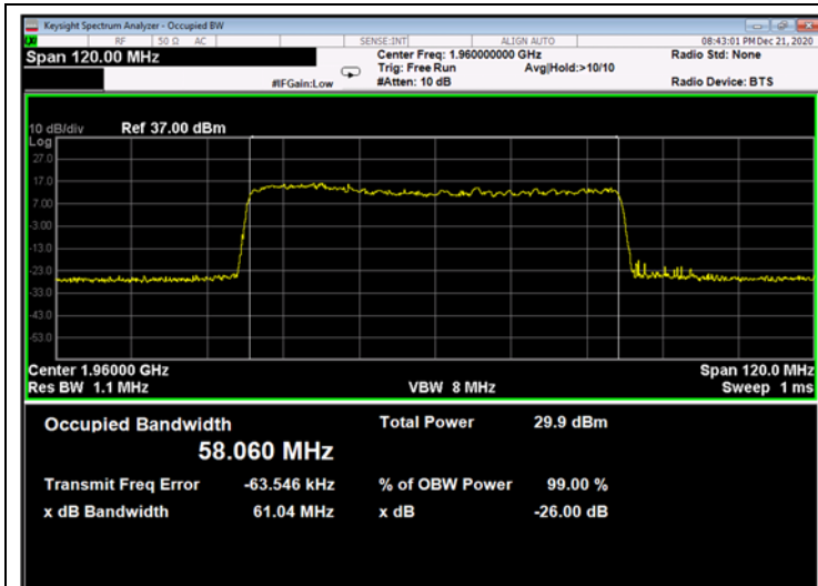
Figure 663: 64QAM 60MHz B.W.; 1960.0MHz, 30kHz - Output
