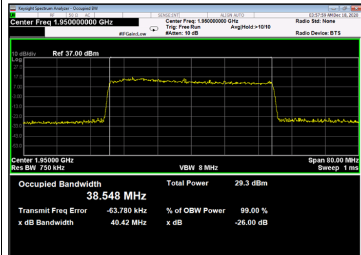
Figure 645: 64QAM 40MHz B.W.; 1950.0MHz, 15kHz – Output
