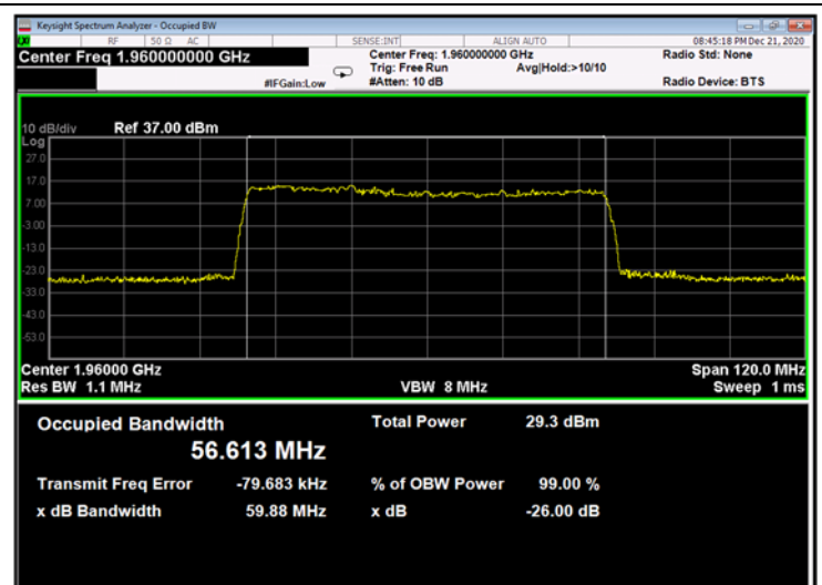
Figure 664: 64QAM 60MHz B.W.; 1960.0MHz, 60kHz - Output
