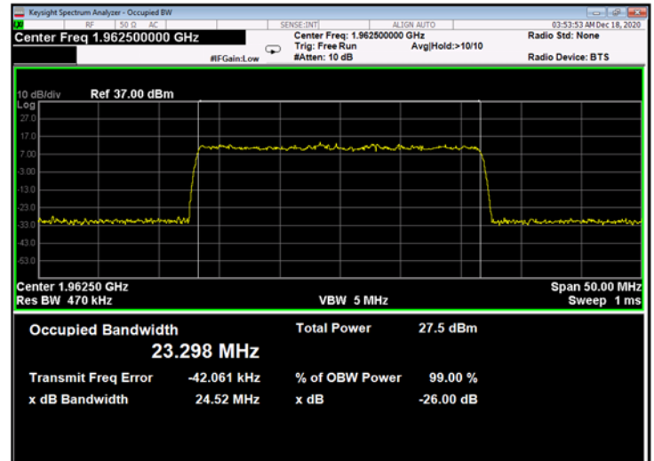
Figure 640: 64QAM 25MHz B.W.; 1962.5MHz, 30kHz - Output
