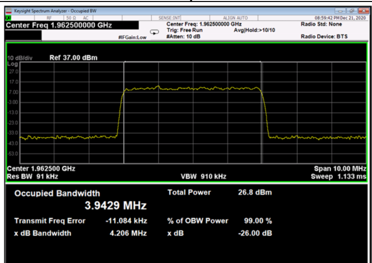
Figure 672: 256QAM 5MHz B.W.; 1962.5MHz, 30kHz - Output
