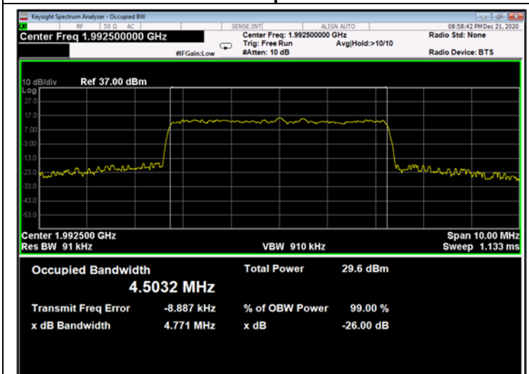
Figure 673: 256QAM 5MHz B.W.; 1992.5MHz, 15kHz - Output
