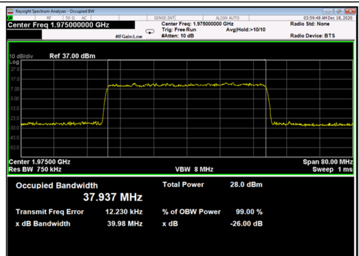
Figure 652: 64QAM 40MHz B.W.; 1975.0MHz, 30kHz - Output
