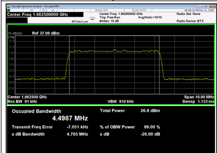
Figure 671: 256QAM 5MHz B.W.; 1962.5MHz, 15kHz - Output
