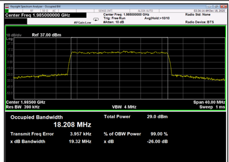
Figure 634: 64QAM 20MHz B.W.; 1985.0MHz, 30kHz - Output
