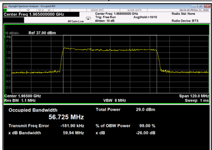
Figure 668: 64QAM 60MHz B.W.; 1965.0MHz, 60kHz - Output
