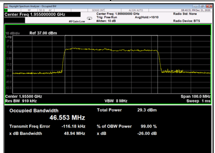
Figure 656: 64QAM 50MHz B.W.; 1955.0MHz, 60kHz - Output
