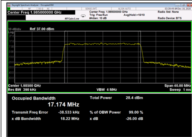
Figure 635: 64QAM 20MHz B.W.; 1985.0MHz, 60kHz - Output
