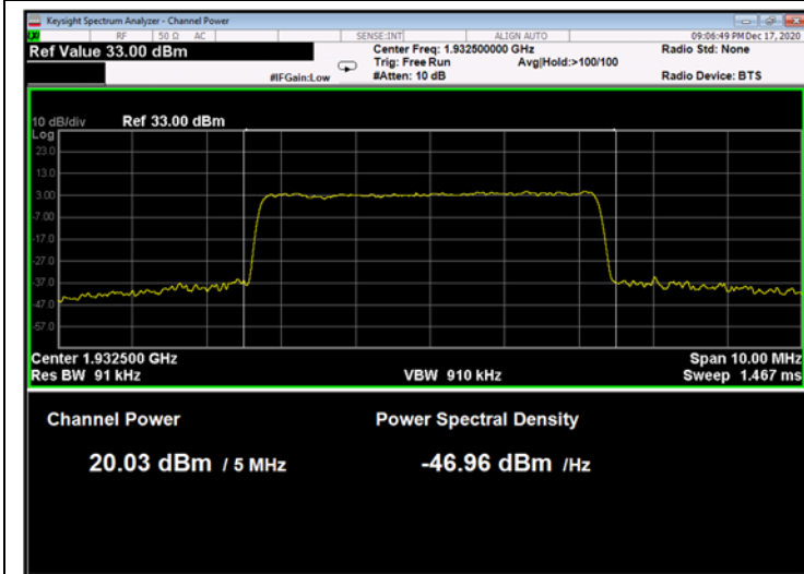
Figure 75: 64QAM 5MHz B.W.; 1932.5MHz, 15kHz
