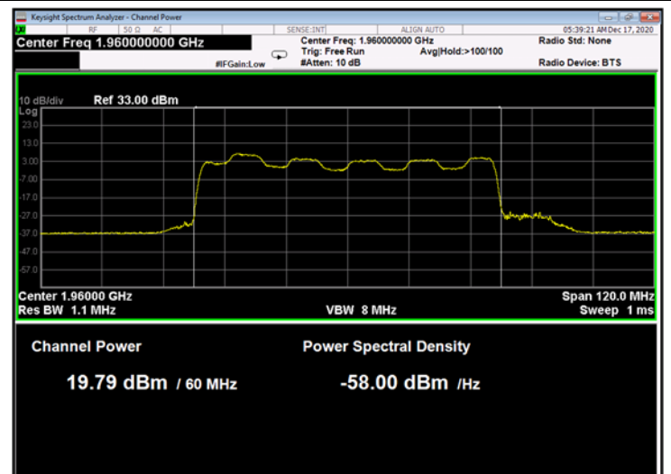
Figure 70: 16QAM 60MHz B.W.; 1960.0MHz, 60kHz
