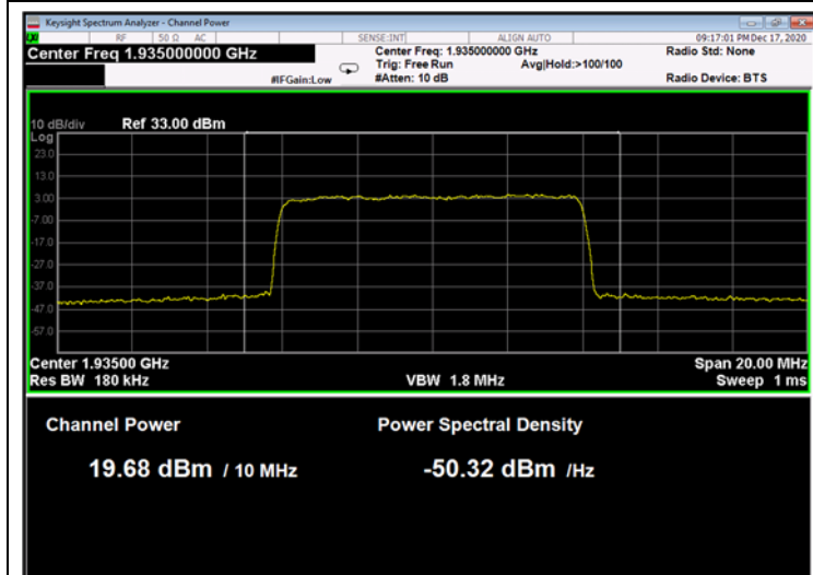
Figure 83: 64QAM 10MHz B.W.; 1935.0MHz, 60kHz
