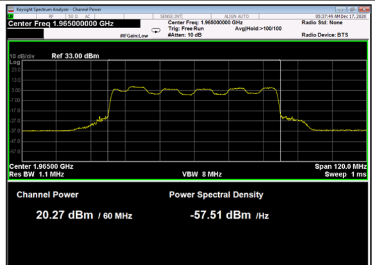
Figure 74: 16QAM 60MHz B.W.; 1965.0MHz, 60kHz
