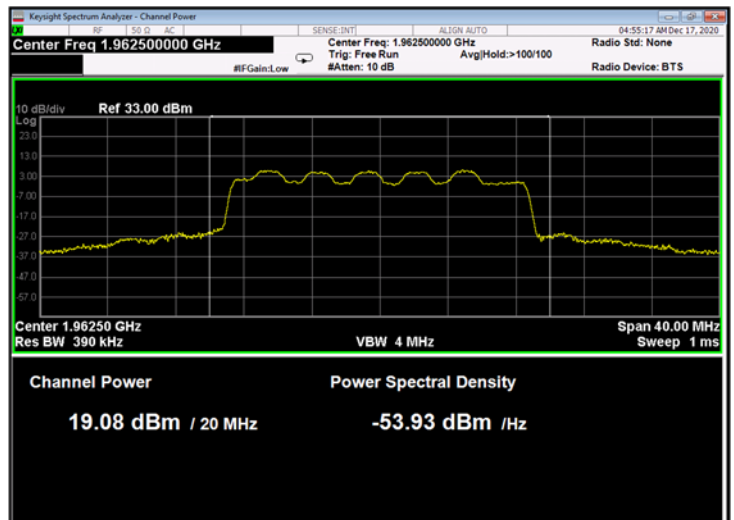
Figure 38: 16QAM 20MHz B.W.; 1962.5MHz, 60kHz
