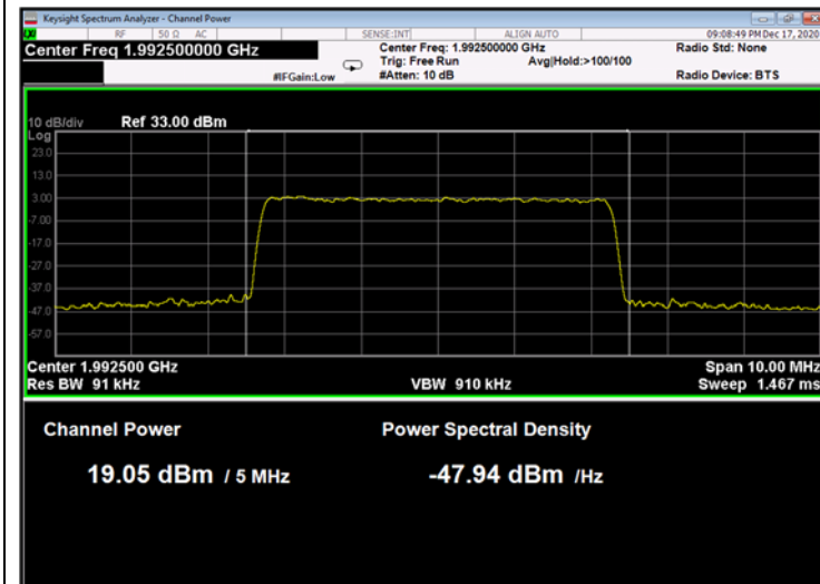
Figure 79: 64QAM 5MHz B.W.; 1992.5MHz, 15kHz
