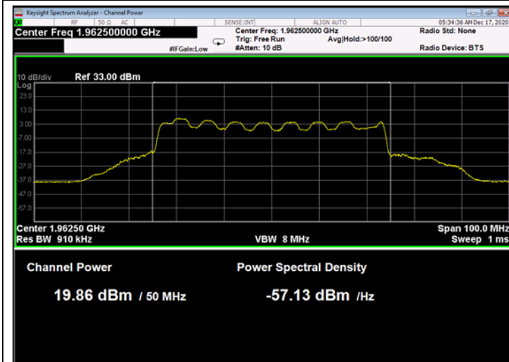
Figure 65: 16QAM 50MHz B.W.; 1962.5MHz, 60kHz
