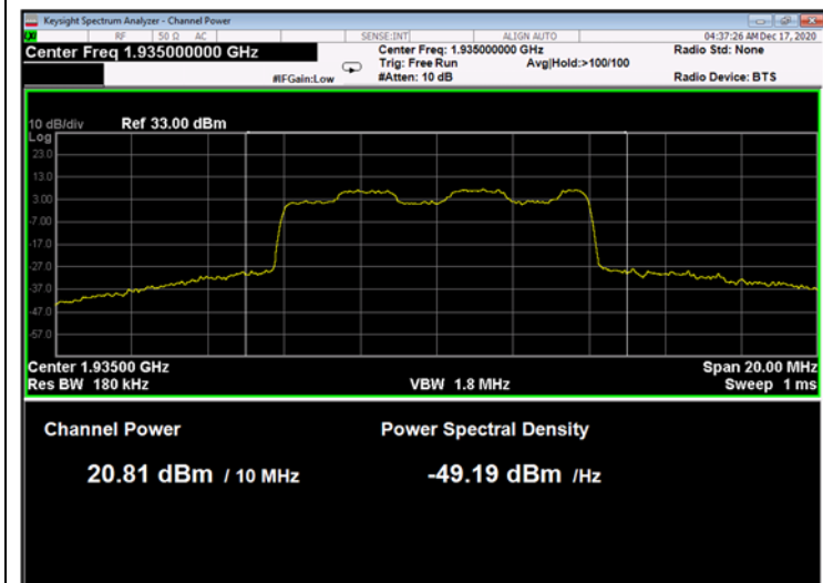
Figure 17: 16QAM 10MHz B.W.; 1935.0MHz, 60kHz
