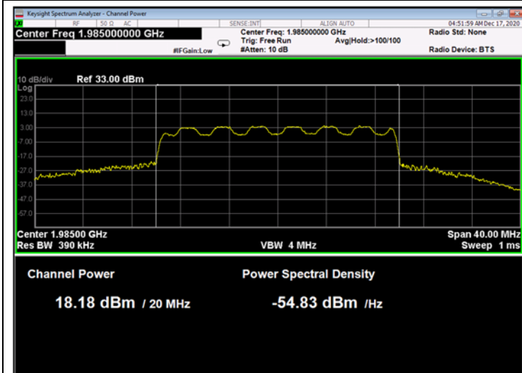
Figure 39: 16QAM 20MHz B.W.; 1985.0MHz, 15kHz
