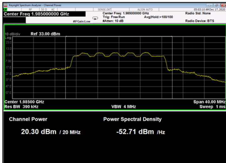
Figure 41: 16QAM 20MHz B.W.; 1985.0MHz, 60kHz
