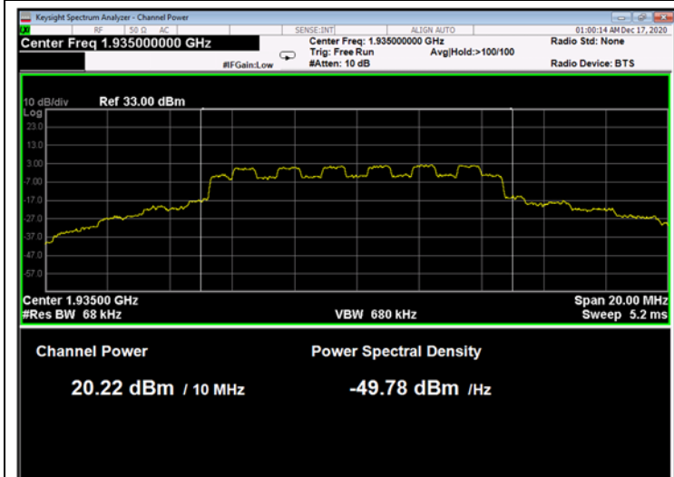
Figure 15: 16QAM 10MHz B.W.; 1935.00MHz, 15kHz
