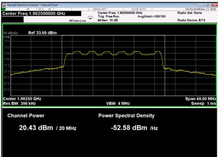
Figure 37: 16QAM 20MHz B.W.; 1962.5MHz, 30kHz
