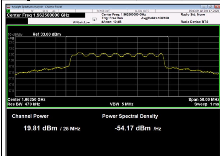
Figure 47: 16QAM 25MHz B.W.; 1962.5MHz, 60kHz
