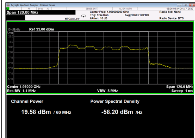
Figure 69: 16QAM 60MHz B.W.; 1960.0MHz, 30kHz
