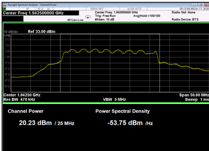
Figure 43: 16QAM 25MHz B.W.; 1942.5MHz, 30kHz
