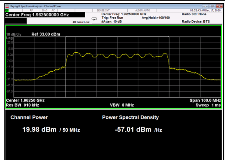
Figure 64: 16QAM 50MHz B.W.; 1962.5MHz, 30kHz
