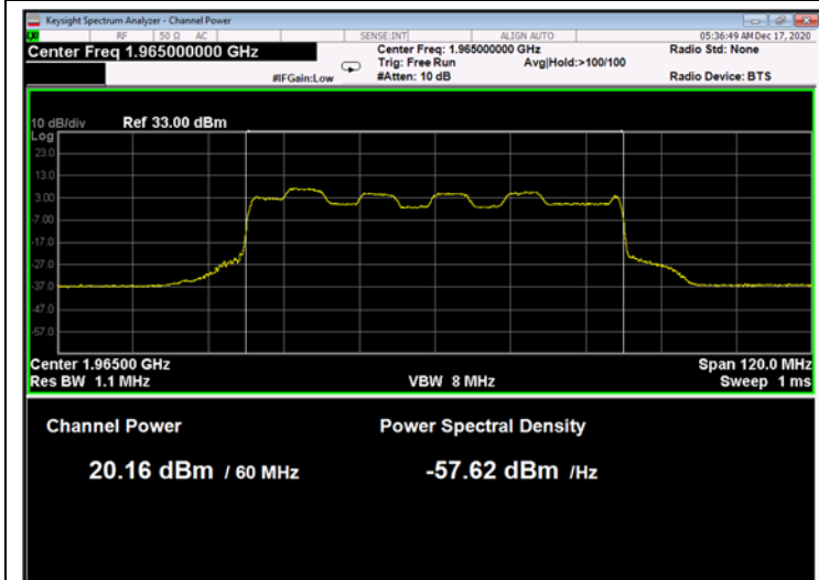
Figure 73: 16QAM 60MHz B.W.; 1965.0MHz, 30kHz
