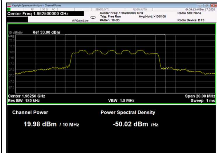
Figure 19: 16QAM 10MHz B.W.; 1962.5MHz, 30kHz
