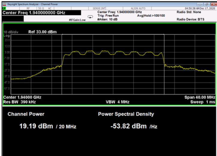
Figure 33: 16QAM 20MHz B.W.; 1940.0MHz, 15kHz
