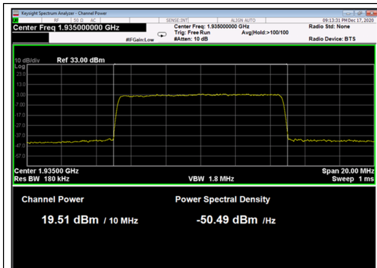
Figure 81: 64QAM 10MHz B.W.; 1935.00MHz, 15kHz
