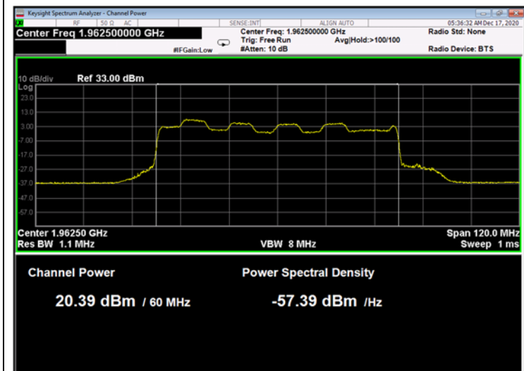
Figure 71: 16QAM 60MHz B.W.; 1962.5MHz, 30kHz
