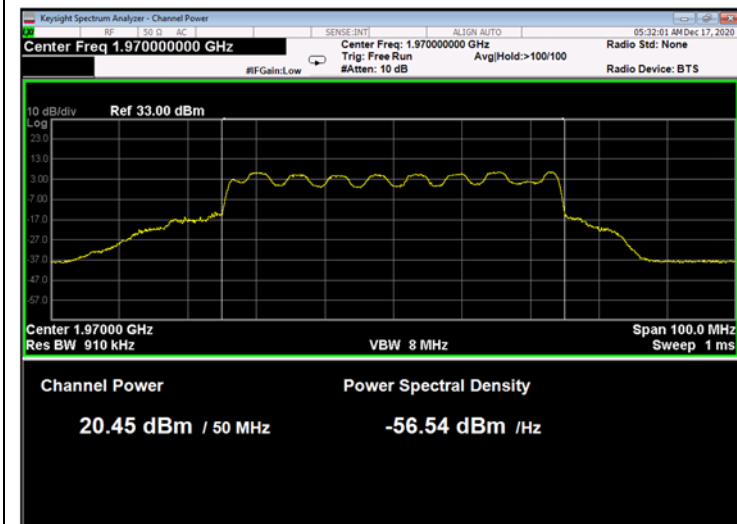
Figure 67: 16QAM 50MHz B.W.; 1970.0MHz, 30kHz
