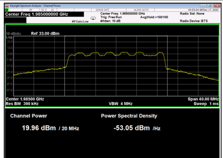
Figure 40: 16QAM 20MHz B.W.; 1985.0MHz, 30kHz
