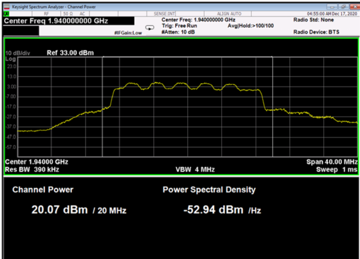
Figure 35: 16QAM 20MHz B.W.; 1940.0MHz, 60kHz
