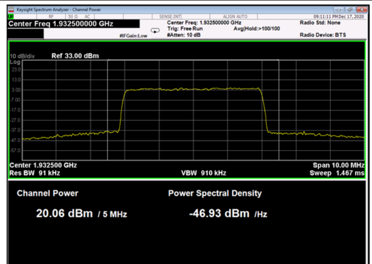
Figure 76: 64QAM 5MHz B.W.; 1932.5MHz, 30kHz
