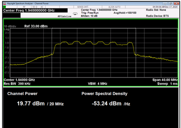
Figure 34: 16QAM 20MHz B.W.; 1940.0MHz, 30kHz
