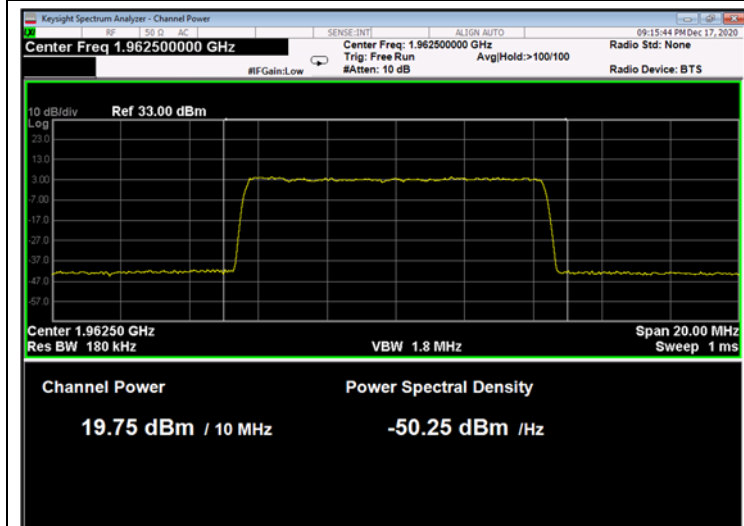
Figure 85: 64QAM 10MHz B.W.; 1962.5MHz, 30kHz
