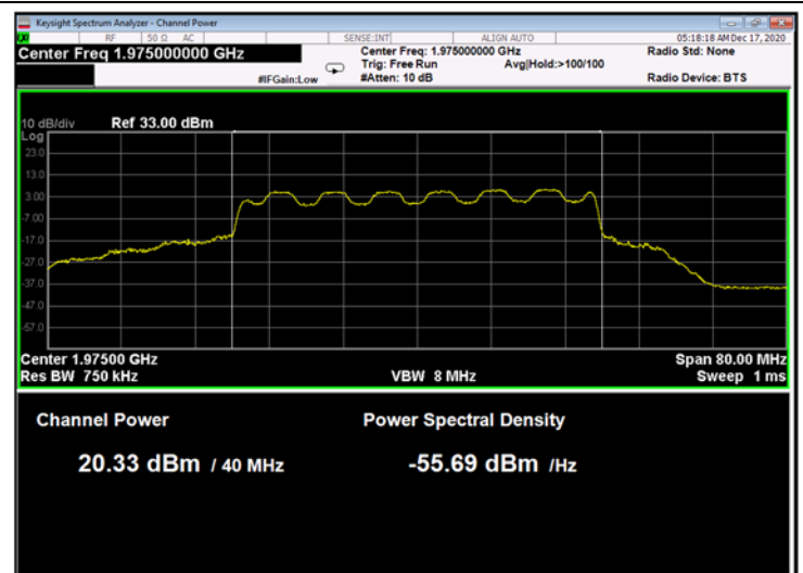
Figure 58: 16QAM 40MHz B.W.; 1975.0MHz, 30kHz
