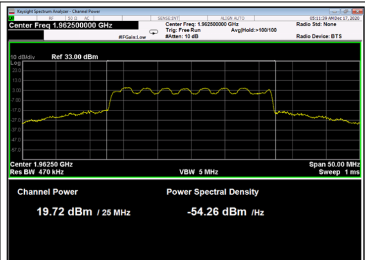
Figure 46: 16QAM 25MHz B.W.; 1962.5MHz, 30kHz
