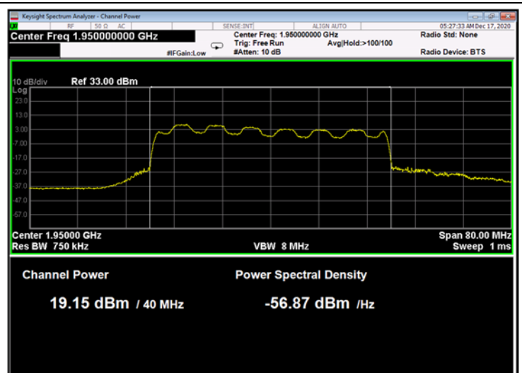
Figure 52: 16QAM 40MHz B.W.; 1950.0MHz, 30kHz
