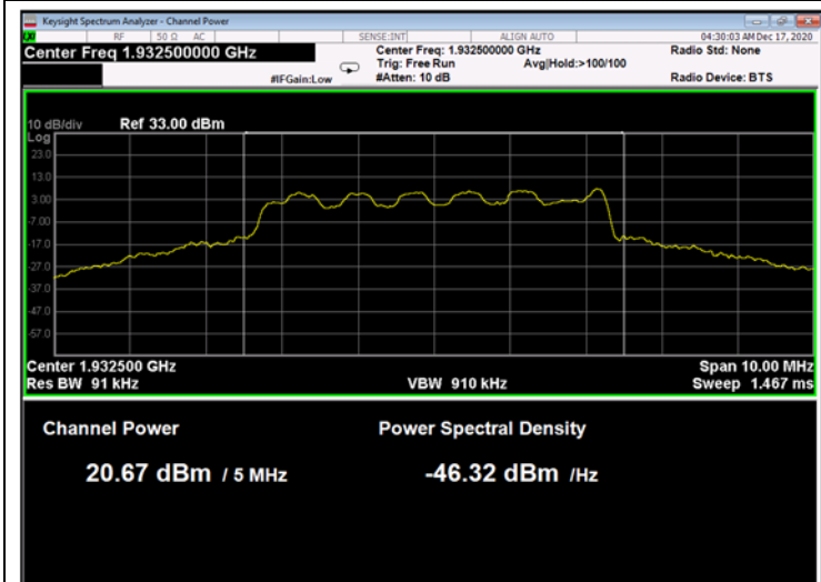
Figure 9: 16QAM 5MHz B.W.; 1932.5MHz, 15kHz
