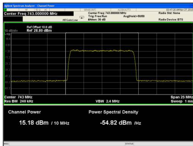
Figure 52: 64QAM 10MHz B.W.; 743.0MHz, 30kHz
