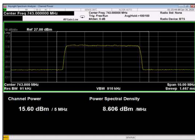
Figure 78: 256QAM 5MHz B.W.; 743.0MHz, 15kHz
