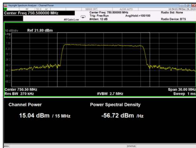
Figure 128: QPSK 15MHz B.W.; 750.5MHz, 60kHz
