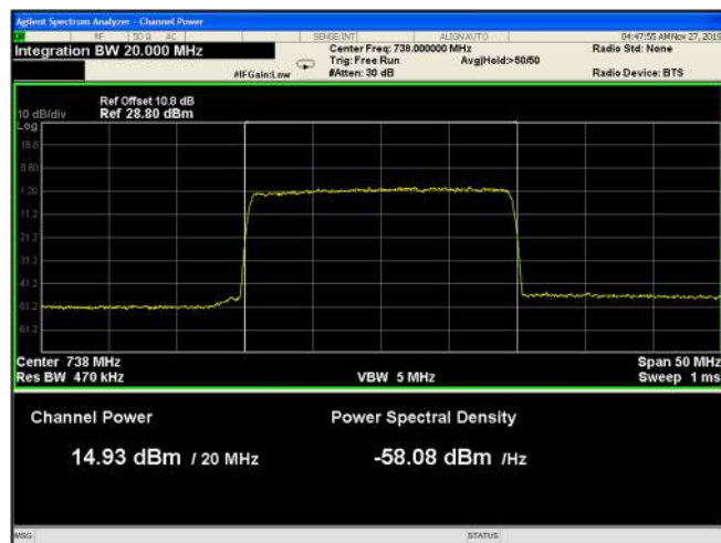
Figure 66: 64QAM 20MHz B.W.; 738.0MHz, 15kHz
