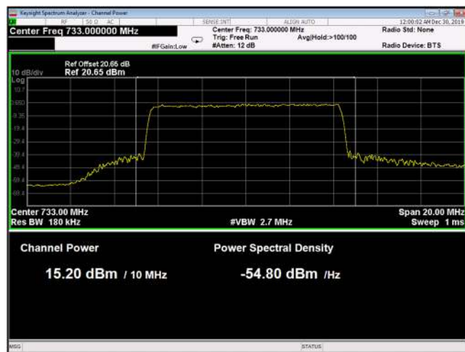
Figure 82: 256QAM 10MHz B.W.; 733.0MHz, 30kHz
