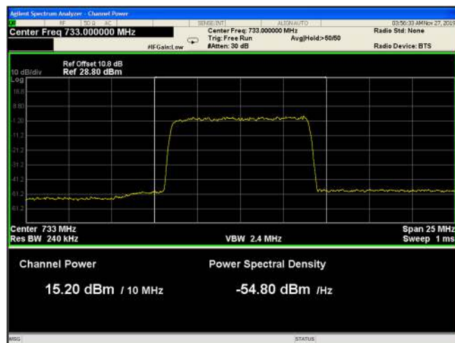
Figure 50: 64QAM 10MHz B.W.; 733.0MHz, 60kHz
