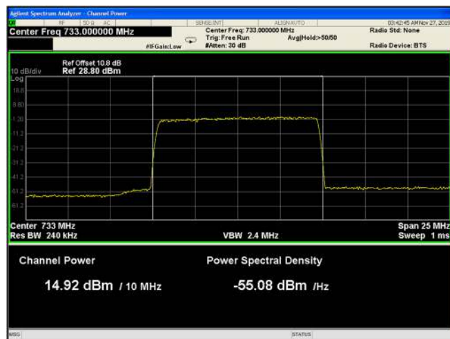
Figure 48: 64QAM 10MHz B.W.; 733.0MHz, 15kHz
