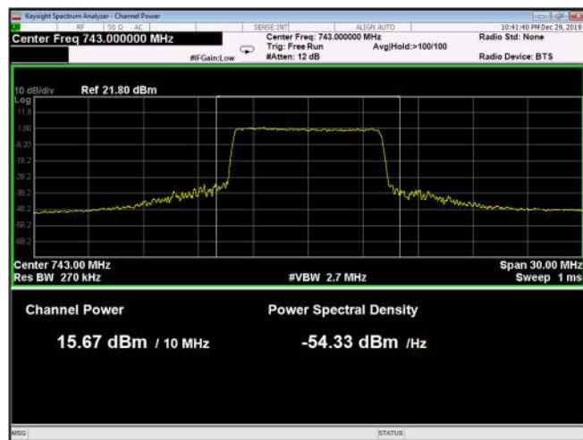
Figure 116: QPSK 10MHz B.W.; 743.0MHz, 60kHz
