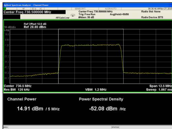
Figure 42: 64QAM 5MHz B.W.; 730.5MHz, 15kHz
