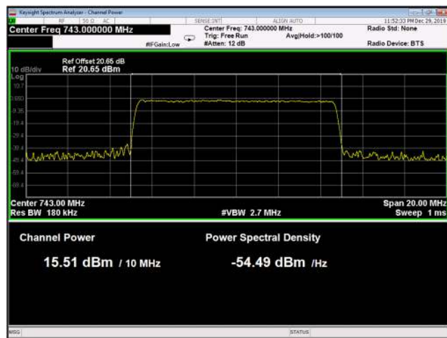
Figure 84: 256QAM 10MHz B.W.; 743.0MHz, 15kHz
