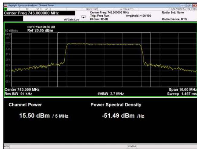
Figure 108: QPSK 5MHz B.W.; 743.0MHz, 30kHz
