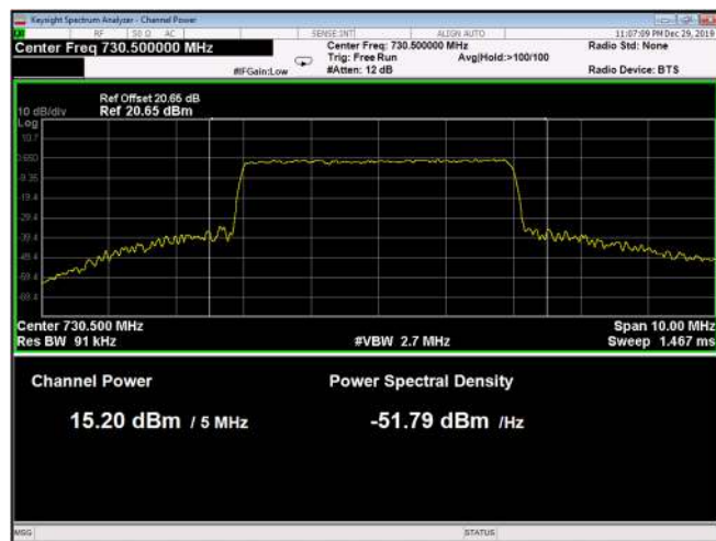
Figure 106: QPSK 5MHz B.W.; 730.5MHz, 30kHz
