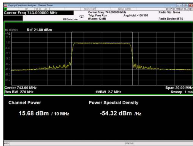
Figure 114: QPSK 10MHz B.W.; 743.0MHz, 15kHz
