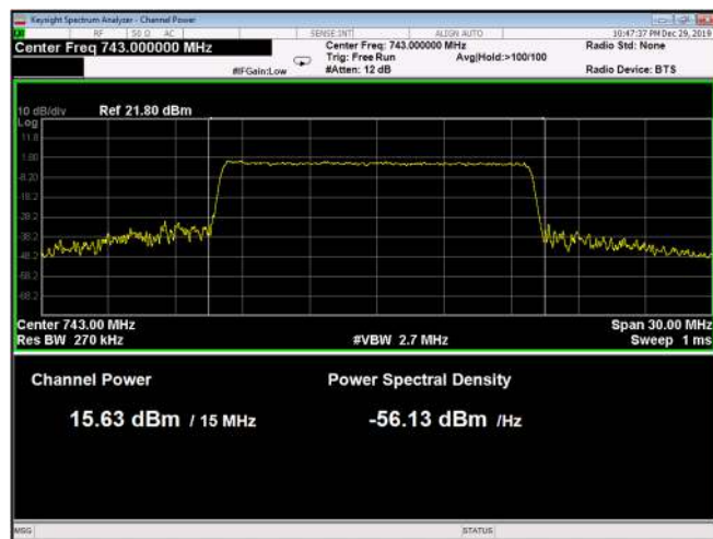
Figure 124: QPSK 15MHz B.W.; 743.0MHz, 30kHz
