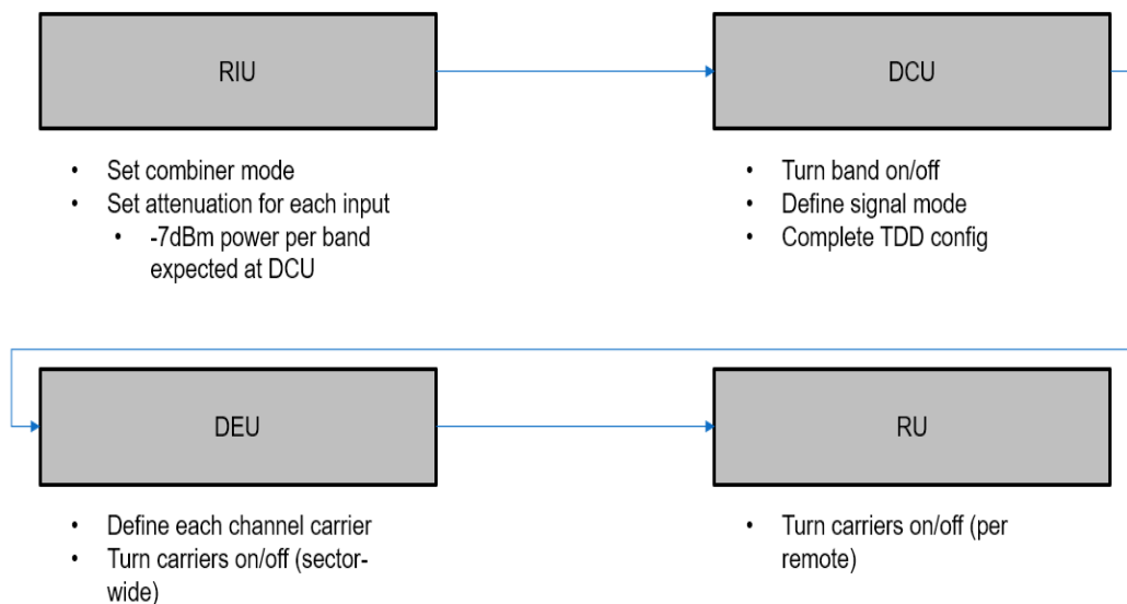
Figure 103. webGUI Workflow
