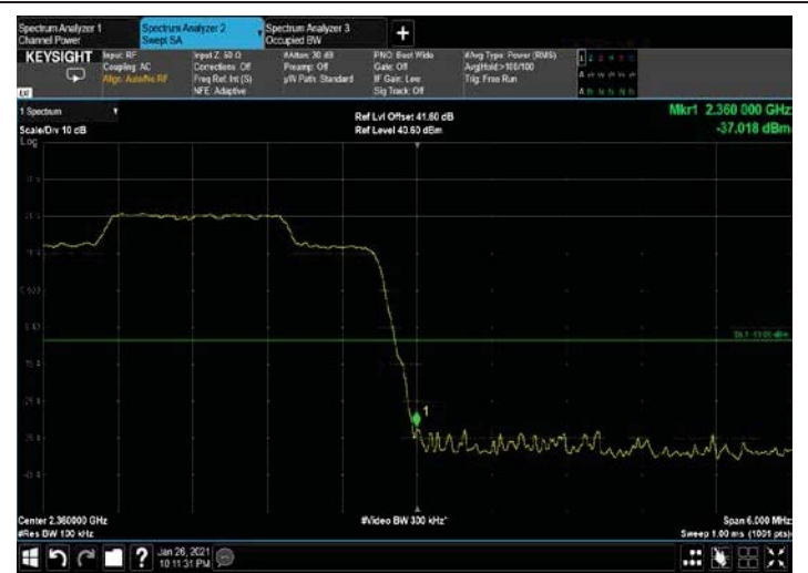
Figure 33: QPSK 10MHz B.W.; 2355MHz, 15kHz-5G Upper Edge
