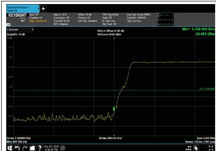
Figure 38: 64QAM 10MHz B.W.; 2355MHz-4G Lower Edge
