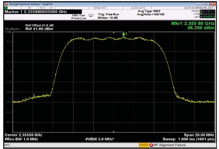
Figure 43: 16QAM 10MHz B.W; 2355MHz, 30kHz-5G
