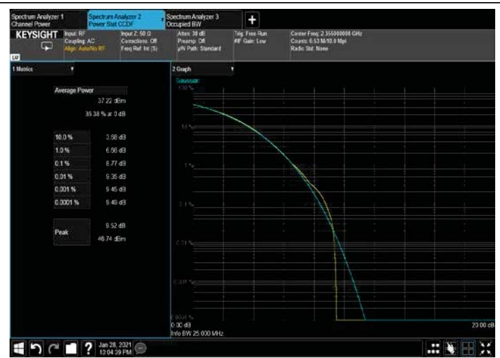
Figure 54: 16QAM 10MHz B.W; 2355MHz, 30kHz-5G
