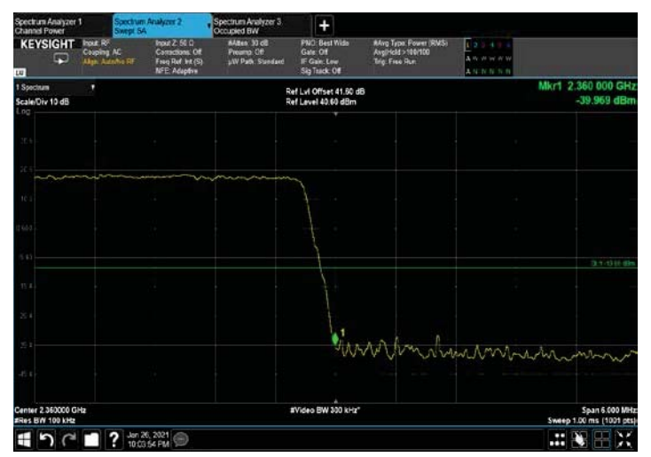
Figure 29: 256QAM 10MHz B.W.; 2355MHz, 15kHz-5G Upper Edge
