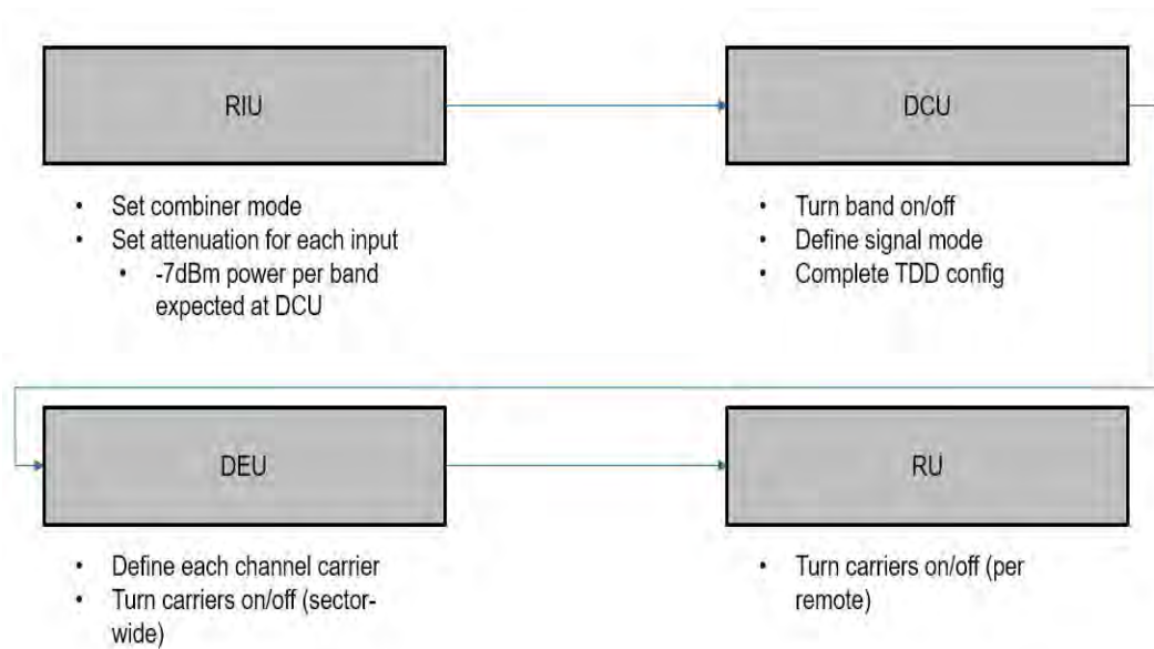
Figure 69 webGUI Workflow
