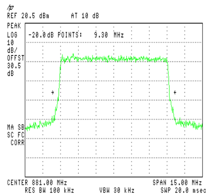
Figure 23.— Input 881 MHz.
