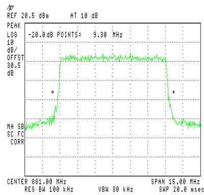
Figure 29.— Input 881 MHz.
