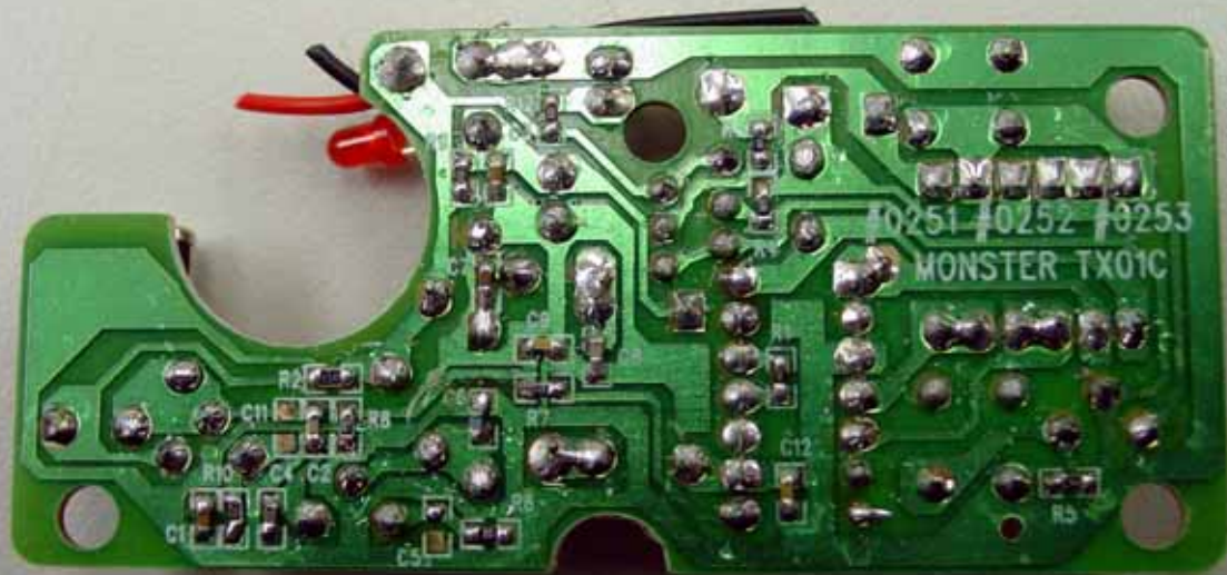
49 MHz - TXPCB
