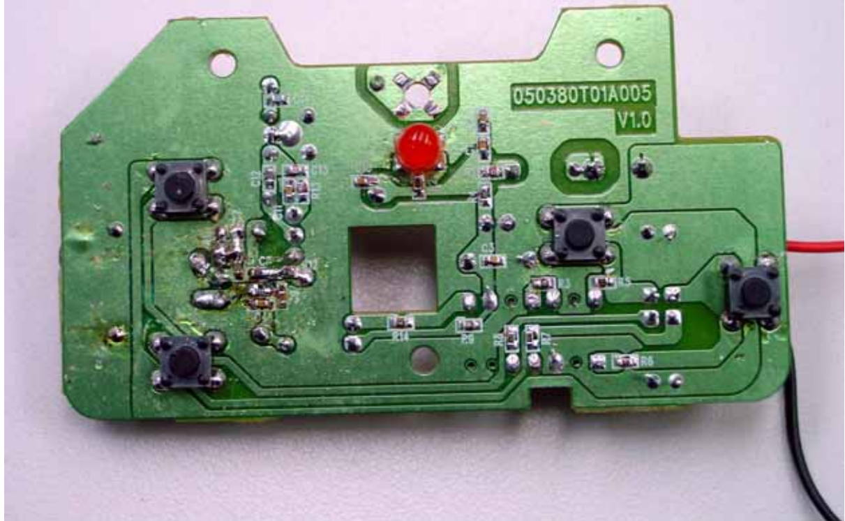
27MHz - TXPCB
