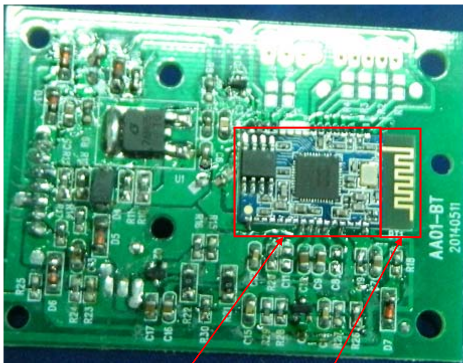
Bluetooth Module
