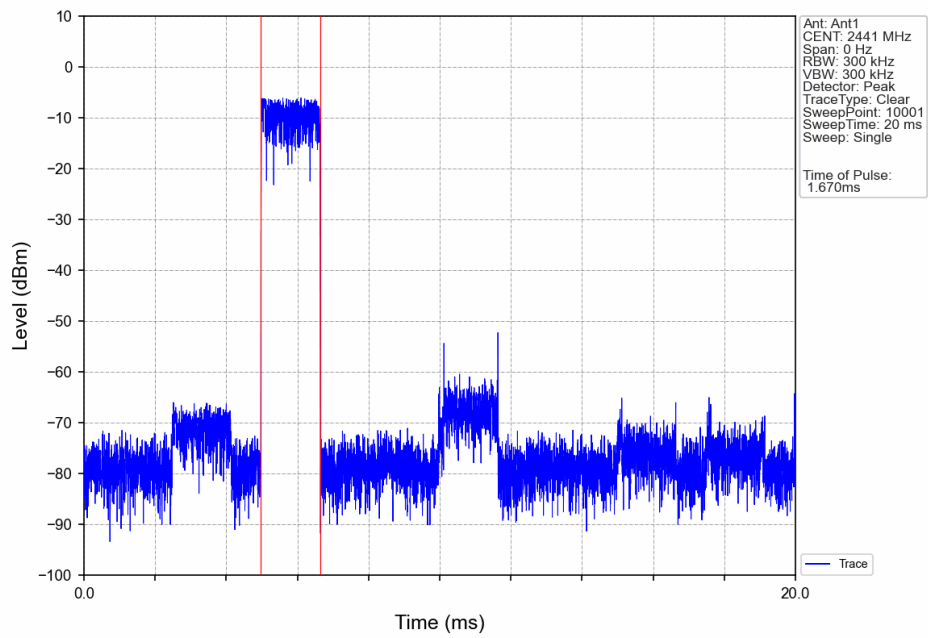
Pi/4DQPSK_2DH3_HOPP_Ant1_NTNV
