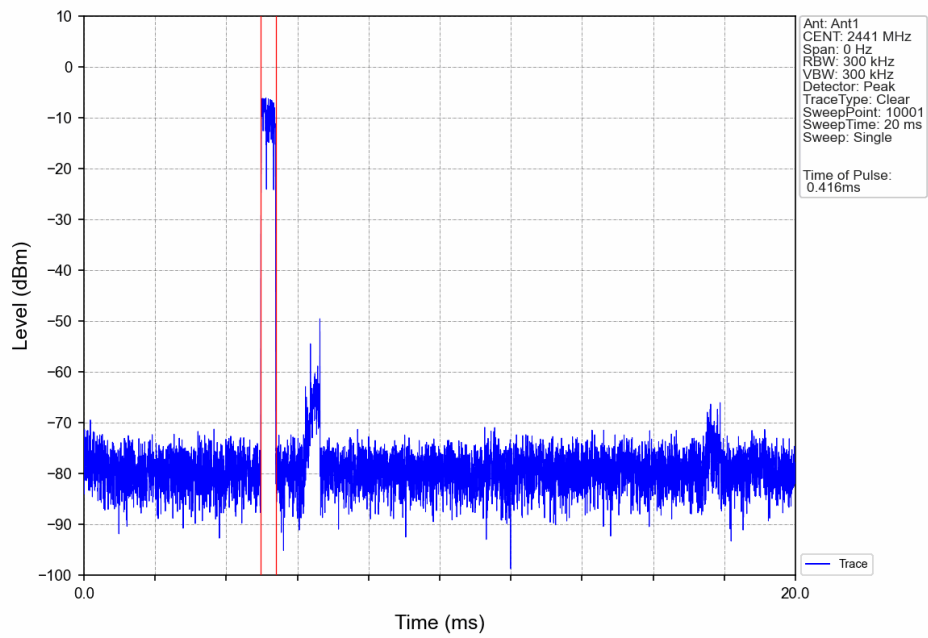
Pi/4DQPSK_2DH1_HOPP_Ant1_NTNV
