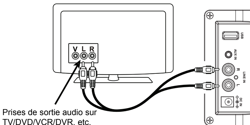
Vue arrière de l'appareil
