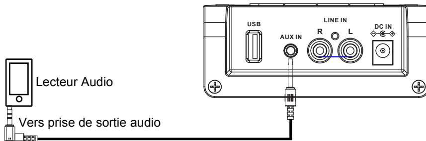
Vue arrière de l'appareil
