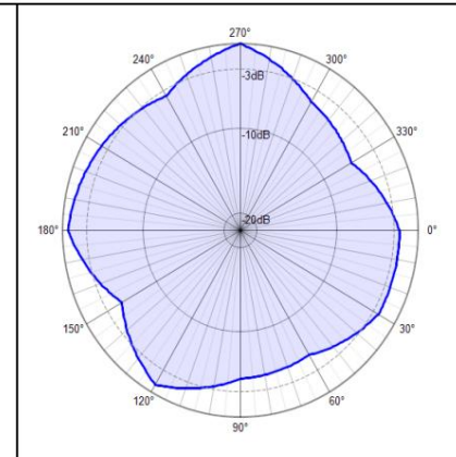
2500MHz E1
