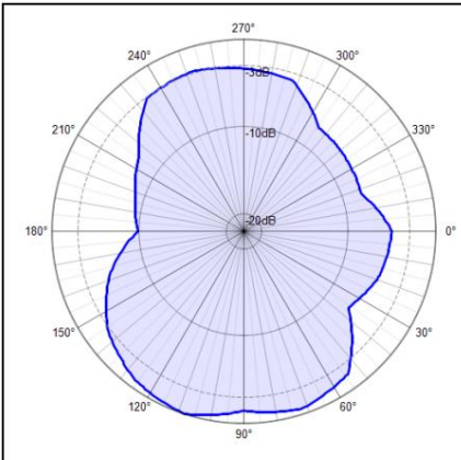
2500MHzH
