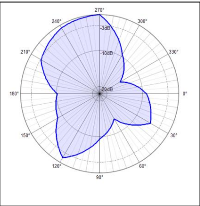
2450MHz E2
