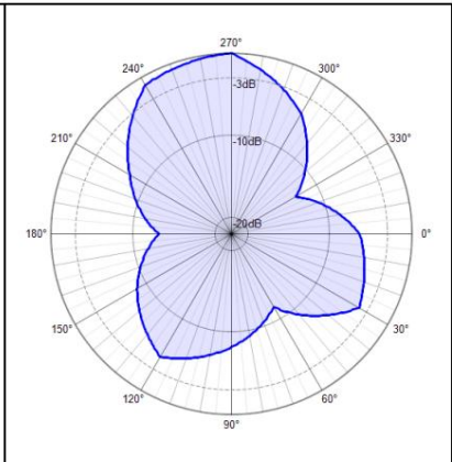
2500MHz E2
