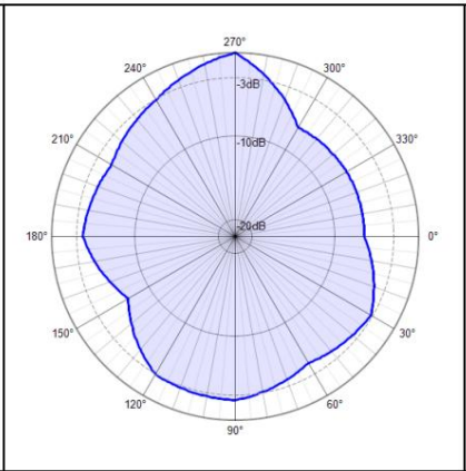
2450MHz E1
