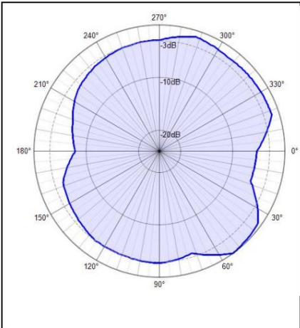
2400MHzH
