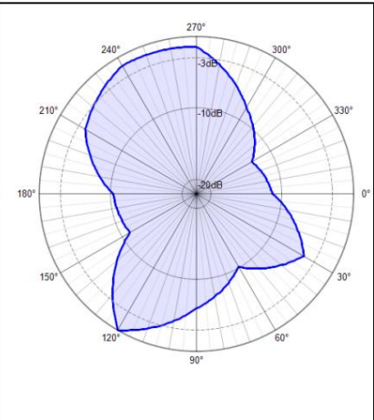
2400MHz E2
