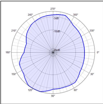
2450MHzH
