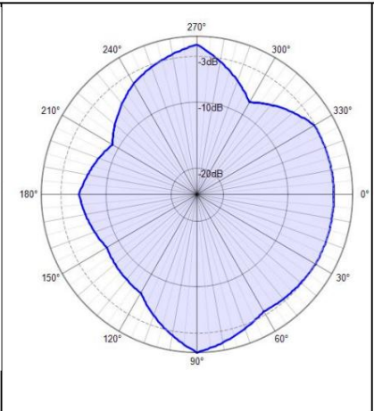
2400MHz E1
