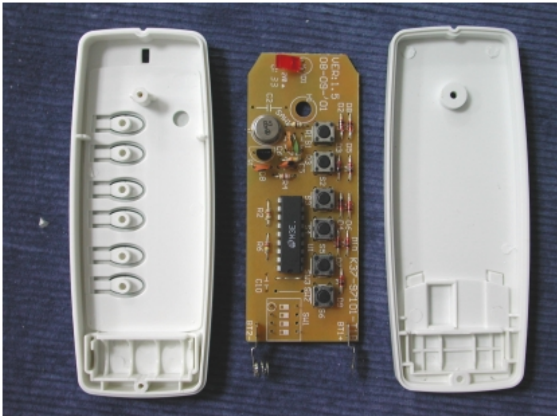
(4) EUT Photo
