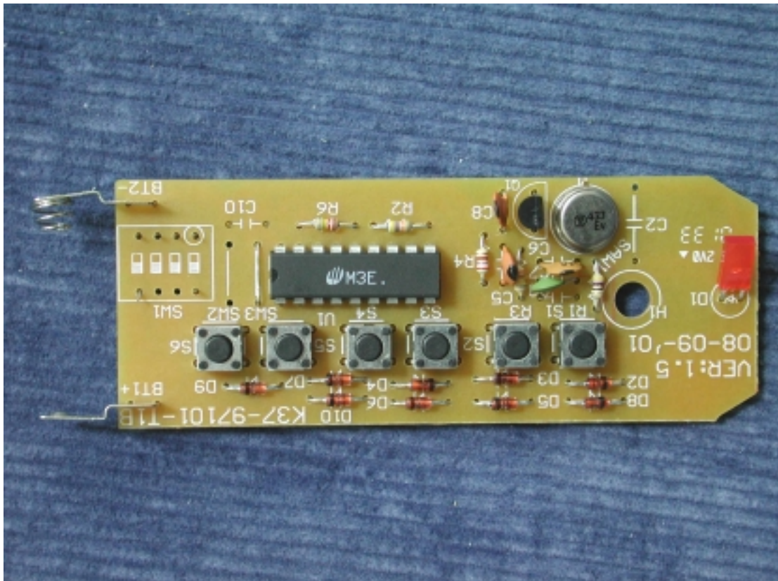
(6) EUT Photo
