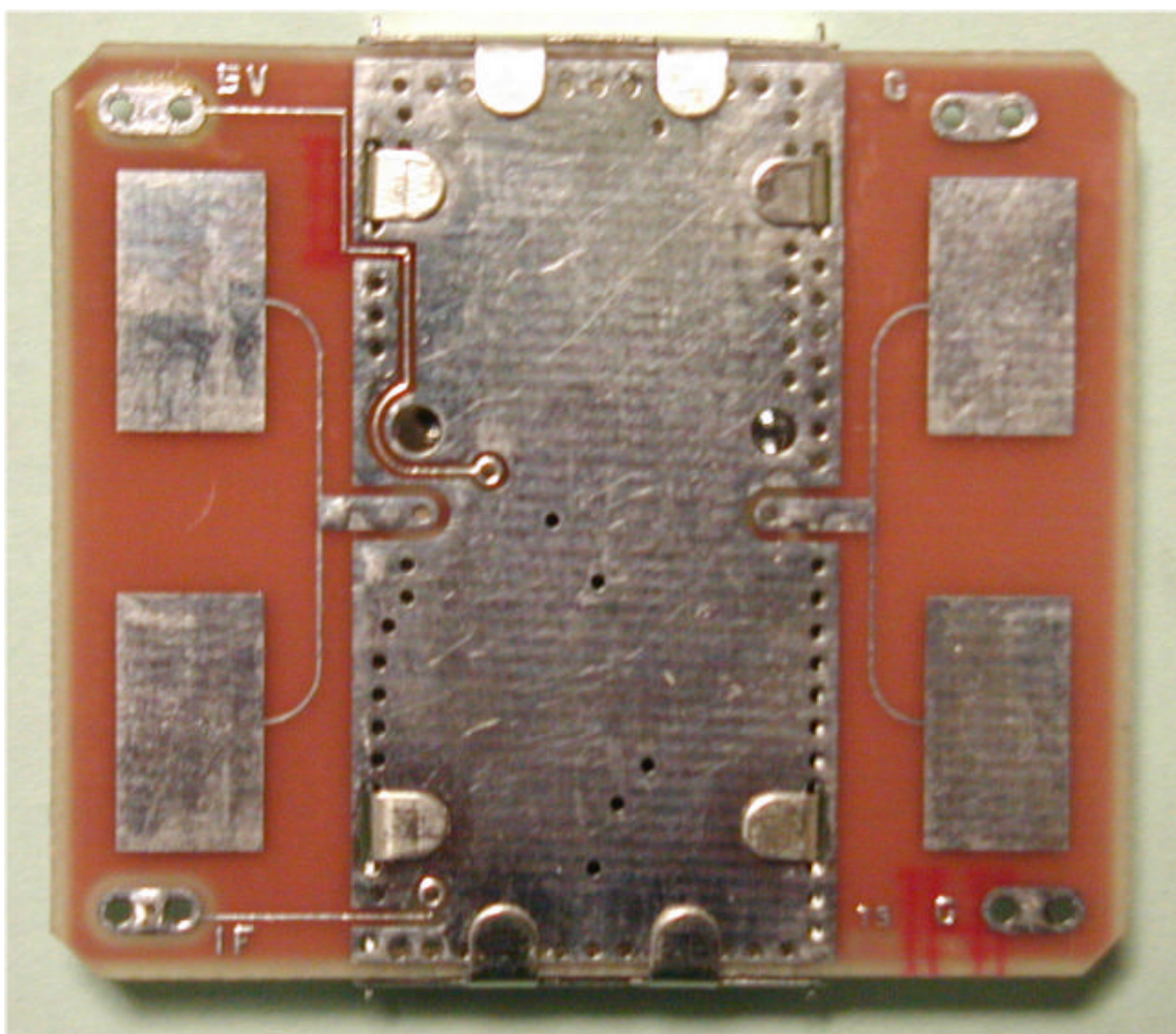
MODULE REAR
