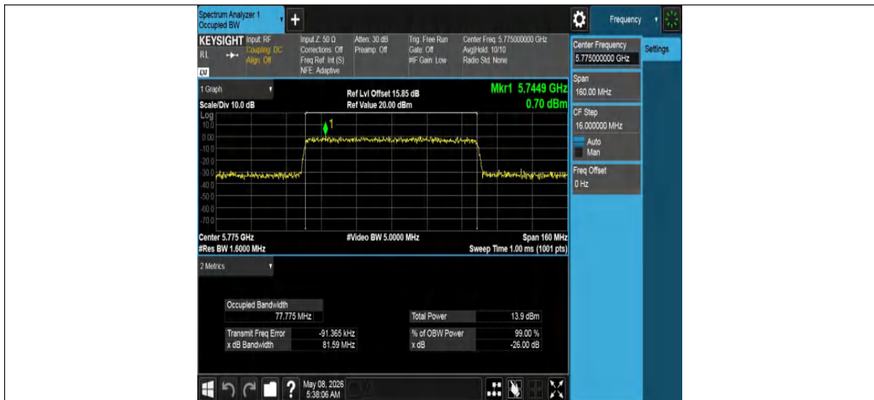
11AX80MIMO_Ant2_5775
