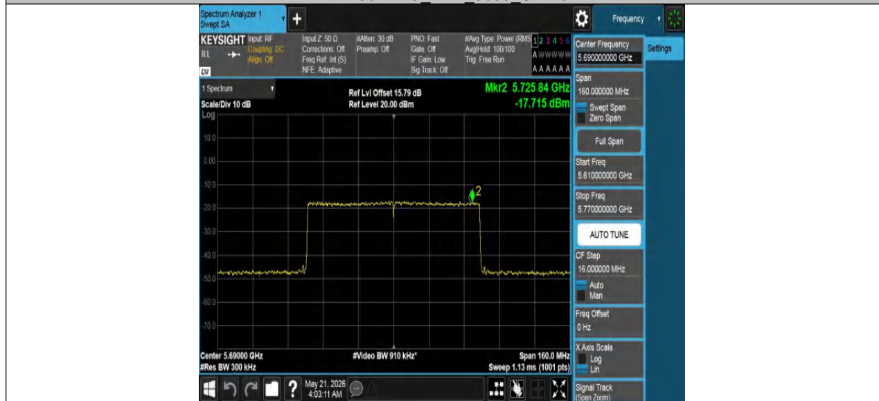
11AX80MIMO_Ant2_5690_UNII-3
