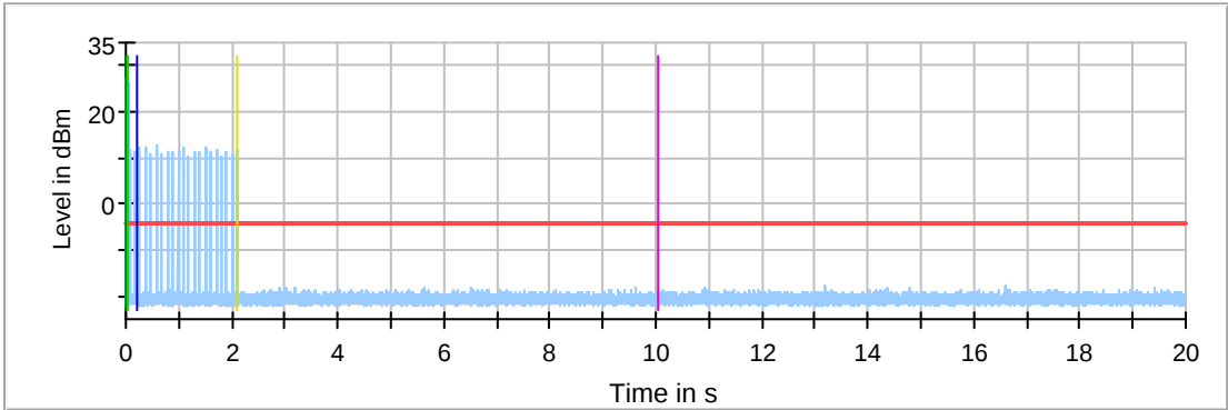
802.11n HT40 5270MHz
