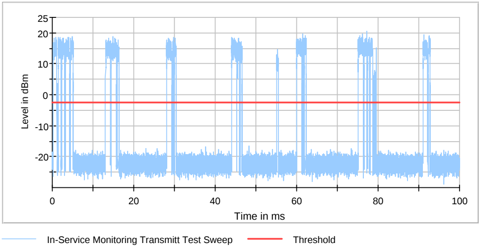
802.11n HT40 5270MHz
