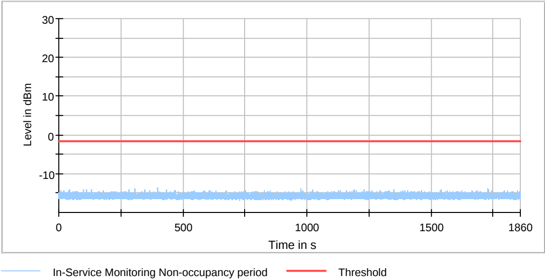
802.11n HT40 5670MHz
