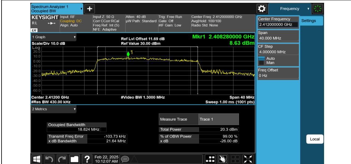
11AX20MIMO-Ant2-2412
