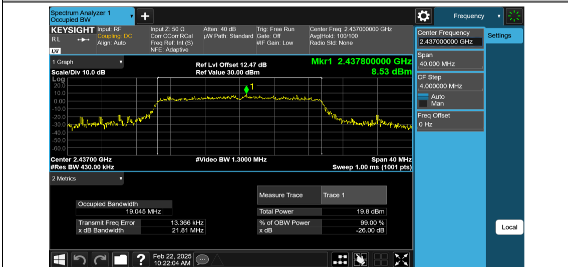
11AX20MIMO-Ant1-2437
