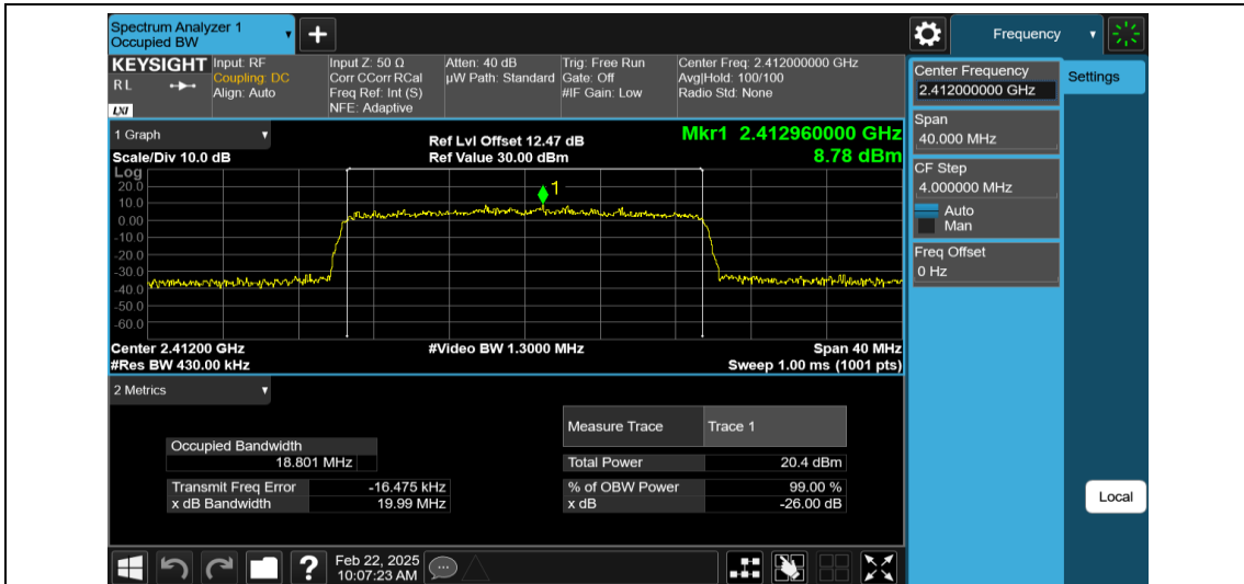
11AX20MIMO-Ant1-2412
