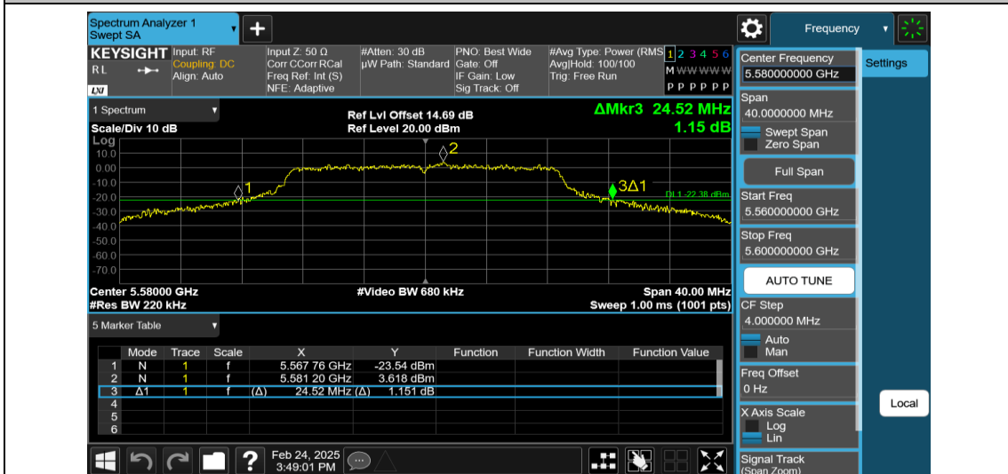
11N20MIMO-Ant1-5580
