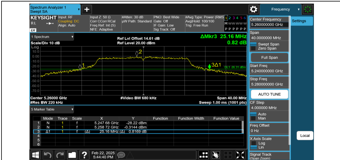
11N20MIMO-Ant1-5260
