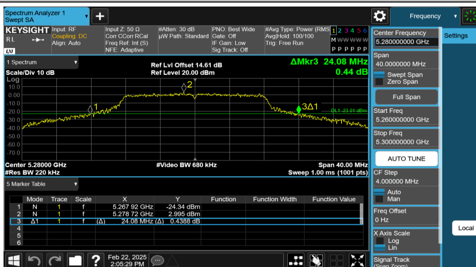
11A-Ant1-5280
