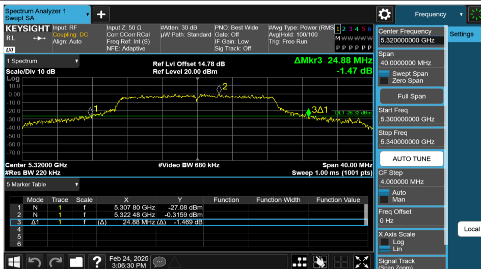
11N20MIMO-Ant1-5320
