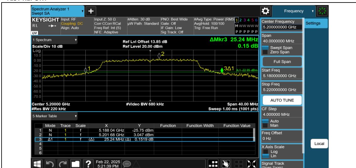
11N20MIMO-Ant2-5200
