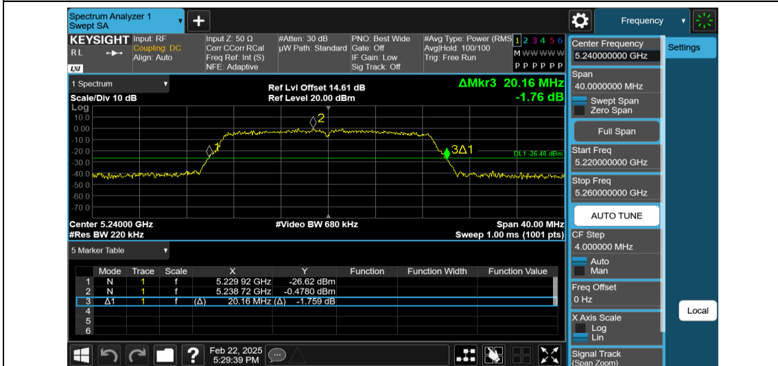
11N20MIMO-Ant1-5240
