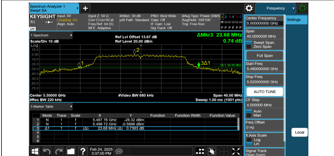
11N20MIMO-Ant2-5500
