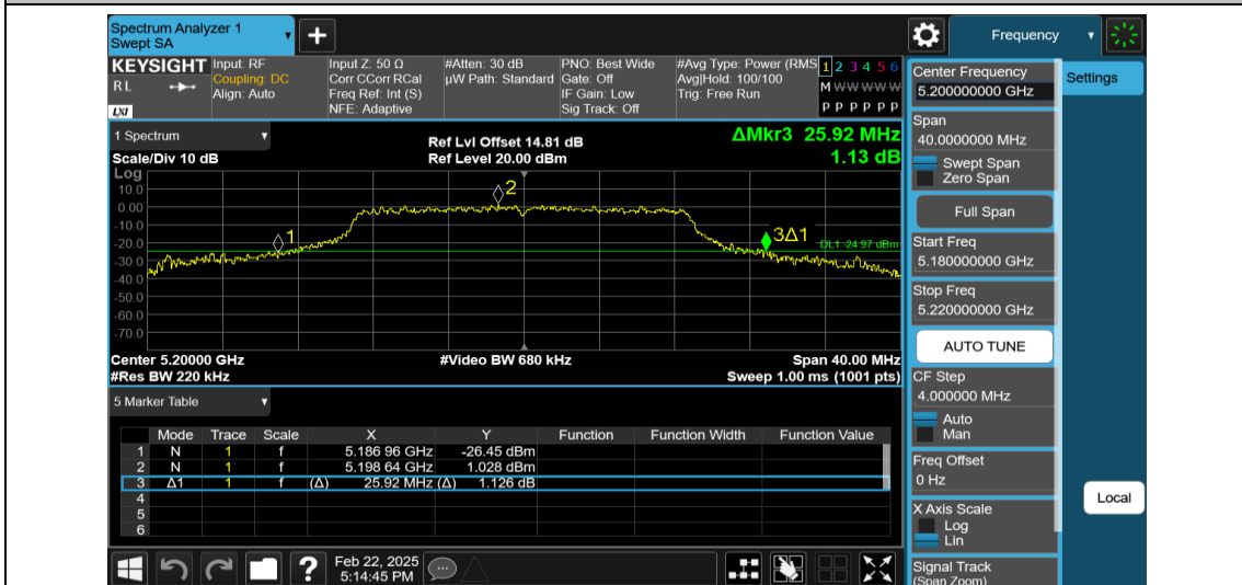
11N20MIMO-Ant1-5200
