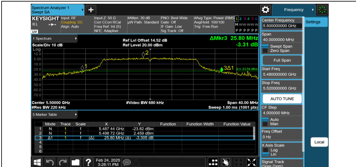
11N20MIMO-Ant1-5500
