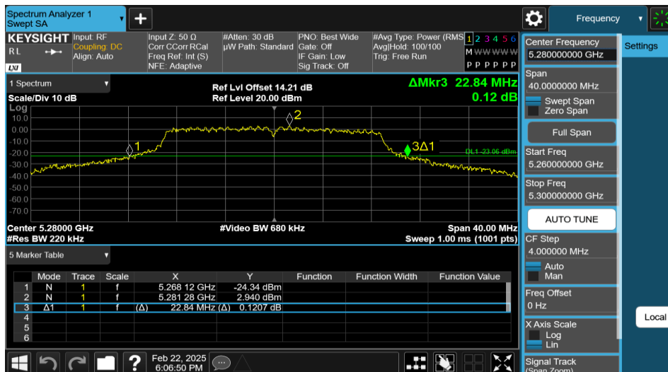
11N20MIMO-Ant2-5280
