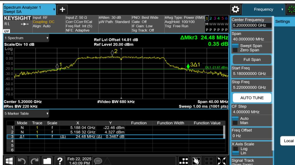
11A-Ant1-5200
