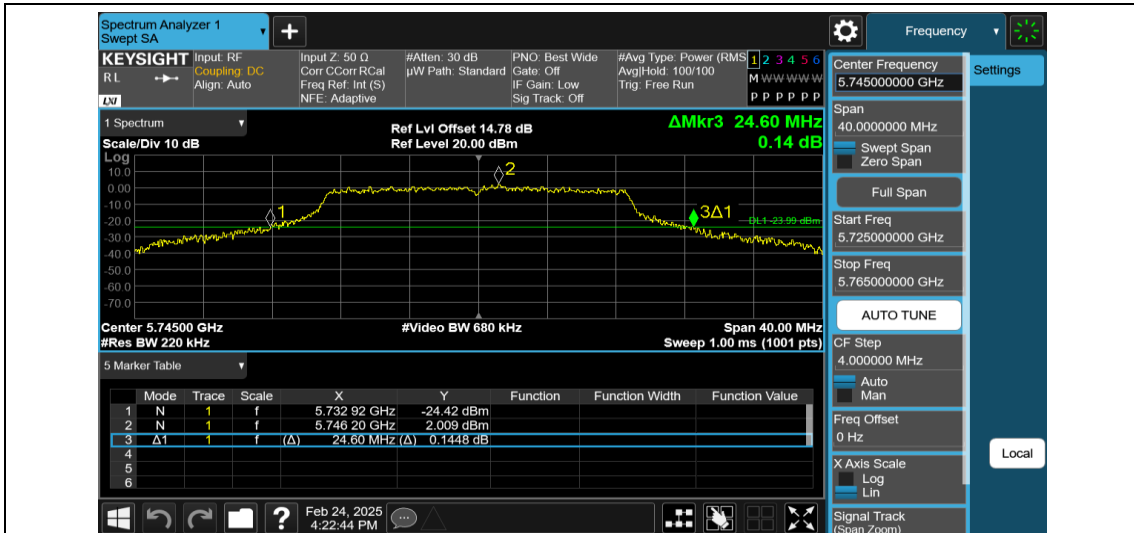
11N20MIMO-Ant1-5745
