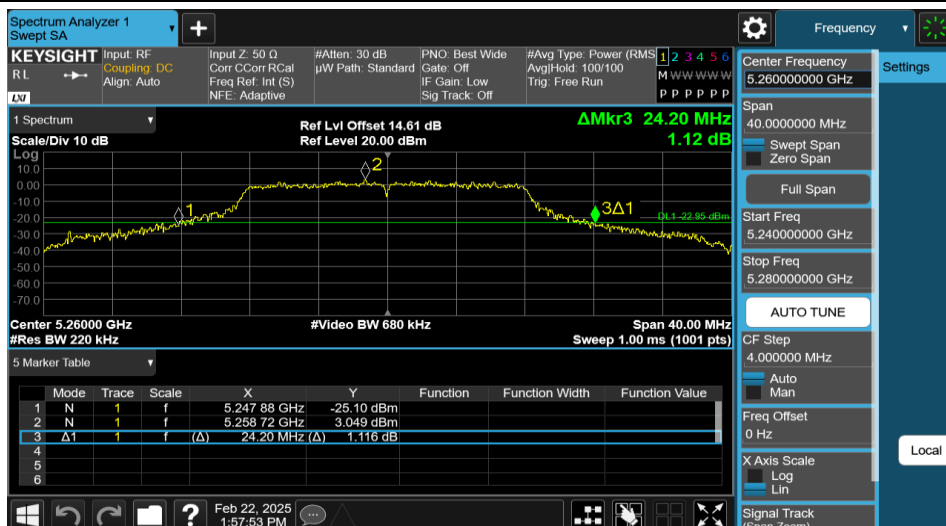
11A-Ant1-5260
