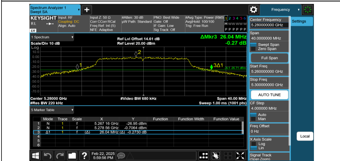
11N20MIMO-Ant1-5280
