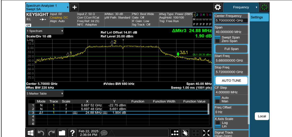
11A-Ant1-5700
