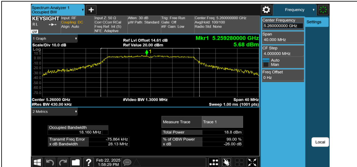
11A-Ant1-5260
