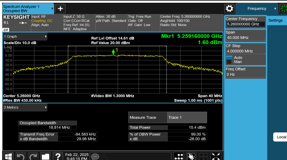
11N20MIMO-Ant1-5260
