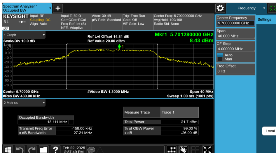
11A-Ant1-5700
