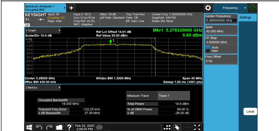
11A-Ant1-5280
