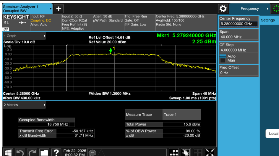
11N20MIMO-Ant1-5280
