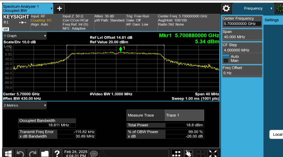
11N20MIMO-Ant1-5700
