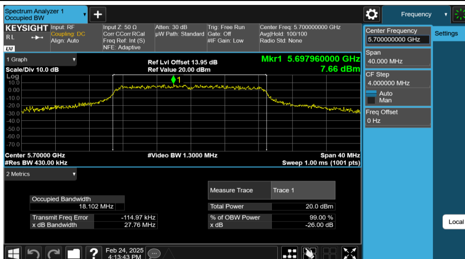
11N20MIMO-Ant2-5700
