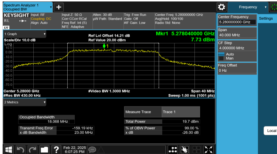
11N20MIMO-Ant2-5280
