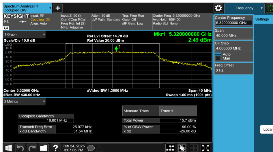
11N20MIMO-Ant1-5320
