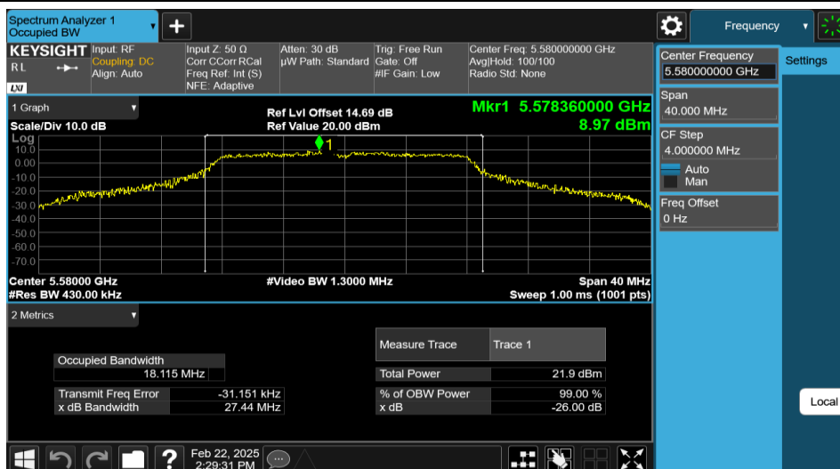
11A-Ant1-5580
