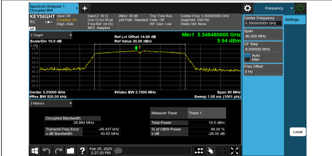
11N40MIMO-Ant1-5550
