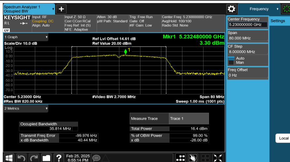
11AC40MIMO-Ant1-5230
