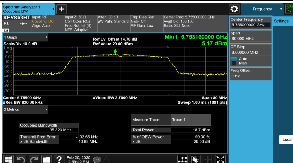
11N40MIMO-Ant1-5755
