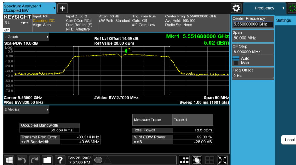
11AC40MIMO-Ant1-5550
