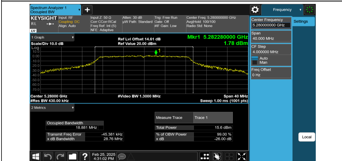
11AC20MIMO-Ant1-5280
