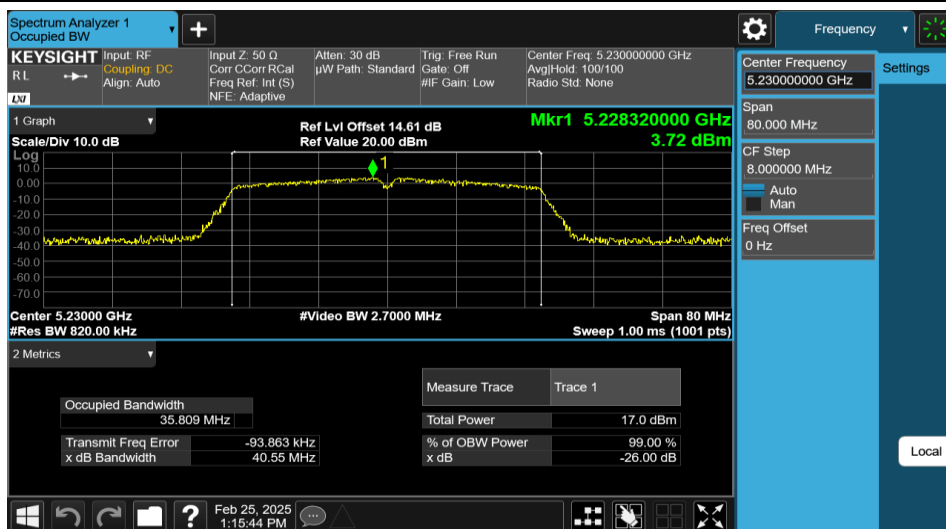
11N40MIMO-Ant1-5230
