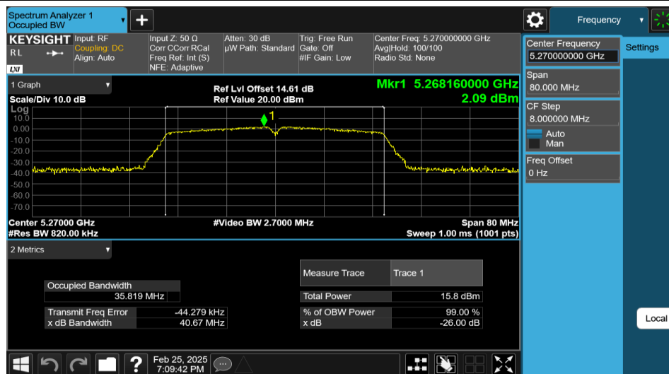
11AC40MIMO-Ant1-5270
