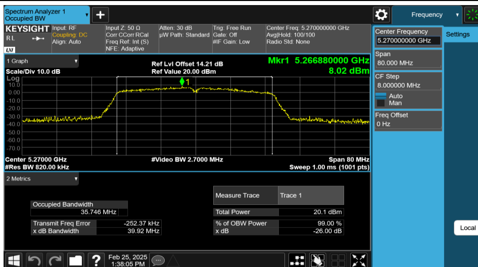
11N40MIMO-Ant2-5270
