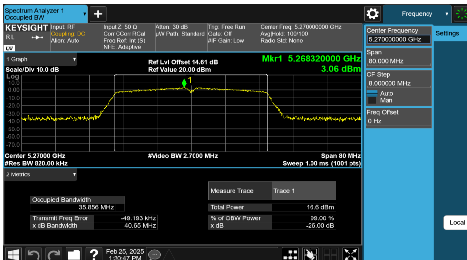
11N40MIMO-Ant1-5270
