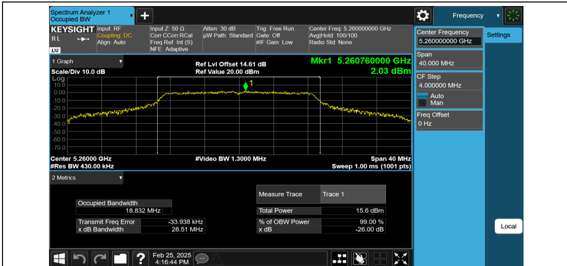
11AC20MIMO-Ant1-5260
