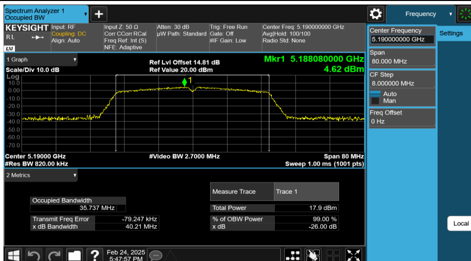
11N40MIMO-Ant1-5190
