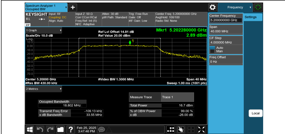
11AC20MIMO-Ant1-5200
