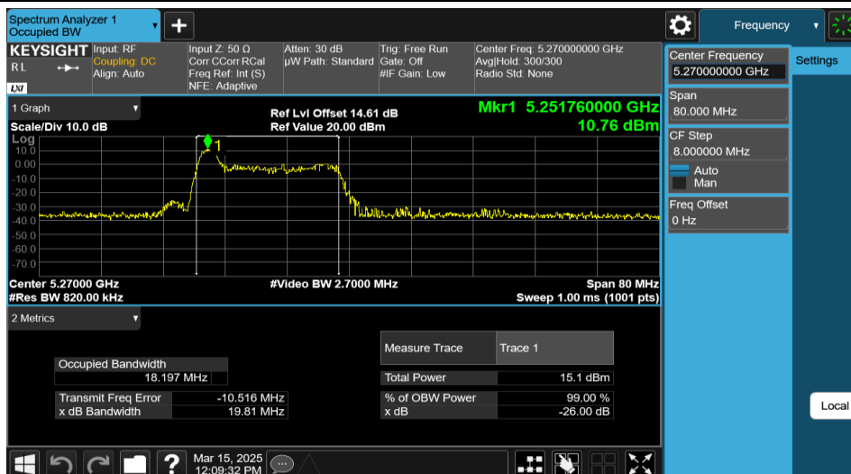
11AX40MIMO-Ant1-5270-26Tone-RU0
