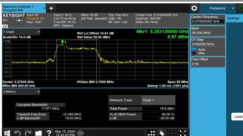
11AX40MIMO-Ant1-5270-52Tone-RU37
