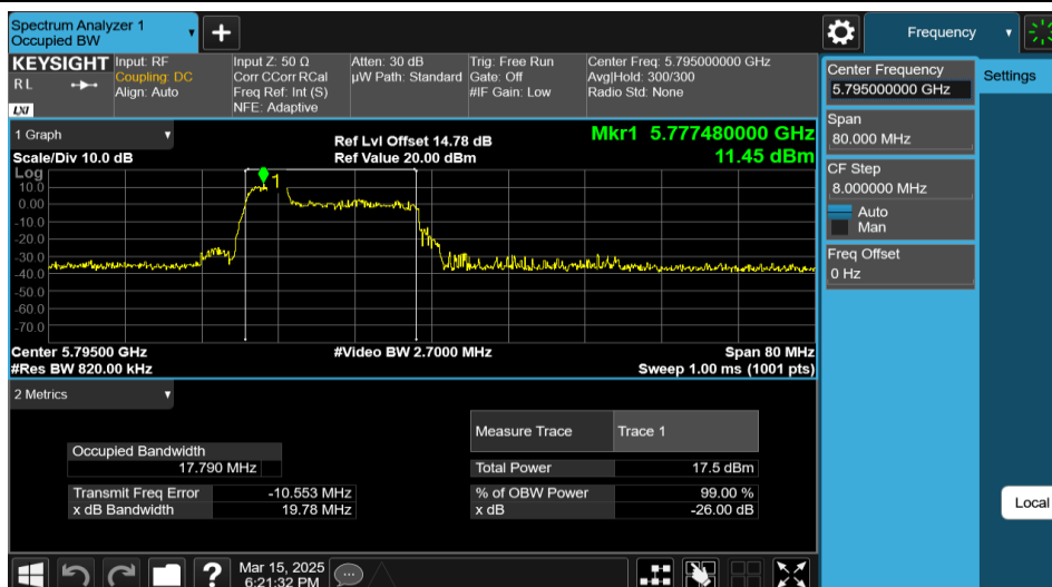
11AX40MIMO-Ant1-5795-52Tone-RU37
