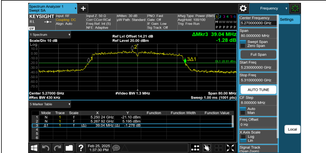
11N40MIMO-Ant2-5270
