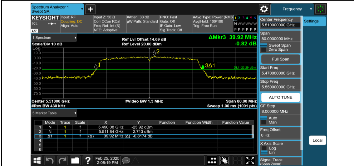
11N40MIMO-Ant1-5510
