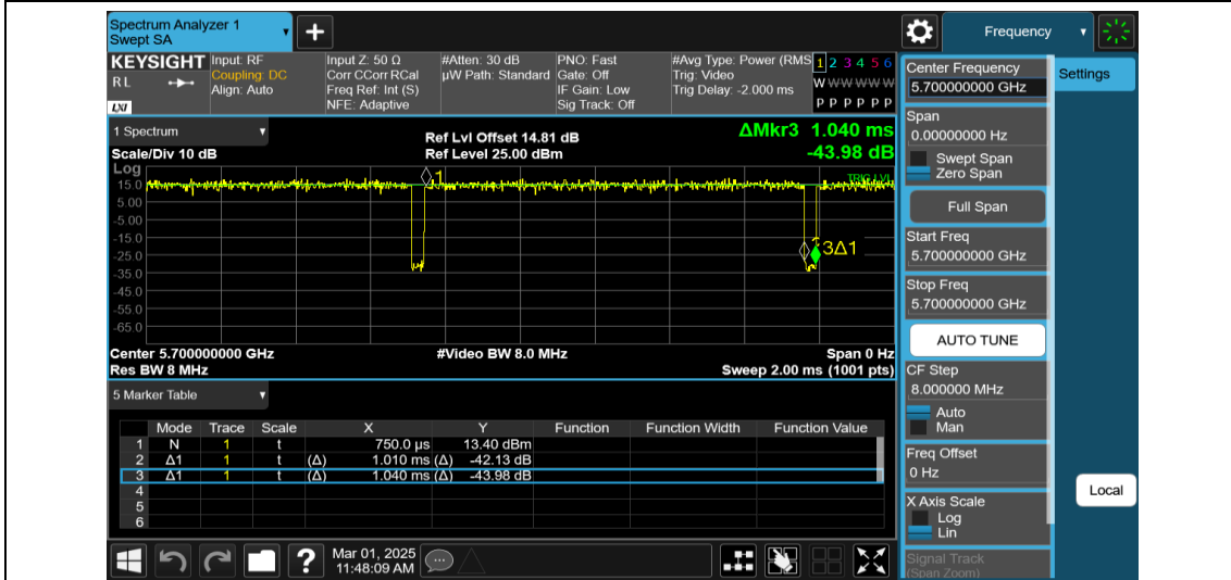
NTNV-11AX20MIMO-Ant1-5700
