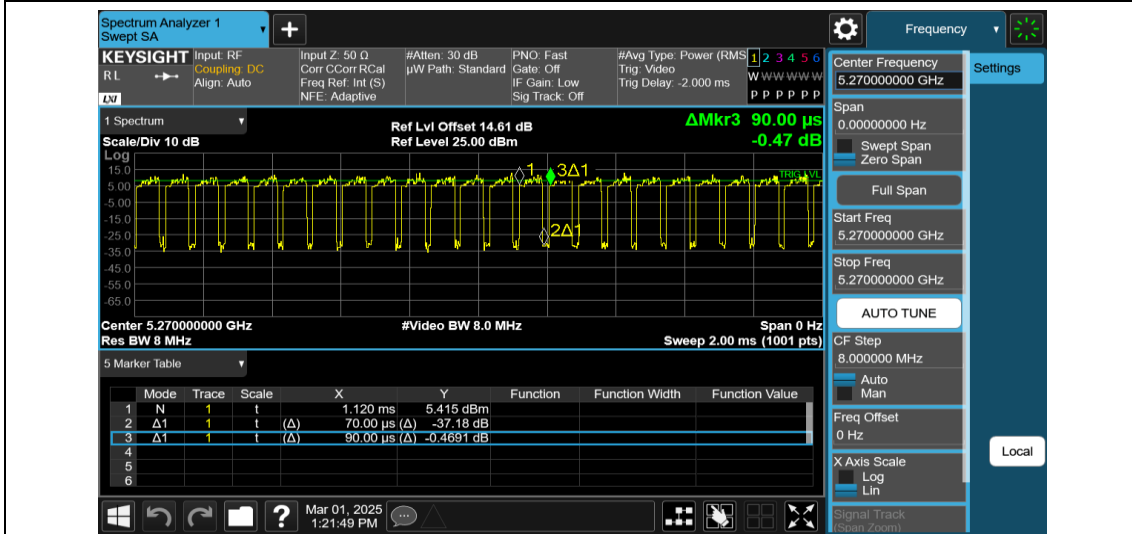
NTNV-11AX40MIMO-Ant1-5270
