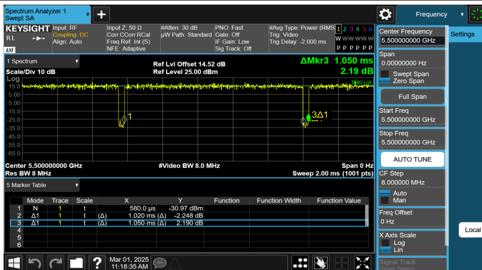
NTNV-11AX20MIMO-Ant1-5500
