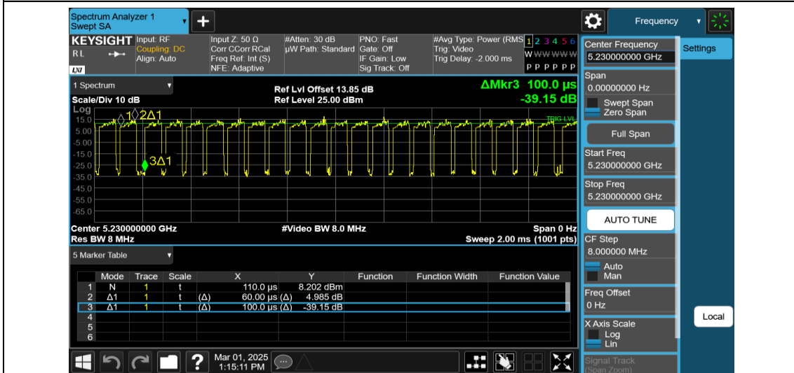
NTNV-11AX40MIMO-Ant2-5230
