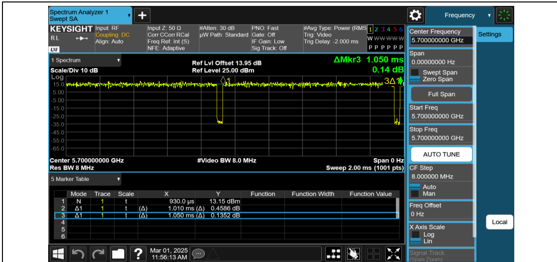
NTNV-11AX20MIMO-Ant2-5700
