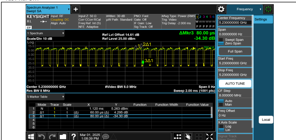
NTNV-11AX40MIMO-Ant1-5230
