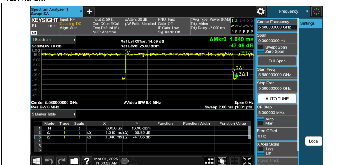
NTNV-11AX20MIMO-Ant1-5580
