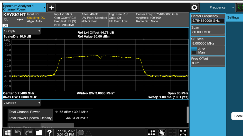
11N40MIMO-Ant1-5755-PASS
