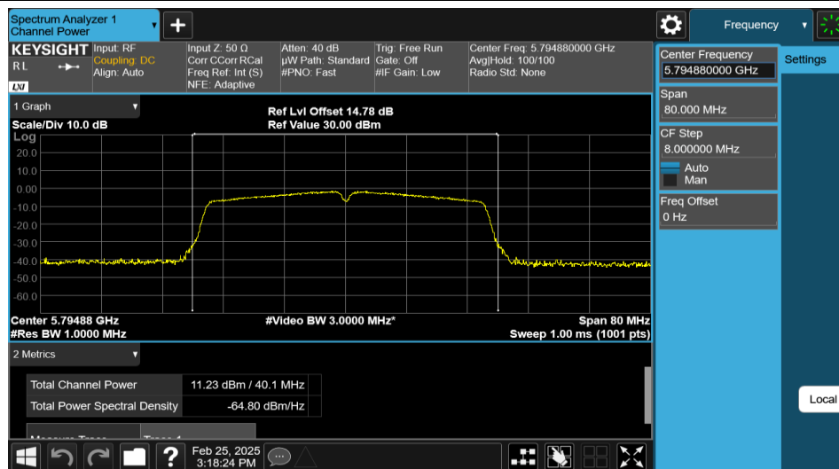
11N40MIMO-Ant1-5795-PASS
