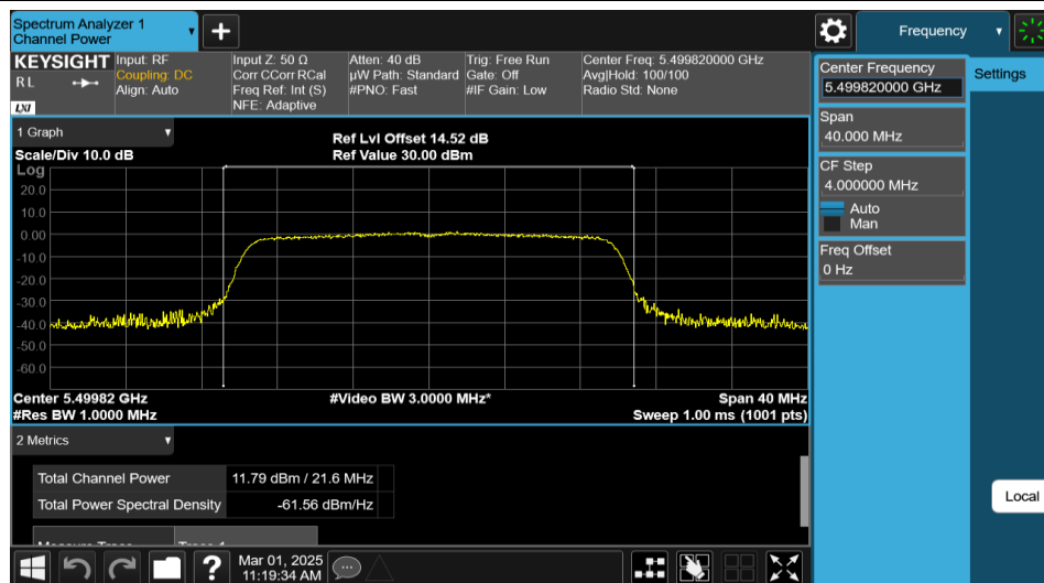
11AX20MIMO-Ant1-5500-PASS
