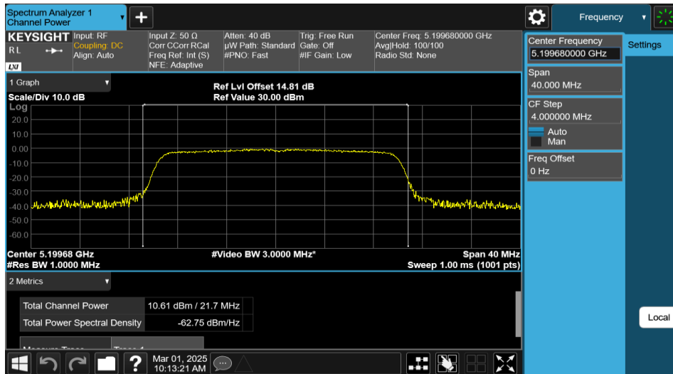
11AX20MIMO-Ant1-5200-PASS
