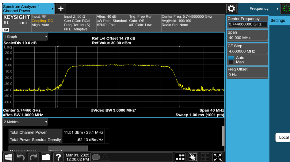
11AX20MIMO-Ant1-5745-PASS
