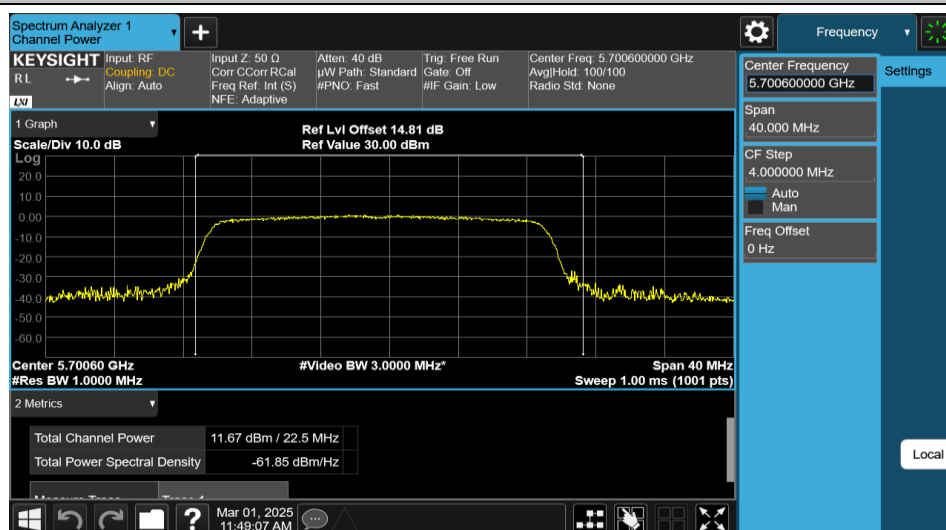
11AX20MIMO-Ant1-5700-PASS
