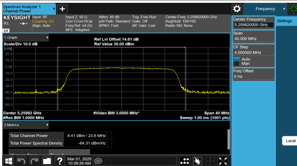
11AX20MIMO-Ant1-5260-PASS
