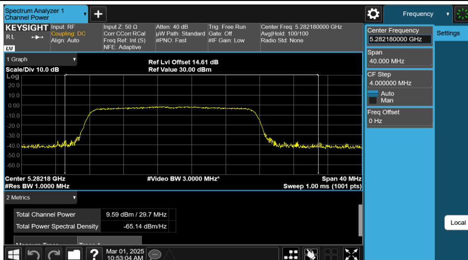
11AX20MIMO-Ant1-5280-PASS
