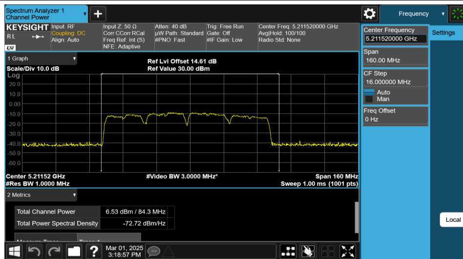
11AX80MIMO-Ant1-5210-PASS
