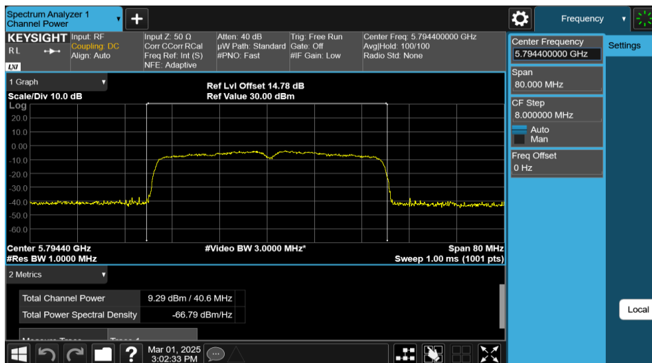
11AX40MIMO-Ant1-5795-PASS
