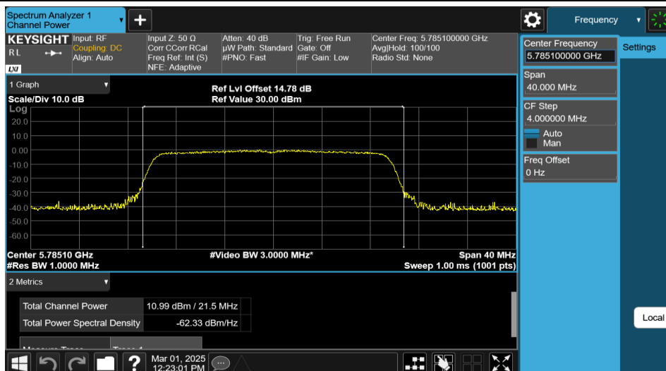
11AX20MIMO-Ant1-5785-PASS
