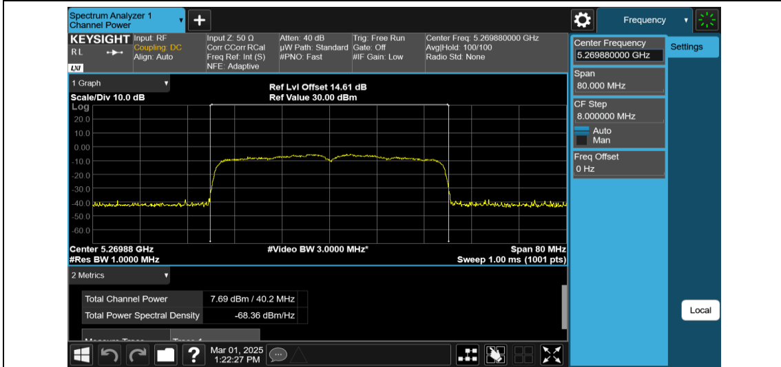
11AX40MIMO-Ant1-5270-PASS
