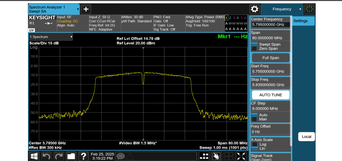
11N40MIMO-Ant1-5795-PASS
