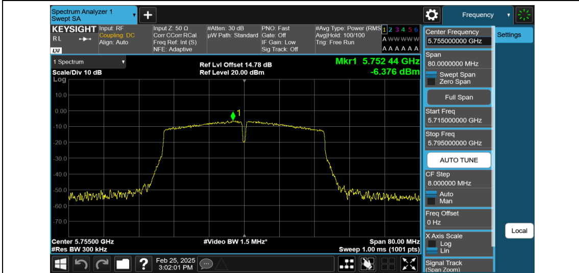
11N40MIMO-Ant1-5755-PASS
