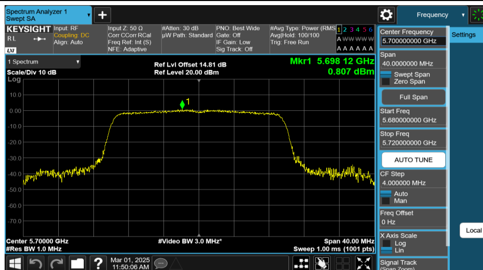
11AX20MIMO-Ant1-5700-PASS
