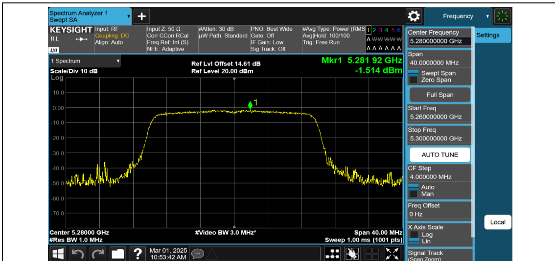
11AX20MIMO-Ant1-5280-PASS
