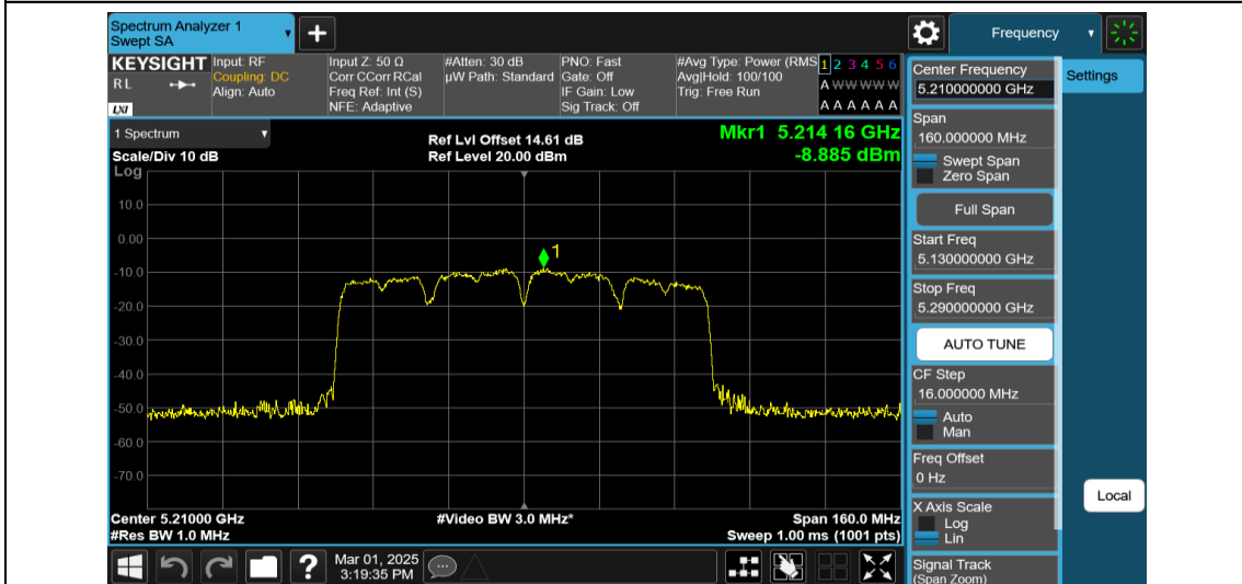
11AX80MIMO-Ant1-5210-PASS
