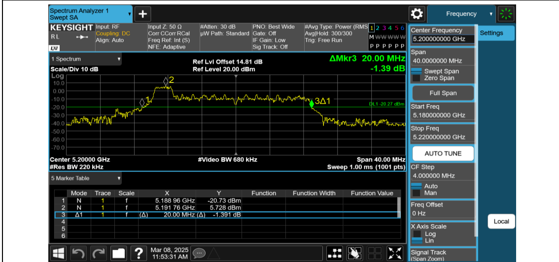
11AX20MIMO-Ant1-5200-26Tone-RU0
