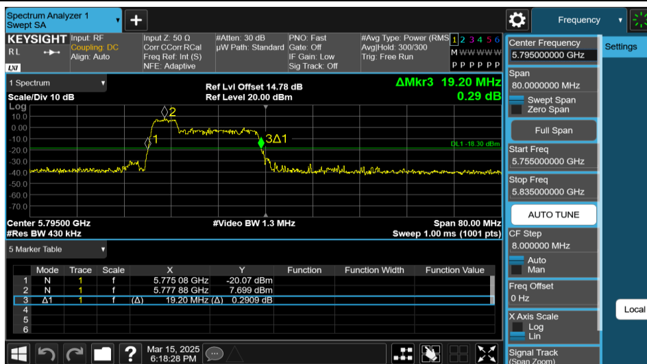
11AX40MIMO-Ant1-5795-52Tone-RU37
