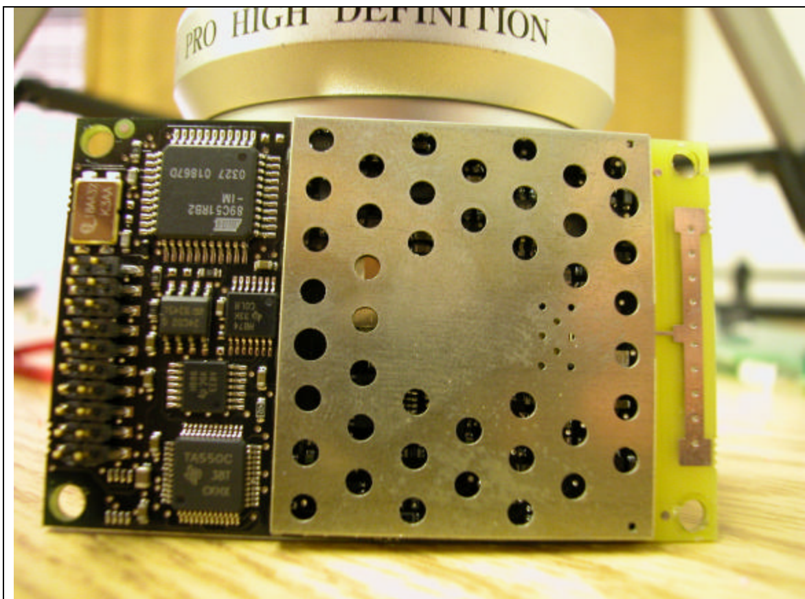
2.4GHz RF Module Top
